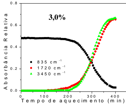
Figura 29. Cinética de termo-oxidação a 140°C do poli(1,4- cis -isopreno) na presença de 3,0% do MAT 2.
