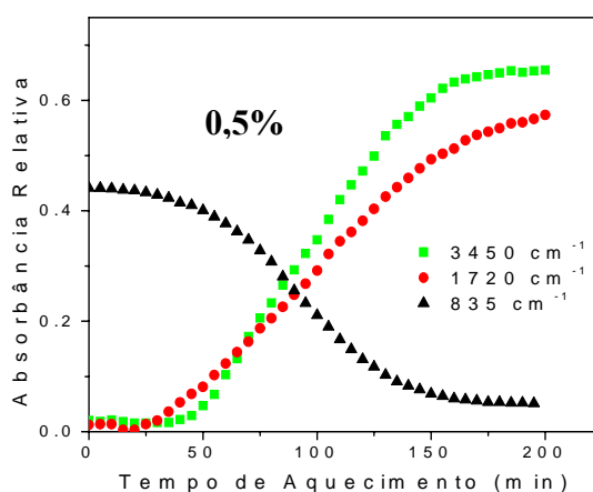
Figura 17. Cinética de termo-oxidação a 140 °C do poli(1,4- cis -isopreno) sintético na presença de 0,5% do MAT 1.
