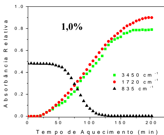
Figura 18. Cinética de termo-oxidação a 140 °C do poli(1,4- cis -isopreno) sintético na presença de 1,0% do MAT 1.
