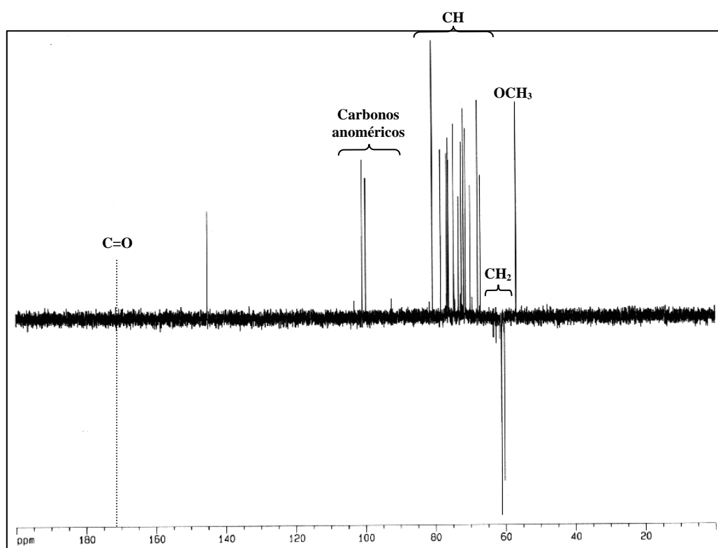
Figura 55. Espectro DEPT do Extrato de BN da mangabeira.
