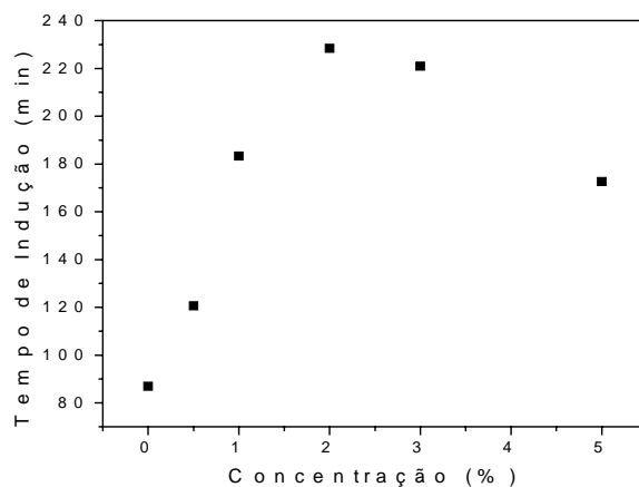
Figura 31. Efeito da concentração do MAT 2 sobre o tempo de indução da degradação termo-oxidativa do PIS.
