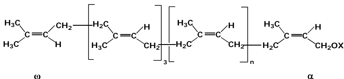
Figura 3. Estrutura da borracha natural. Valores de n = 320-360 (girassol), 1000-2000 ( Soligado altíssima ) e \sim 10.000 ( Hevea brasiliensis ). X = \text{H} ( Soligado altíssima ), \text{COR} ( Hevea brasiliensis ). O grupo \omega -isopropilideno não foi detectado na BN da seringueira. 10
