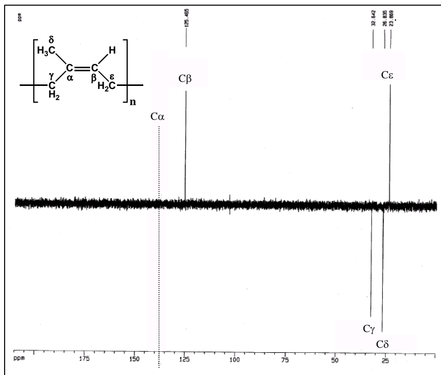
Figura 47. Espectro DEPT do MAT 2.
