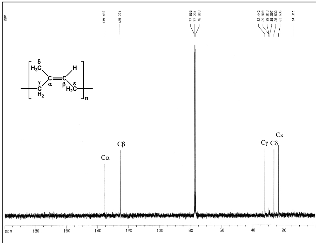
Figura 46. Espectro de RMN ^{13}\text{C} do MAT 2 obtido em \text{CDCl}_3 .
