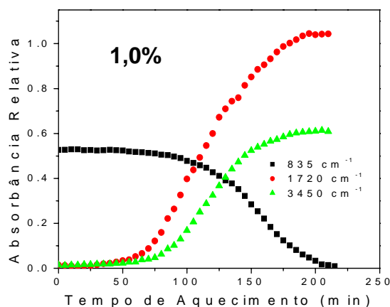
Figura 32. Cinética de termo-oxidação a 140°C do poli(1,4- cis -isopreno) sintético na presença de 1,0% do CENT 1.
