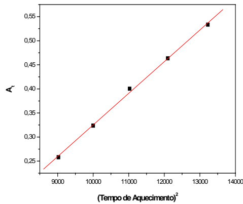
Figura 15. Representação sistemática de cálculo aplicada para determinação dos parâmetros cinéticos da degradação termo-oxidativa do PIS (banda em 1720\text{ cm}^{-1} ).
