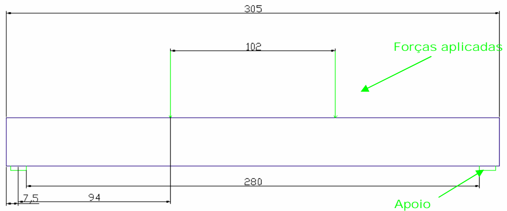
Figura 4.8 Localização dos pontos de apoio e de aplicação das forças nos modelos
