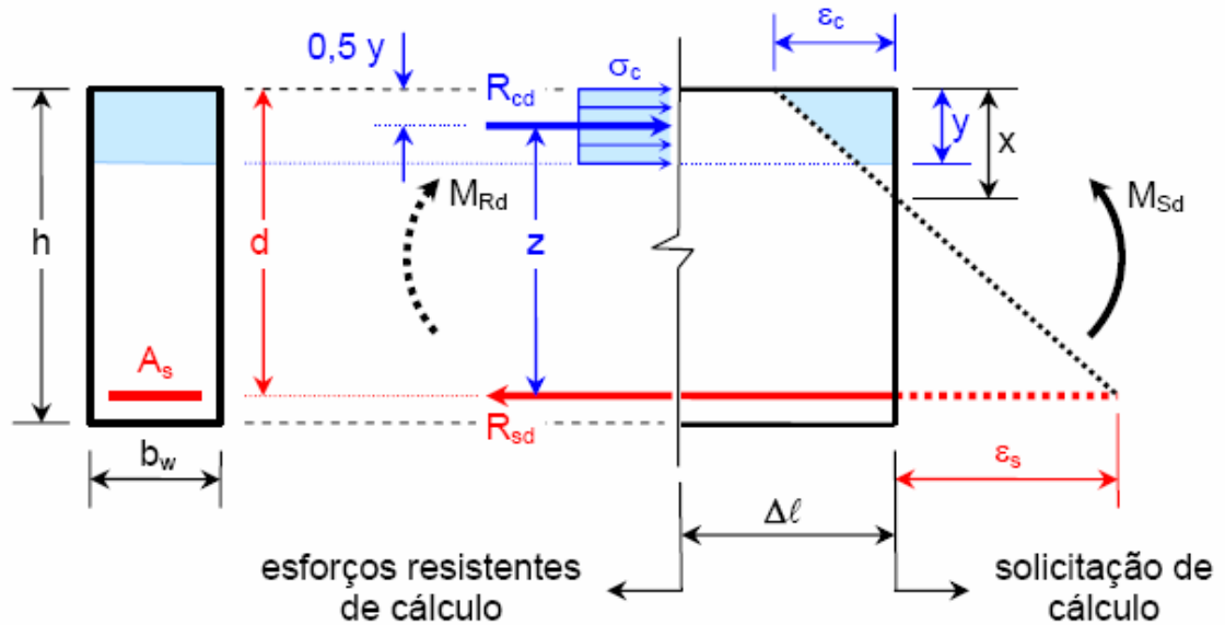
Figura 5.27 Seção transversal típica de uma viga de concreto simplesmente armada
