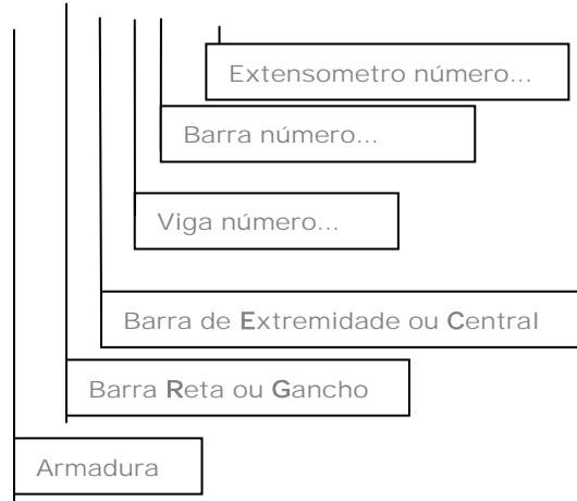
Figura 4.5 - Nomenclatura dos extensômetros
