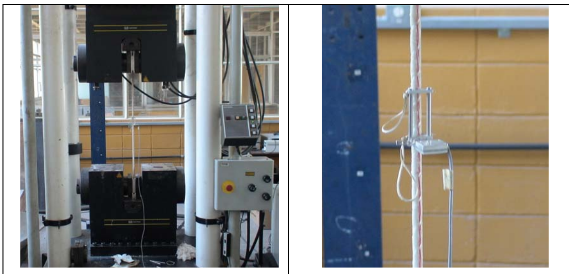
Figura 4.14 Ensaio de tração direta das GFRP
