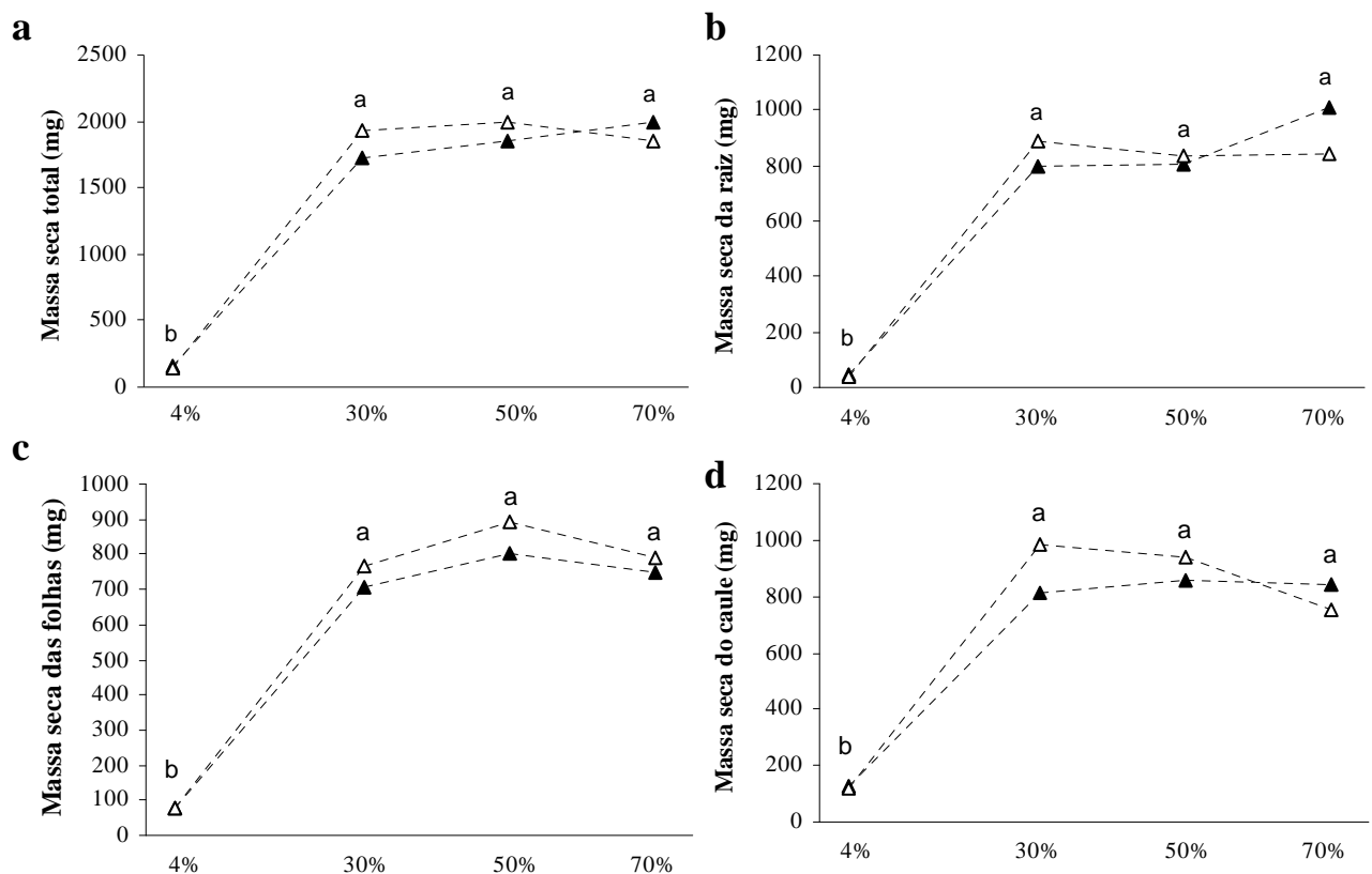
Figura 4. Biomassa de plantas de Tabebuia avellanedae Lorentz ex Griseb. com quatro meses de idade, cultivadas em diferentes intensidades de luz e colonizadas por fungos micorrízicos nativos (△) e selecionados (▲). a) Massa seca total; b) massa seca da raiz; c) massa seca das folhas; d) massa seca do caule. Valores com a mesma letra, para o efeito luz, não diferem significativamente entre si pelo teste Tukey ( p \leq 0,05 ).
