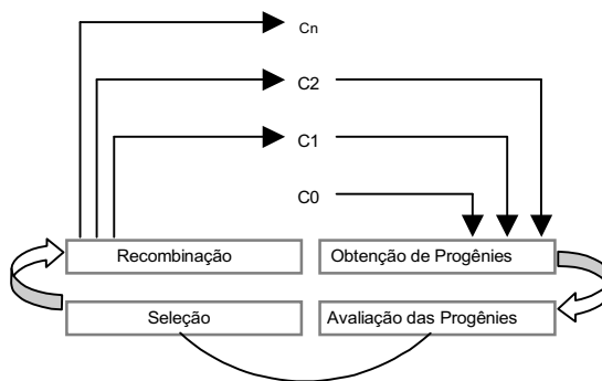
FIGURA 2. Representação esquemática da seleção recorrente.
