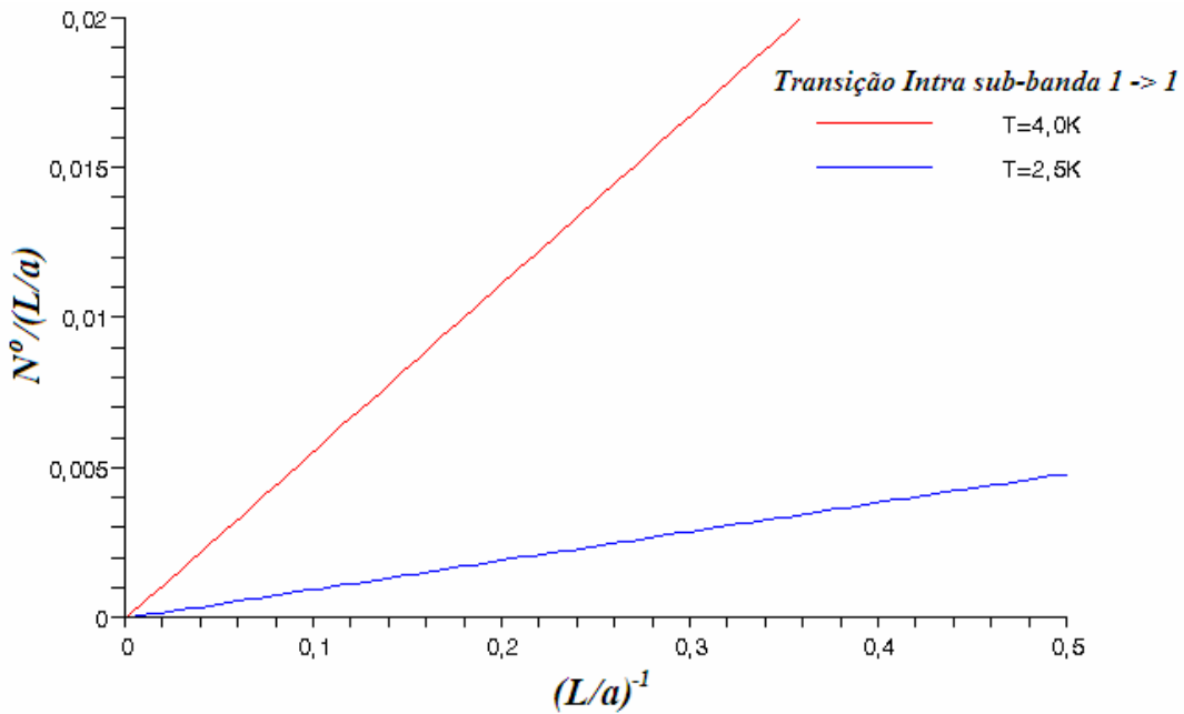
Fig. 4.5: N^{(0)}/(L/a) expressada como função do inverso da largura do poço quântico para dois valores de temperatura: T = 4,0 K (linha vermelha) e T=2,5 K (linha azul). A energia dos magnons foi tomada fixa e igual a 1,0 meV.
