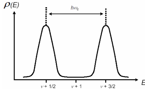
Fig. 2.6. Densidade de estado com alargamento de nível de Landau. Aqui \nu = (n_e/n_L) = (n_e h/eB) é o fator de preenchimento ou número de níveis de Landau ocupados.
