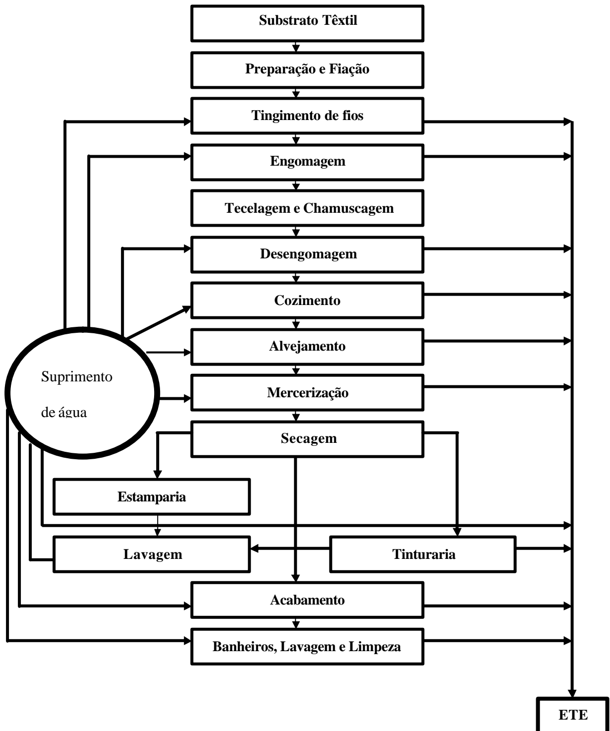
FIGURA 05: Etapas das características do processamento de tecidos de algodão e sintéticos.
