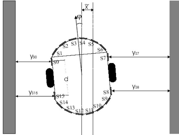
Figura 15: Disposição dos sensores ultra-sônicos e as variáveis de estado \tilde{x} e \varphi .
