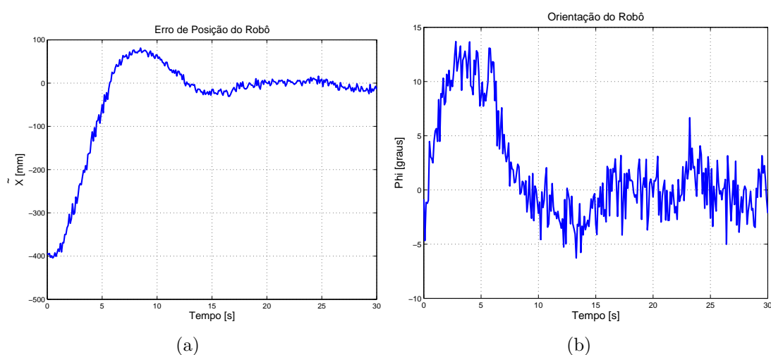
Figura 27: Erro de posição (a) e a orientação (b) do robô.
