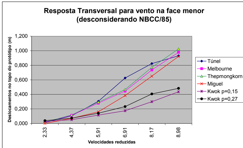
FIGURA 5.16 – Comparação dos resultados para vento com p=0,19 incidindo na face menor
