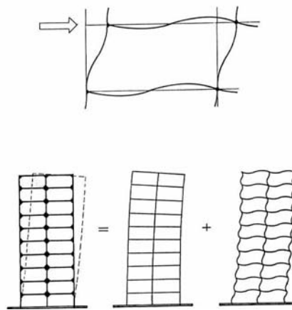
FIGURA 3.1 – Deformação na malha estrutural de um edifício alto, frente à ação de carregamentos laterais (Ellwanger, 1996)
