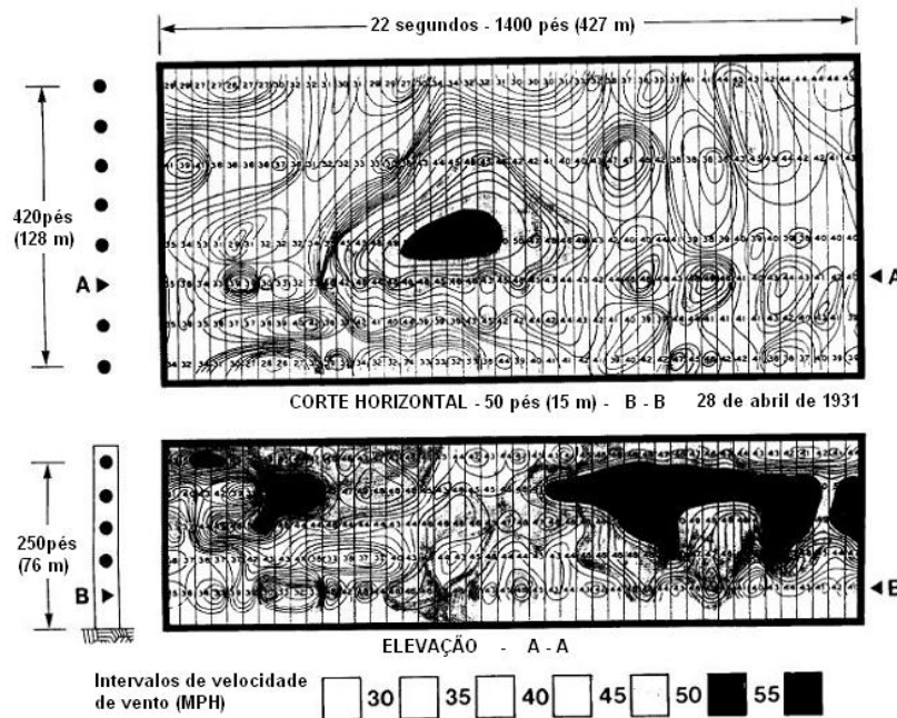
FIGURA 2.2 – Estrutura turbulenta do vento (Sherlock & Stout, 1937)
