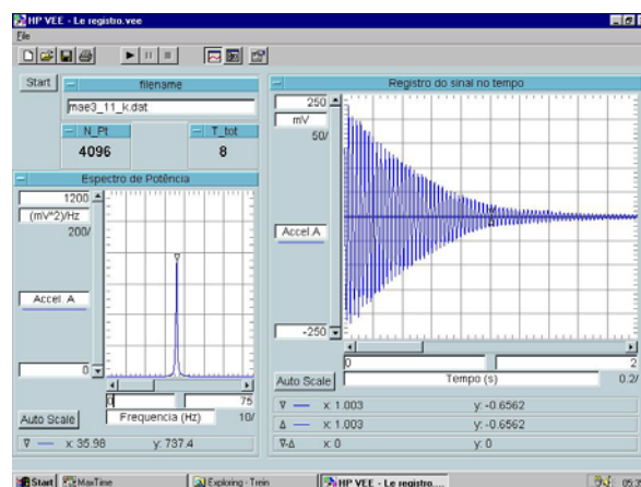
FIGURA 4.17 – Registro de vibração livre obtido pelo programa HP VEE 3.2, onde o modelo não se encontra em sua configuração final
