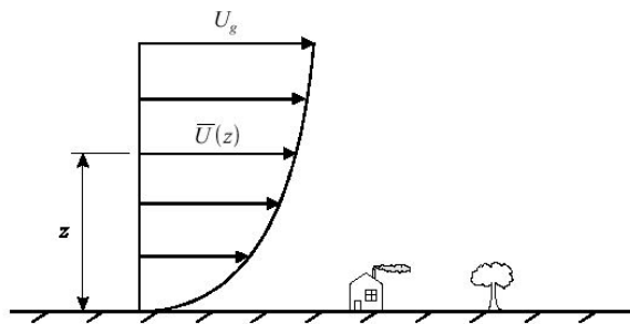
FIGURA 2.4 – Gradiente de velocidades do vento (Sparling, 1997)
