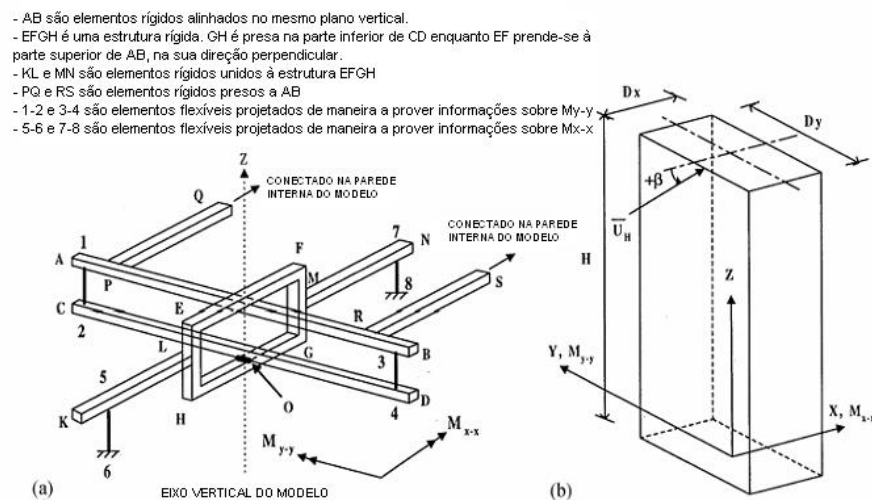
FIGURA 3.4 - Representação esquemática do BHA: (a) BHA, com 2 GDL; (b) modelo de edifício (Thepmonkorn et al., 1999)
