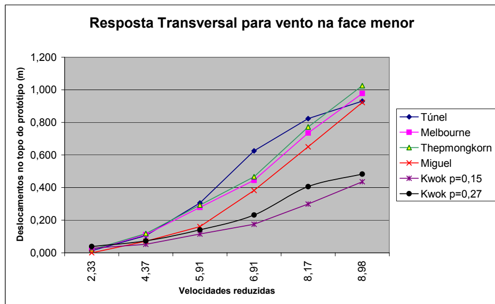
FIGURA 5.8 – Comparação dos resultados para vento com p=0,19 incidindo na face menor
