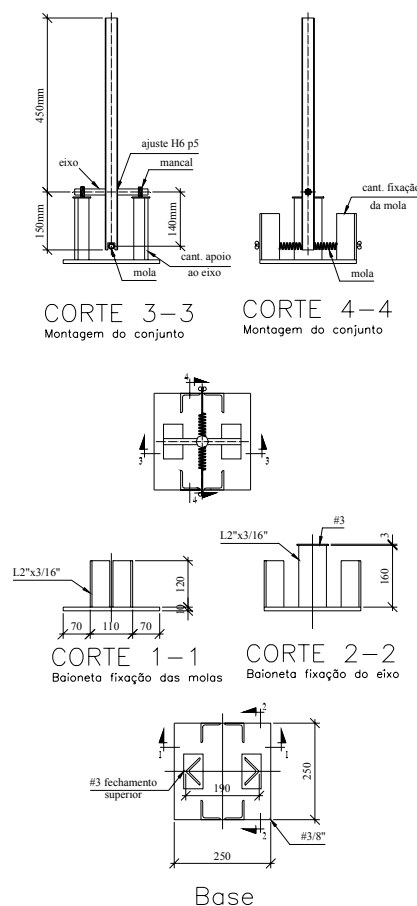
FIGURA 3.10 - Parte mecânica do modelo
