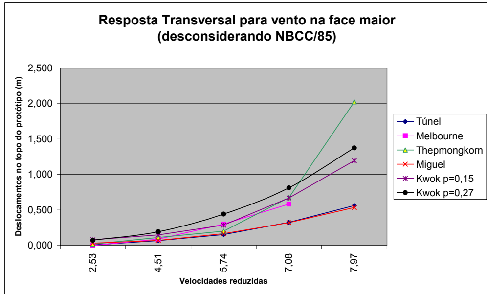
FIGURA 5.15 – Comparação dos resultados para vento com p=0,19 incidindo na face maior
