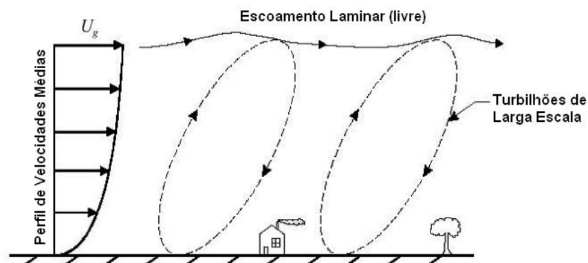
FIGURA 2.1 – Turbilhões e perfil de velocidades na camada limite atmosférica (Sparling, 1997)
