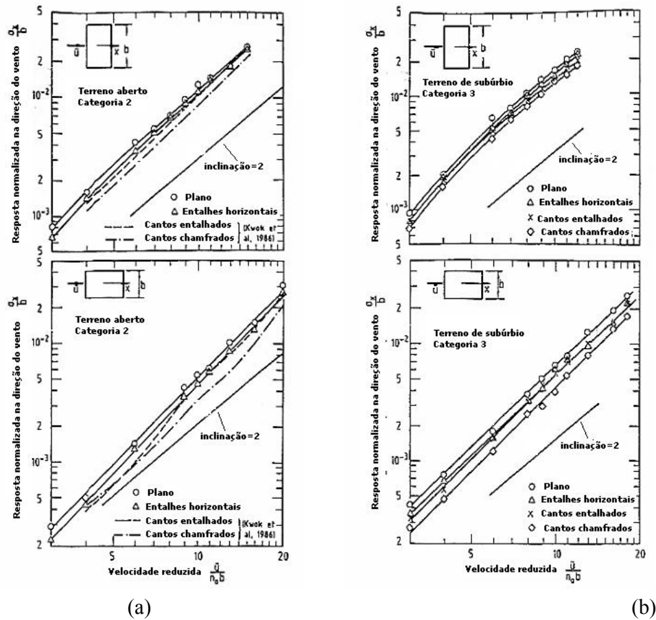
FIGURA 5.3 – Resposta Longitudinal no topo do protótipo ( CAARC Standard Tall Building ) para vento incidindo na face maior: (a) vento com p=0,15 ; (b) vento com p=0,27 (Kwok, 1988)
