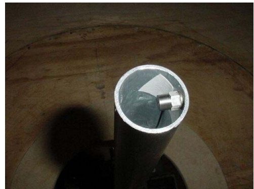
FIGURA 4.12 – Fixação do acelerômetro no modelo
