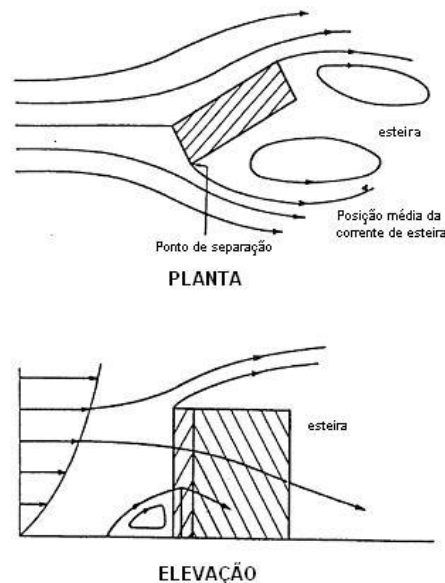
FIGURA 2.7 – Ação do vento em seções prismáticas e em edificações alteadas (Sparling, 1997)
