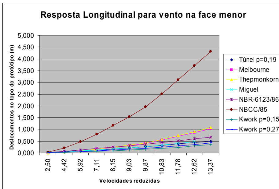
FIGURA 5.6 – Comparação dos resultados para vento com p=0,19 incidindo na face menor
