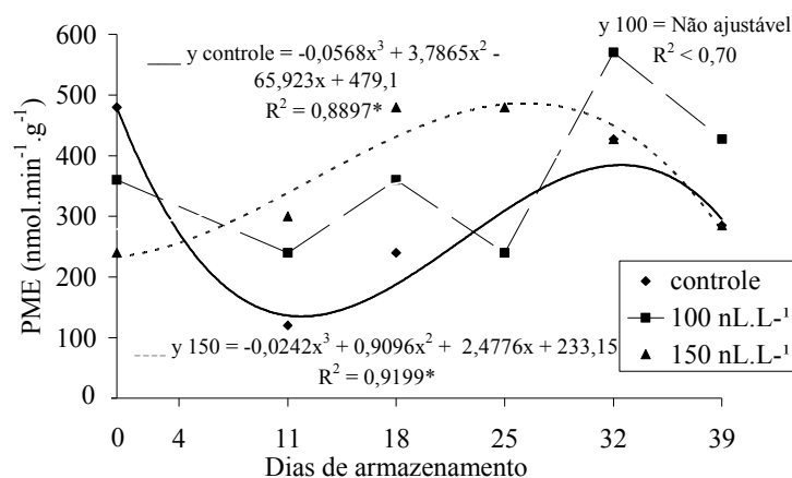
FIGURA 43 Curvas e equações de regressão de atividade de pectinametilsterase (PME) em mangas 'Palmer' submetidas ao 1-MCP e armazenadas sob temperatura refrigerada ( 10 \pm 1^\circ\text{C} ) e temperatura ambiente por 4 dias. Lavras, MG, 2005.
