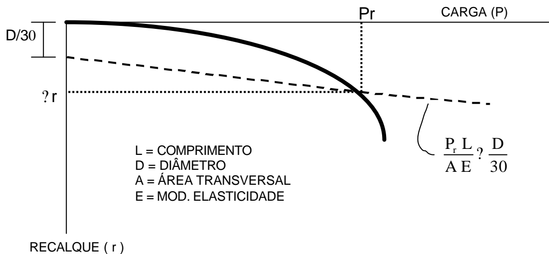
Figura 4.2 – Carga de ruptura pela NBR 6122/96
