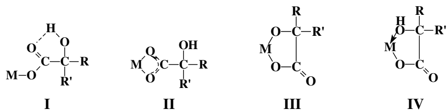
FIGURA 1 Coordenação dos ácidos hidroxicarboxílicos com metais
