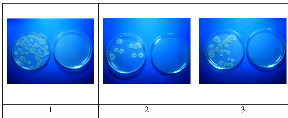
FIGURA 2B Fotografia das placas de crescimento micelial de Aspergillus fumigatus (1), Penicillium comune (2) e Penicillium solitum (3) na concentração de 50ppm.
