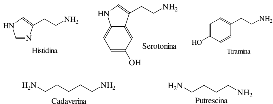
FIGURA 8 Fórmulas estruturais de aminas biogênicas
