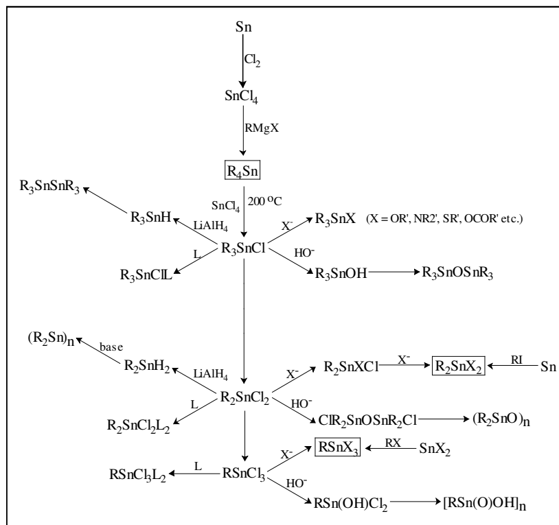
FIGURA 2 Esquema de síntese de derivados organoestânicos a partir de \text{SnCl}_4 (Davies & Smith, 1982)
