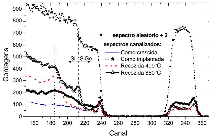
Fig. 5.6. Espectros de RBS/C de uma amostra como crescida ( \frac{3}{4} ), da amostra como implantada na fluência de 7 \times 10^{15} He \text{cm}^{-2} e energia de 30 keV ( \star ) e amostras implantadas e recozidas a 400^\circ\text{C} (---) e 850^\circ\text{C} (-D-). Os espectros foram obtidos com um feixe de \text{He}^+ de 1,2 MeV.
