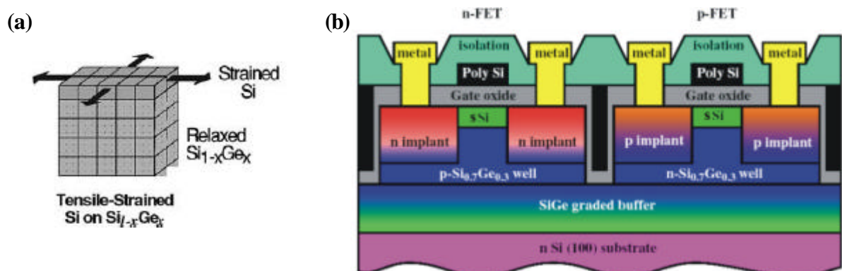
Fig. 1.1. (a) Camada ultrafina de Si tensionado (sSi) sobre SiGe relaxado [6]. (b) Esquema típico de dois transistores CMOS com canal de sSi [2].
