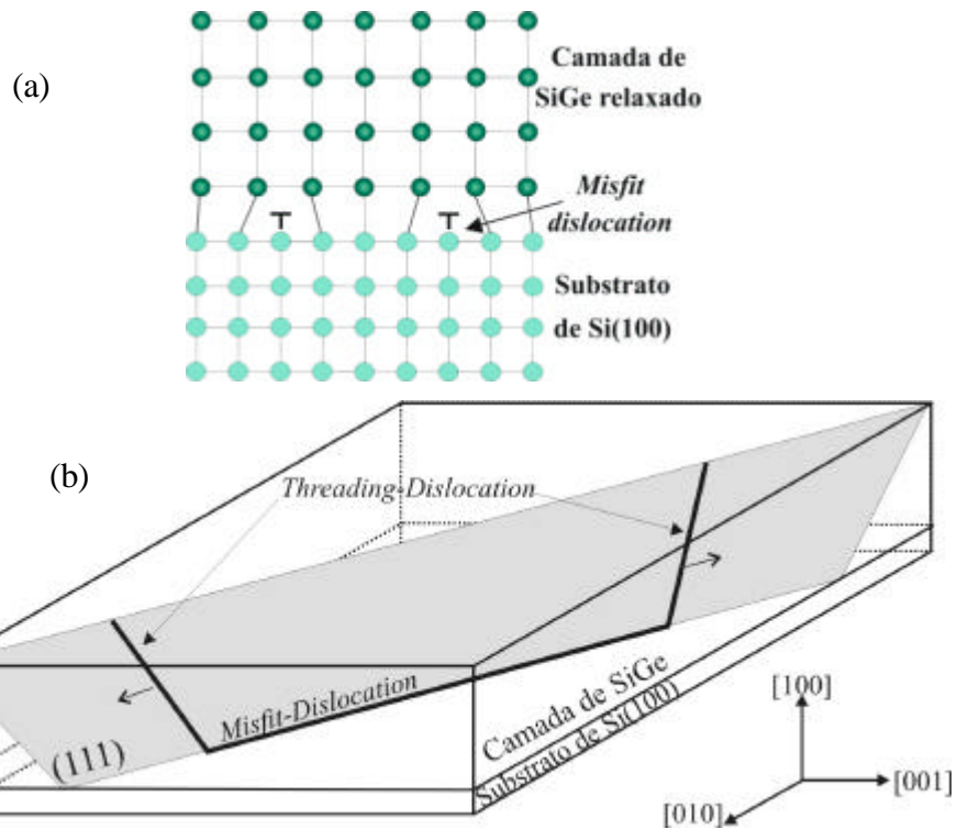
Fig. 1.5. Discordâncias de misfit (MDs) na interface SiGe-Si e discordâncias tipo threading (TDs) na camada de SiGe.
