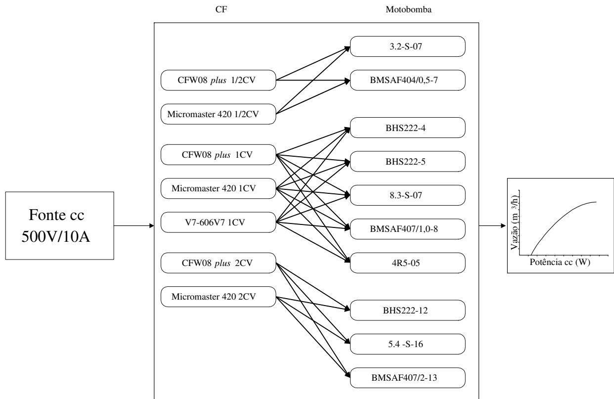
Figura 3.11: Ensaios realizados com a fonte de tensão cc 500 V/ 10 A.
