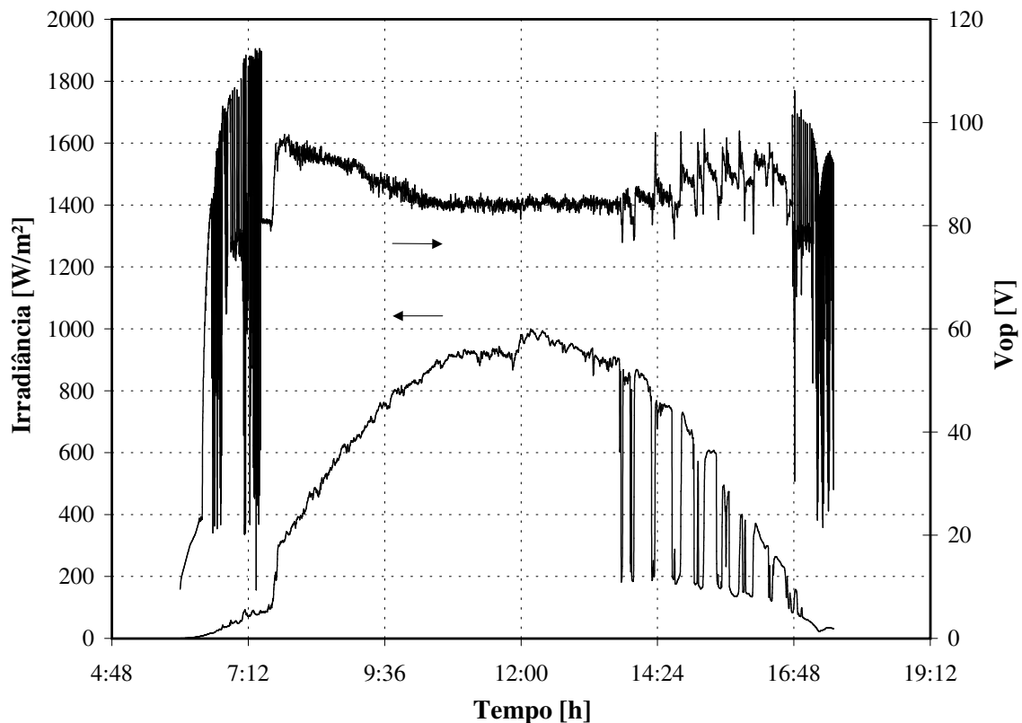
Figura 2.18: Variação de V_{op} , SBFCV.
