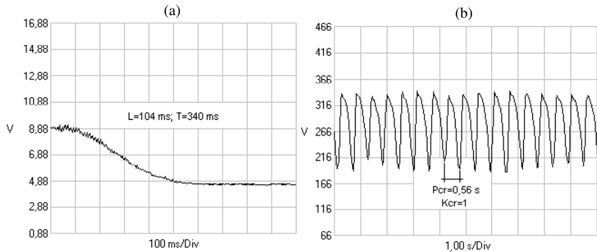
Figura 2.12: Caracterização do processo para o SBFCF 2: (a) - curva de reação; (b) - oscilações estáveis.
