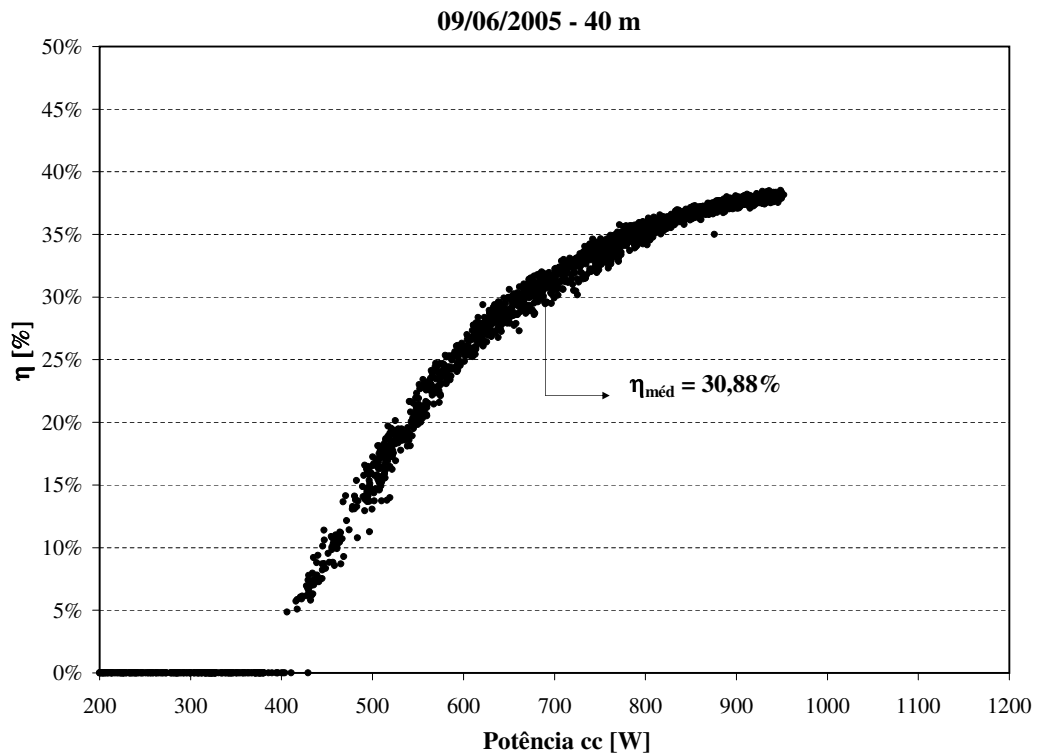
Figura 3.15: Eficiência média do conjunto CF+motobomba.
