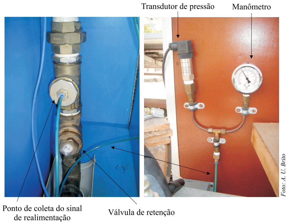
Figura 3.4: Detalhes da bancada de ensaio - ponto de coleta do sinal de realimentação, válvula de retenção, manômetro e transdutor de pressão.
