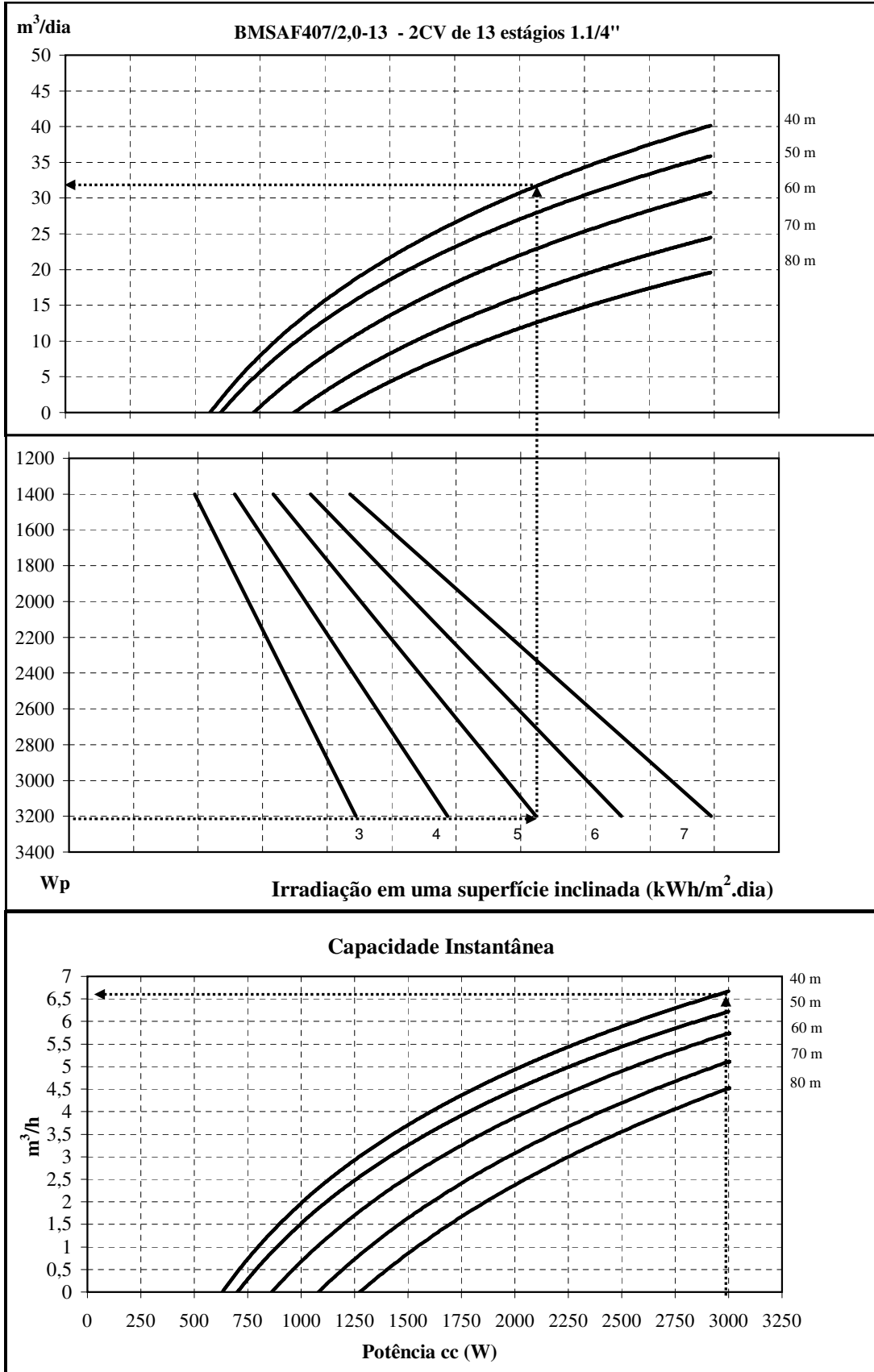
Figura 3.21: Ábaco de dimensionamento.
