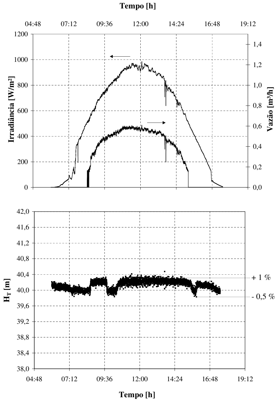
Figura 3.9: Variação de H T ao longo do dia - SBFCV.
