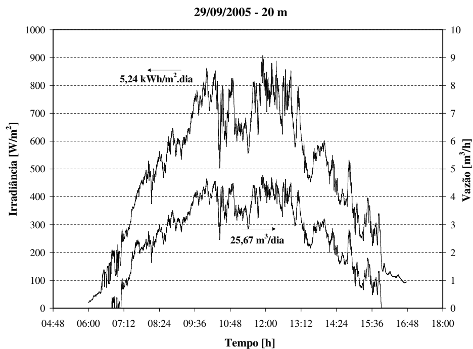
Figura 2.2: Volume bombeado - motobomba SQF 5A-6 - centrífuga.
