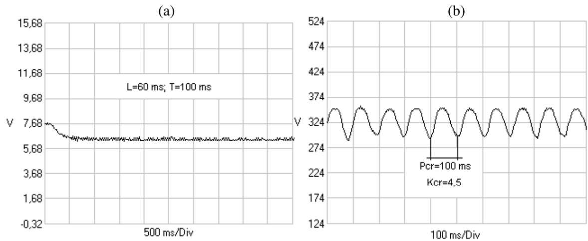
Figura 2.11: Caracterização do processo para o SBFCF 1: (a) - curva de reação; (b) - oscilações estáveis.
