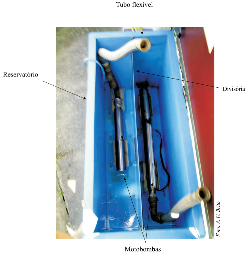
Figura 3.3: Detalhes da bancada de ensaio - reservatório, divisória, motobombas e tubos flexíveis.
