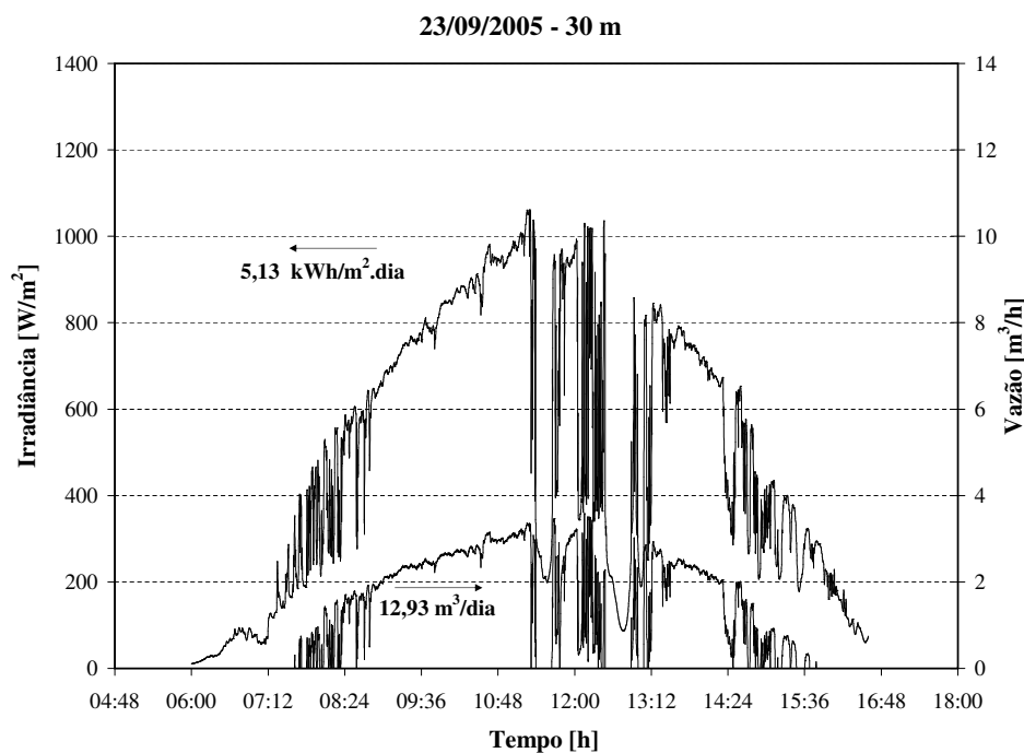
Figura 2.4: Volume bombeado - motobomba SQF 5A-6 - centrífuga.
