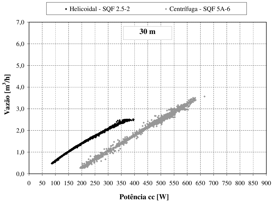
Figura 2.6: Curva de capacidade instantânea - motobomba helicoidal e centrífuga (30 m).
