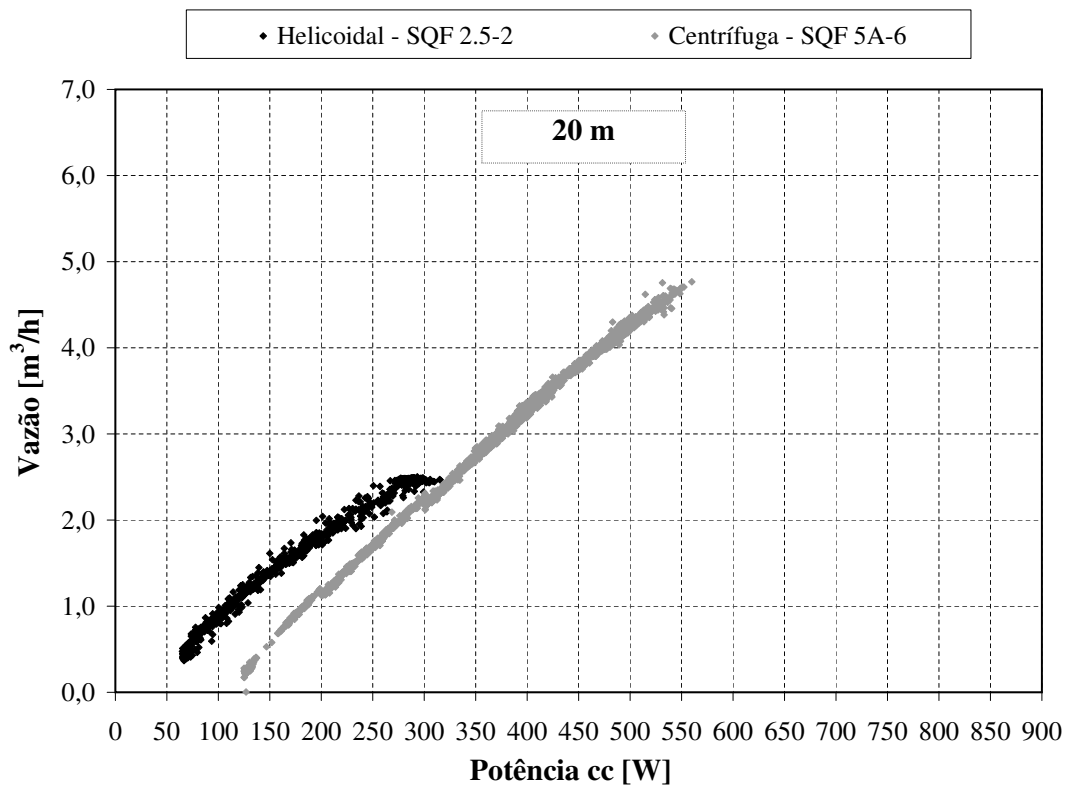
Figura 2.5: Curva de capacidade instantânea - motobomba helicoidal e centrífuga (20 m).
