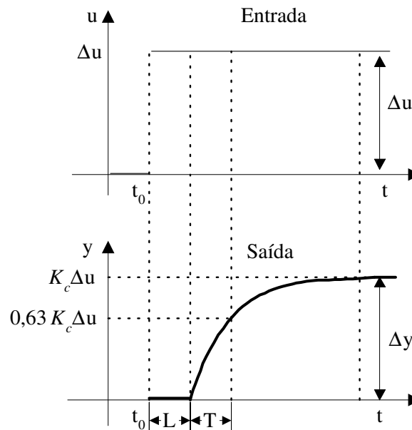
Figura 2.8: Exemplo de resposta do processo a um degrau na variável de entrada.
