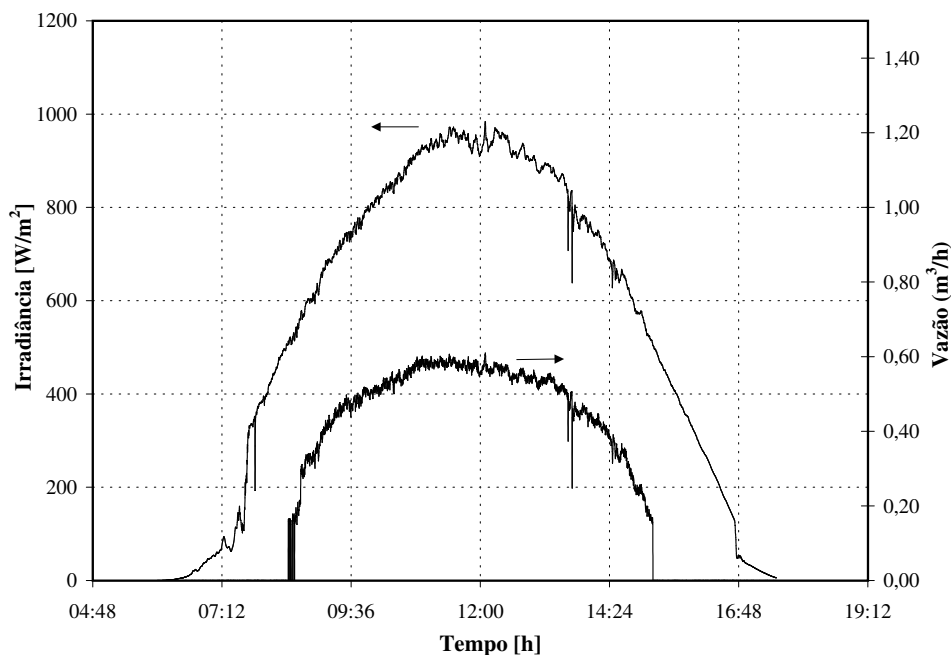
Figura 1.4: Variação da vazão e irradiância ao longo do dia.
