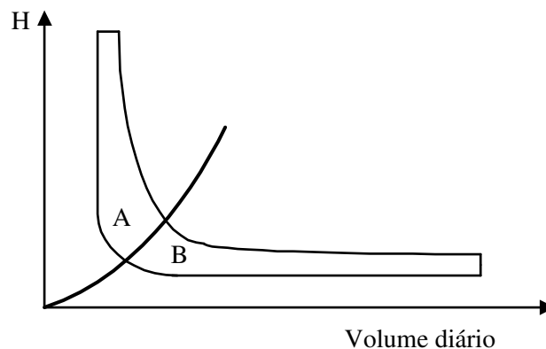
Figura 2.7: Curvas indicativas de utilização de motobombas de deslocamento positivo (A) e centrífugas (B).
