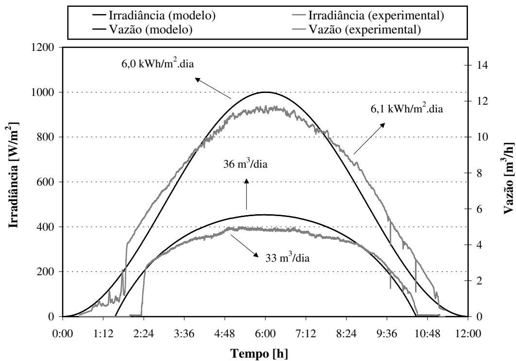
Figura 3.27: Comparação entre os valores de irradiância e vazão - modelo x experimental.
