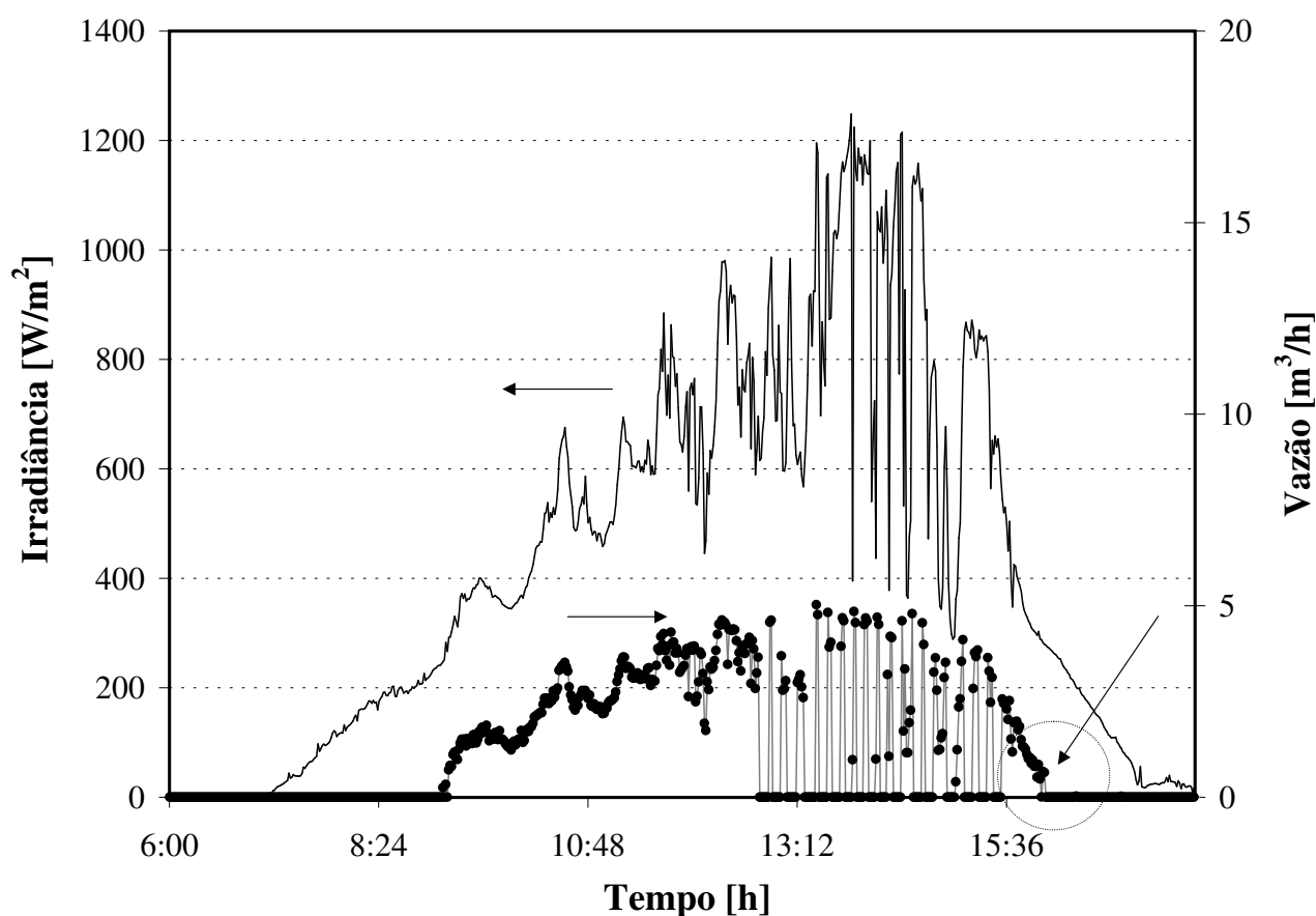
Figura 3.24: Variação da irradiância e vazão - 19/01/2006.
