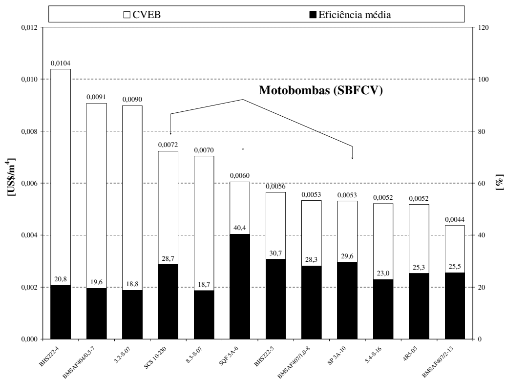
Figura 3.29: CVEB e Eficiência média, Cenário II.
