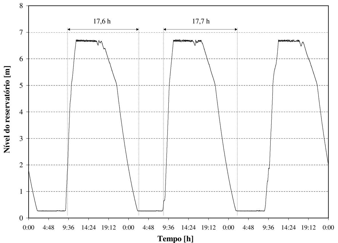
Figura 3.25: Variação do nível do reservatório ao longo do dia.
