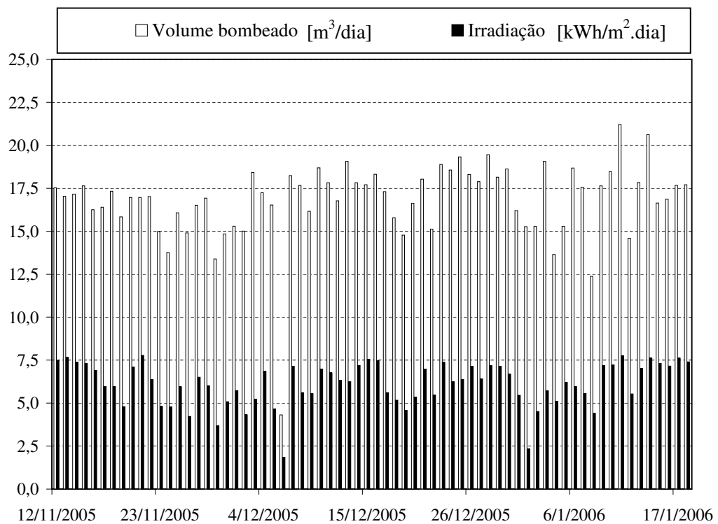
Figura 3.23: Volume bombeado diário de água.
