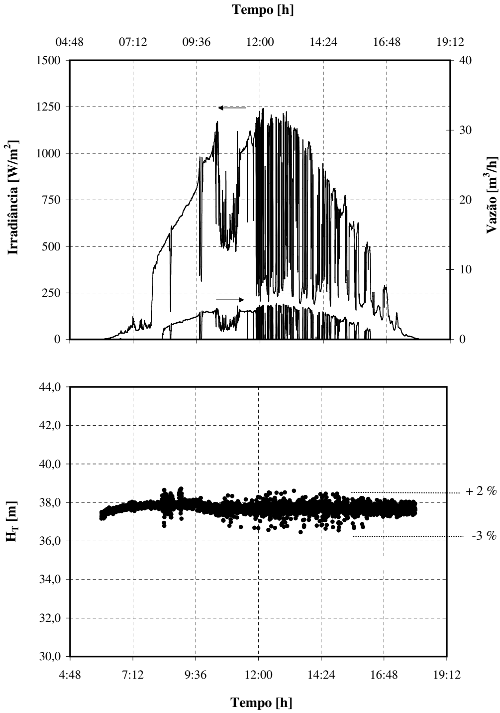
Figura 3.10: Variação de H T ao longo do dia - SBFCF.
