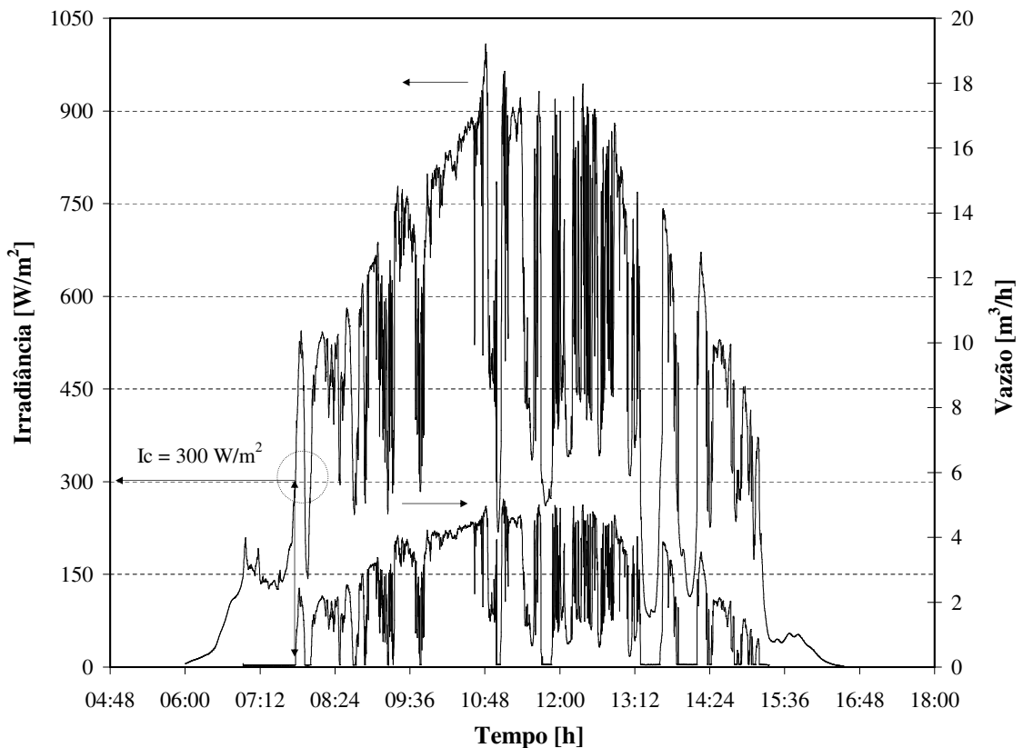
Figura 1.6: Valor de I_c para a motobomba de 1/2 CV operando a 10 m.
