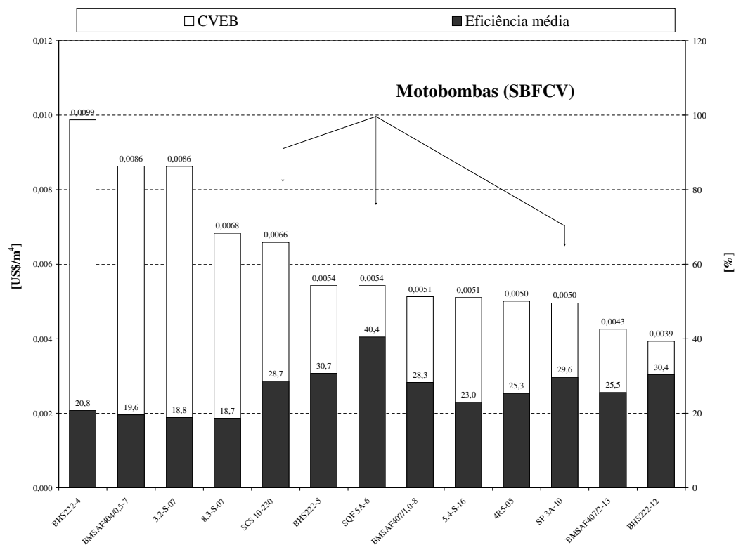
Figura 3.28: CVEB e Eficiência média, Cenário I.
