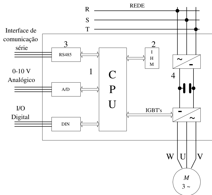
Figura 1.2: Diagrama de blocos de um conversor de frequência (CAPELLI, 2002).
