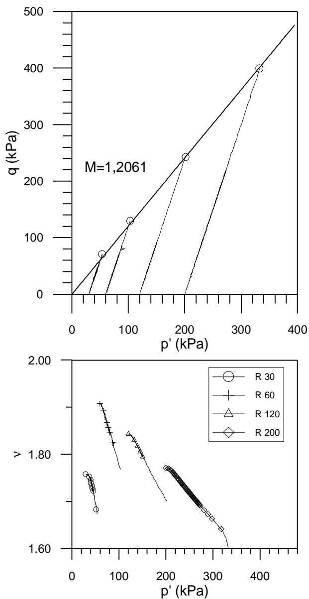
Figura 4-15: Trajetórias de tensões efetivas dos ensaios R e curvas p':n .
