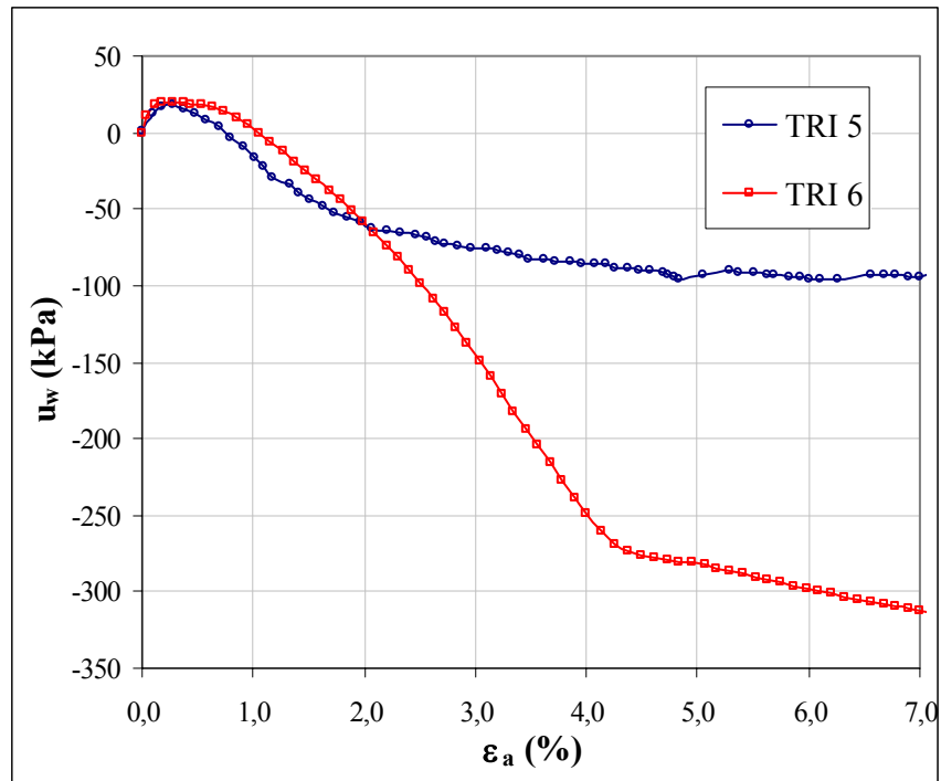
Figura 6.17: curvas de geração de poro-pressão para os corpos-de-prova com relação vazios/cimento = 55
