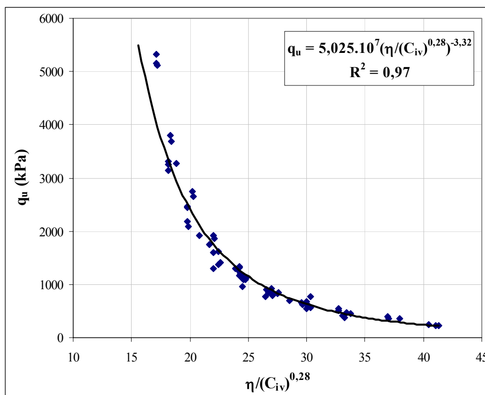
Figura 7.21: relação vazios/cimento expresso em termos da porosidade e do teor de volumétrico de cimento
