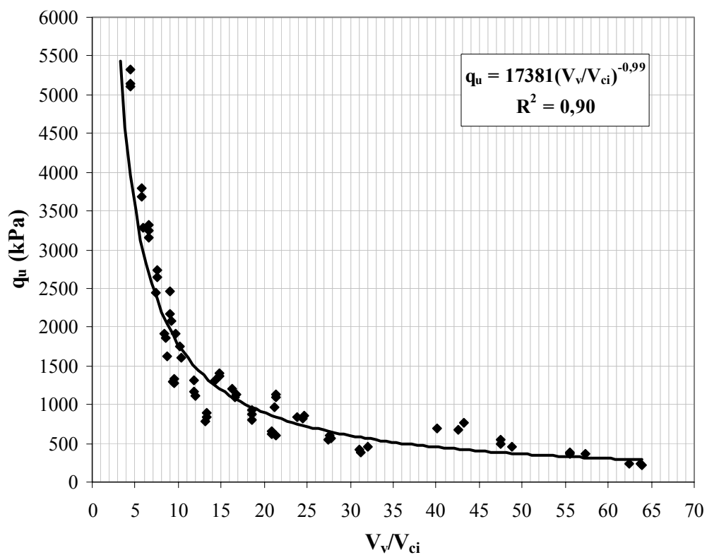
Figura 6.7: relação vazios/cimento como proposta por LARNACH (1960) versus resistência à compressão simples
