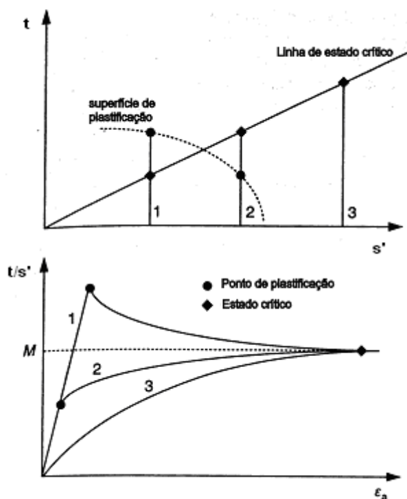
Figura 7.10: comportamento idealizado de solos cimentados onde o efeito da cimentação é preponderante (CUCCOVILLO & COOP, 1999 adaptado de COOP & ATKINSON, 1993)
