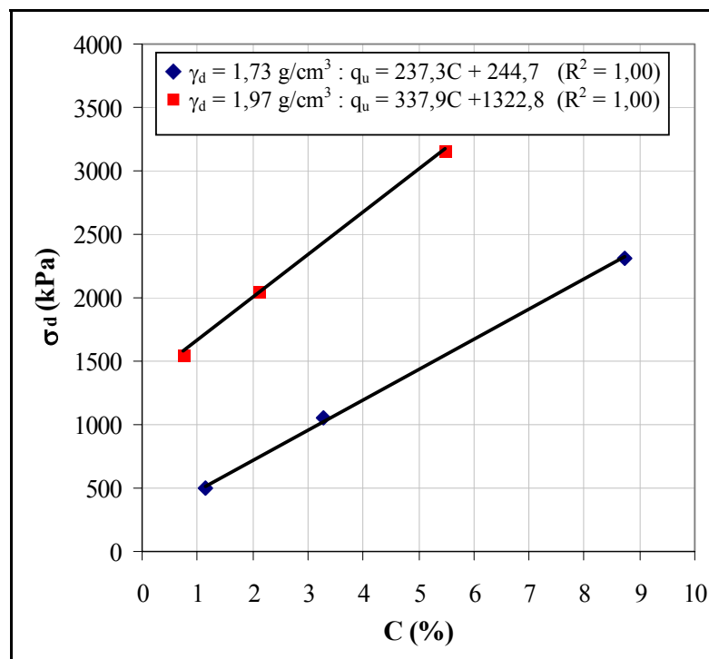
Figura 7.9: variação da resistência de pico dos ensaios triaxiais não-drenados em função do teor de cimento
