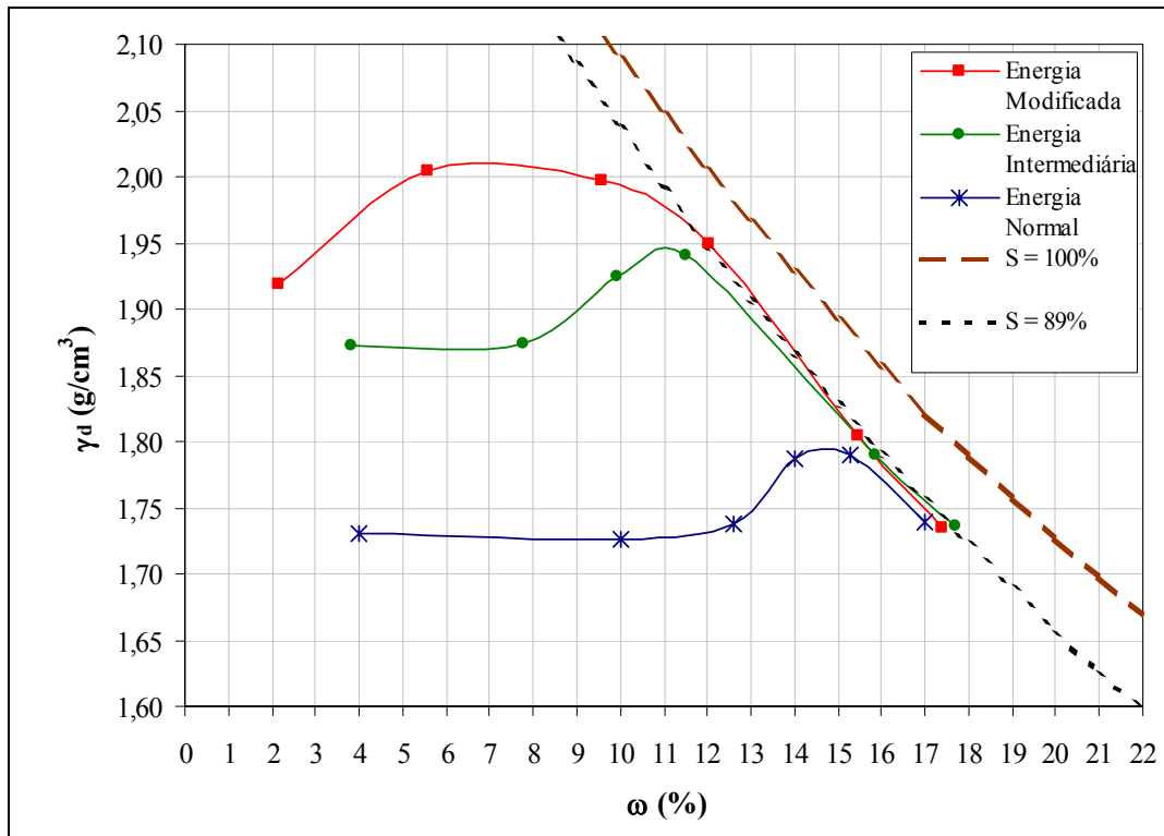
Figura 5.9: curvas de compactação do solo residual de arenito Botucatu
