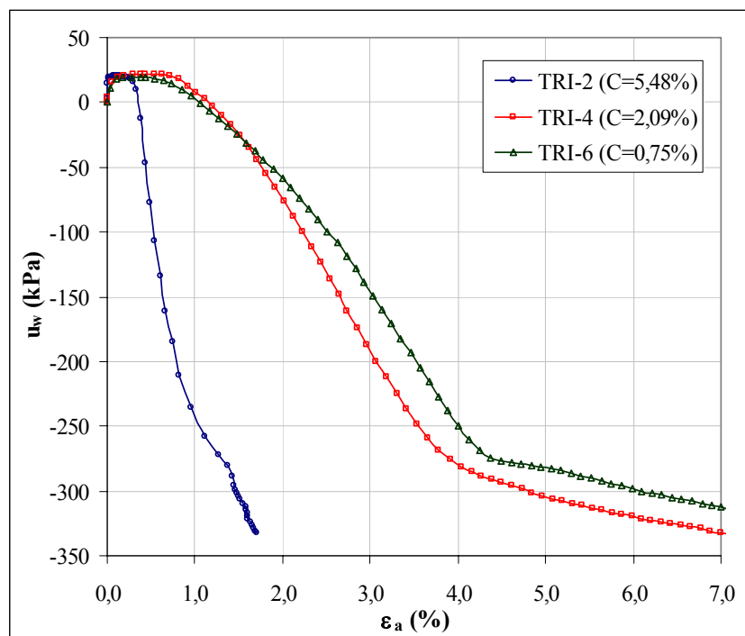
Figura 7.7: curvas geração de poro-pressão versus deformação axial dos corpos-de-prova com \gamma_d = 1,97 \text{ g/cm}^3
