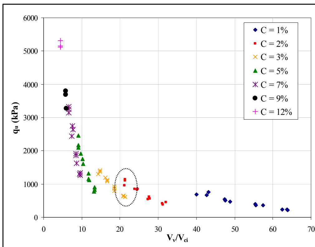
Figura 7.15: relação vazios/cimento conforme definição de LARNACH (1960)
