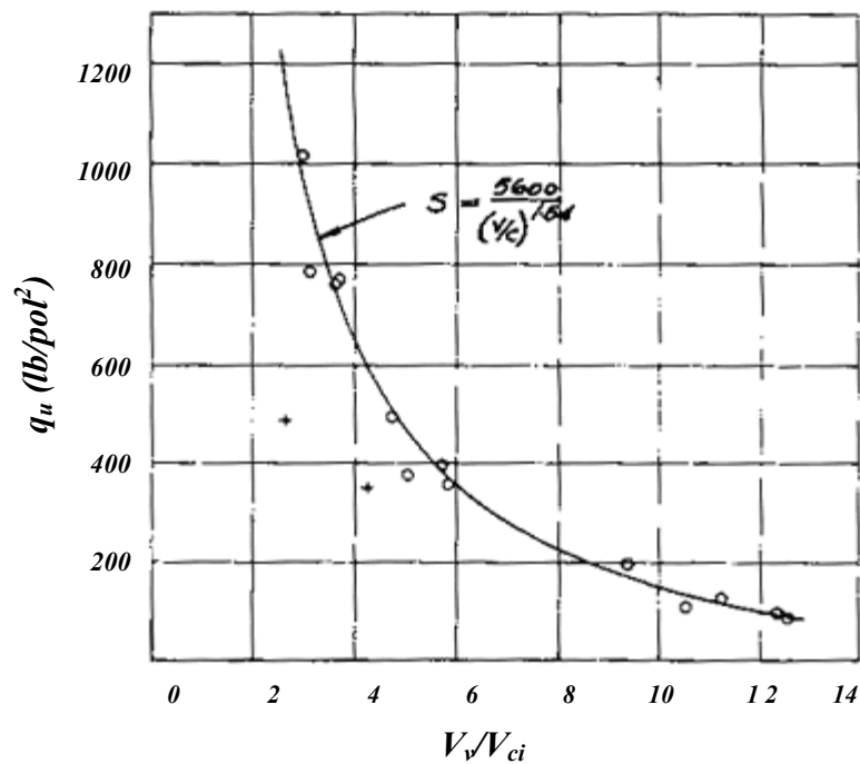
Figura 3.1: relação vazios/cimento versus resistência à compressão simples (adaptado de LARNACH, 1960)
