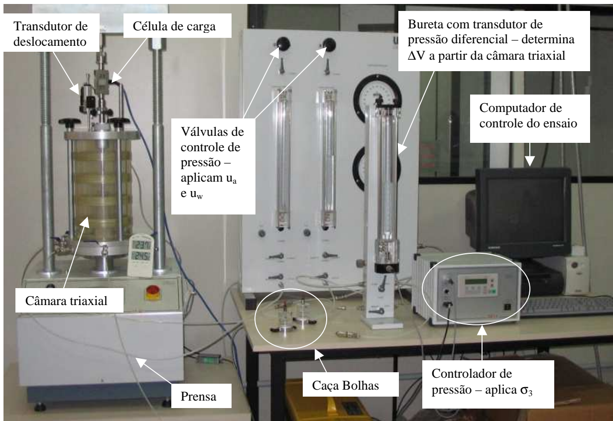
Figura 3.5 – Equipamento de ensaio triaxial para realização de ensaios não saturados.
