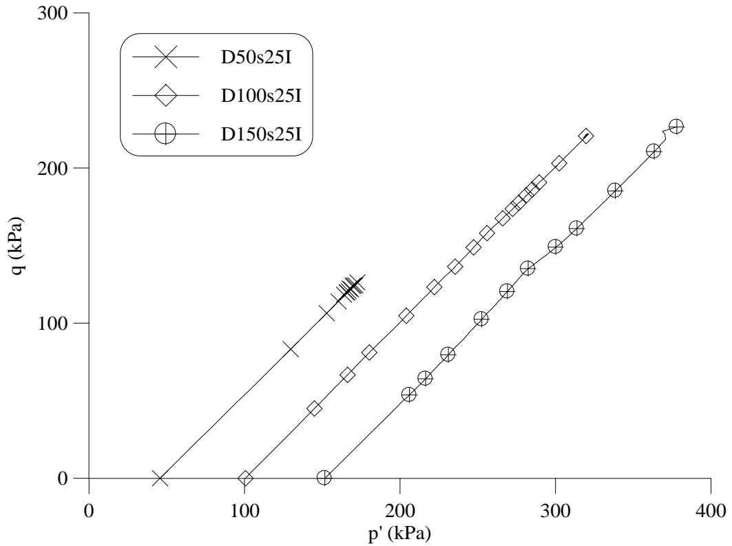
Figura 5.15 – Gráficos p' versus q dos ensaios triaxiais com sucção controlada drenados em corpos de prova indeformados para um nível de sucção de 25 kPa.
