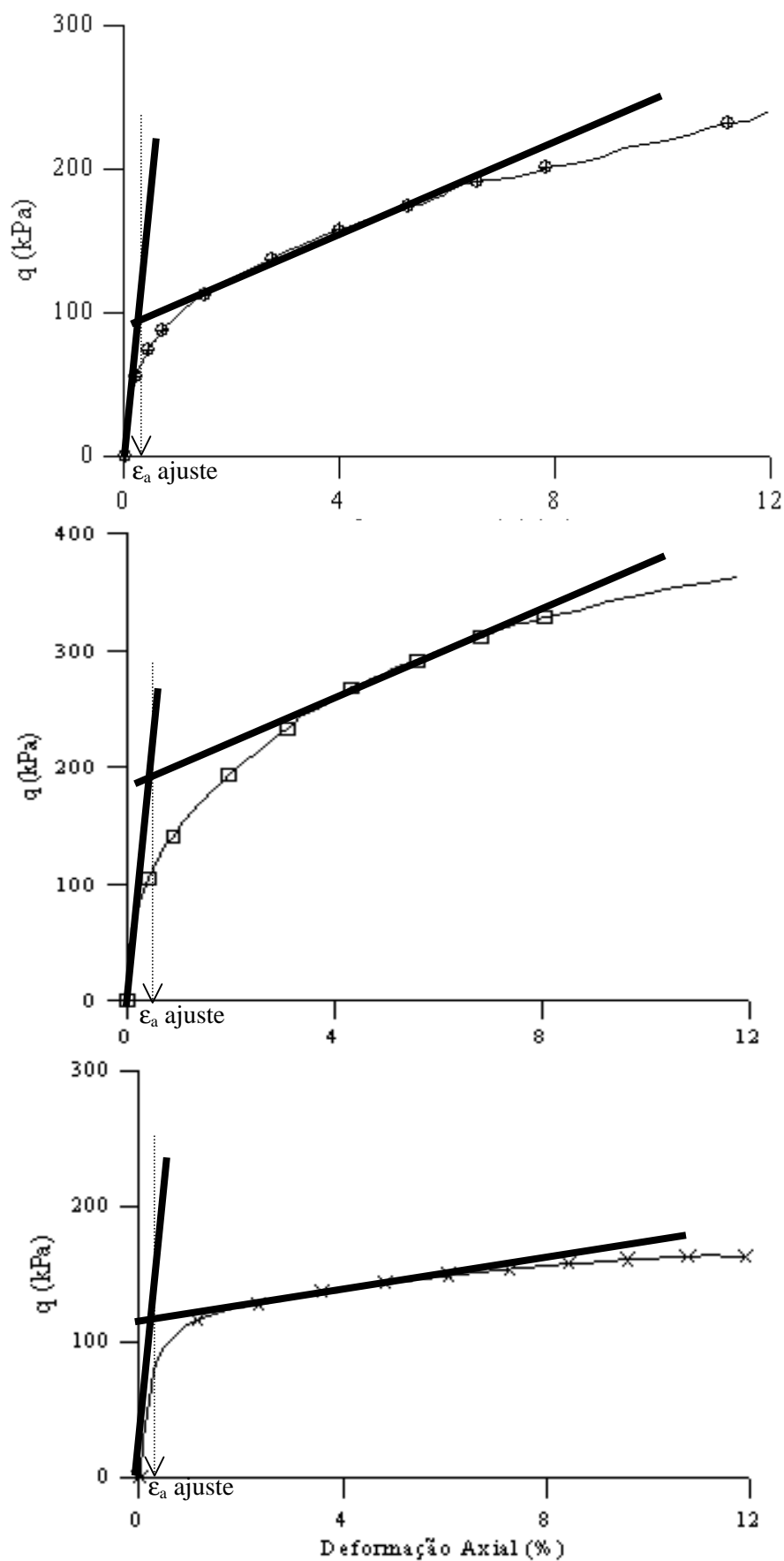
Figura 5.32 – Exemplos de aplicação do método de ajustes das curvas tensão versus deformação axial.
