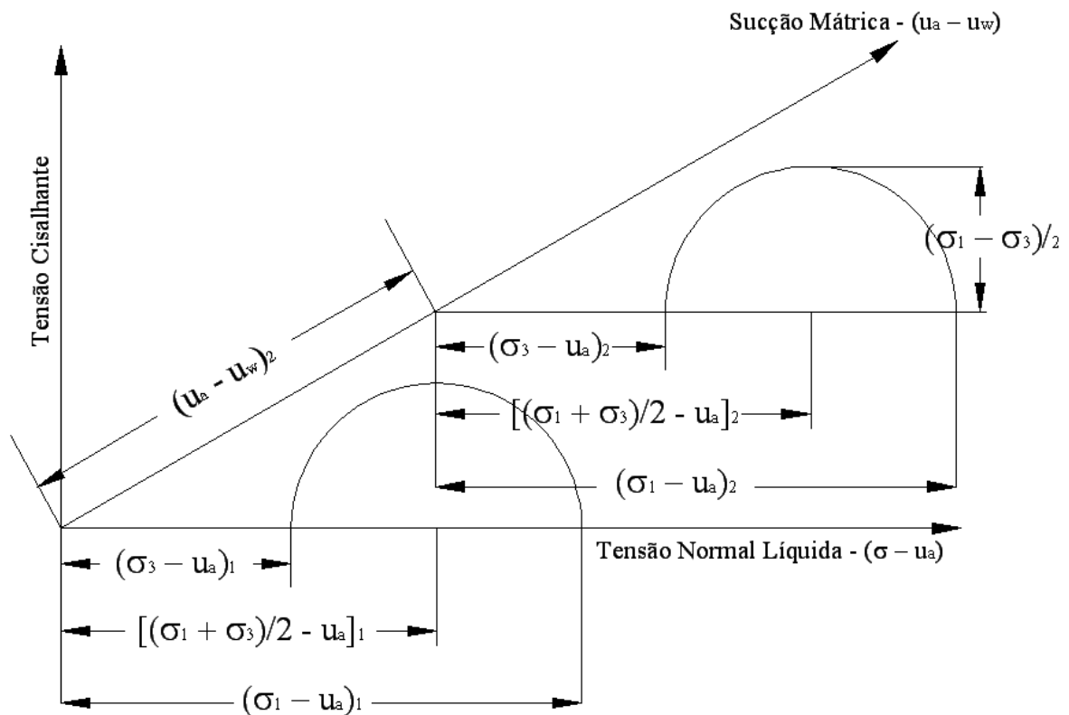
Figura 2.3 – Círculo de Mohr estendido para solos não saturados (Fredlund, 1979).
