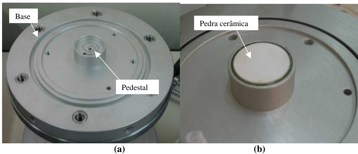
Figura 3.4 – Base da câmara triaxial: (a) com a ranhura e (b) com a pedra de alto valor de entrada de ar colada.
