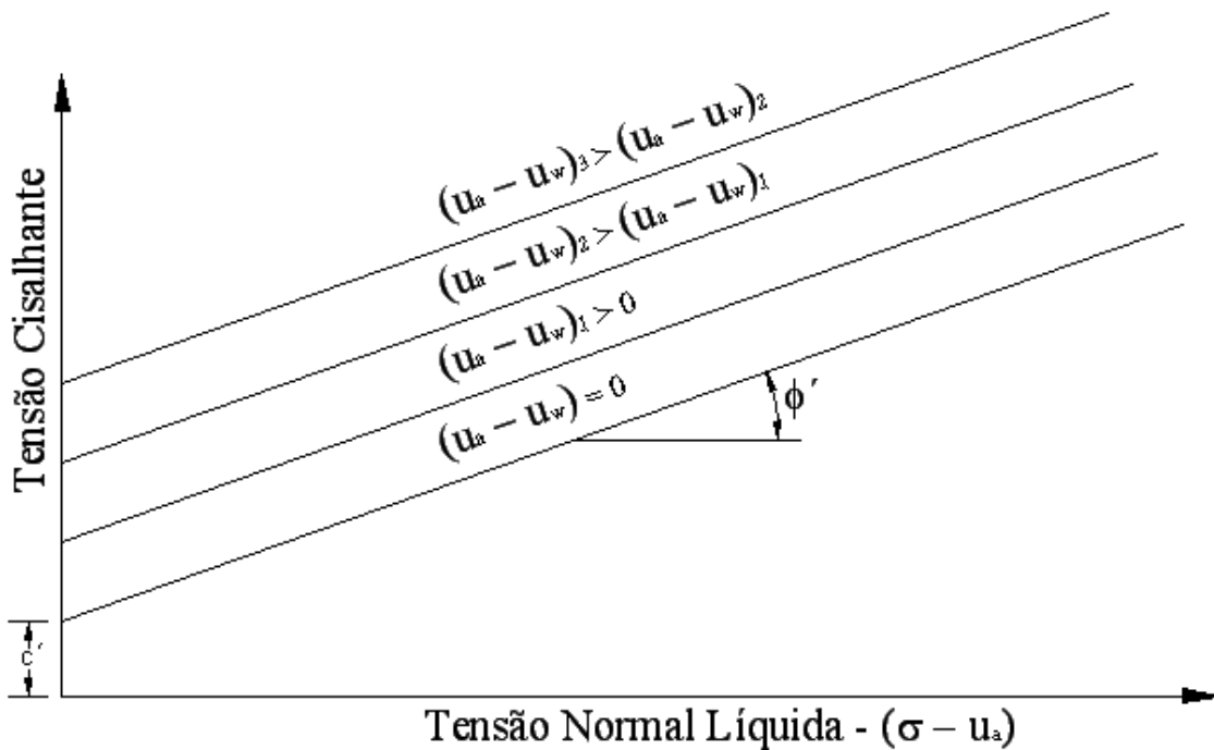
Figura 2.5 – Representação gráfica da resistência ao cisalhamento em um plano (Ho e Fredlund, 1982).
