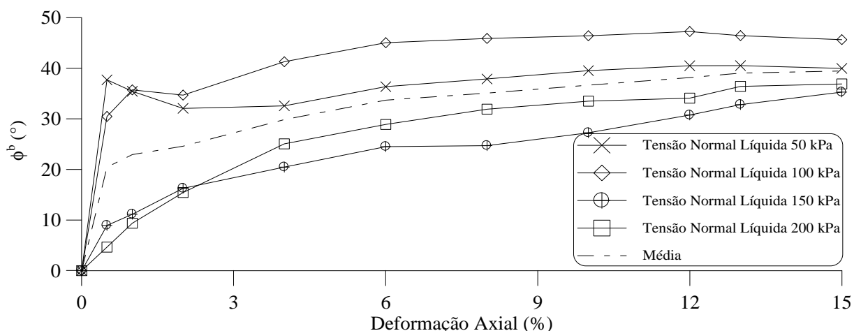
Figura 5.24 – Variação do valor de \phi^b com a deformação axial para os ensaios com sucção controlada drenados.
