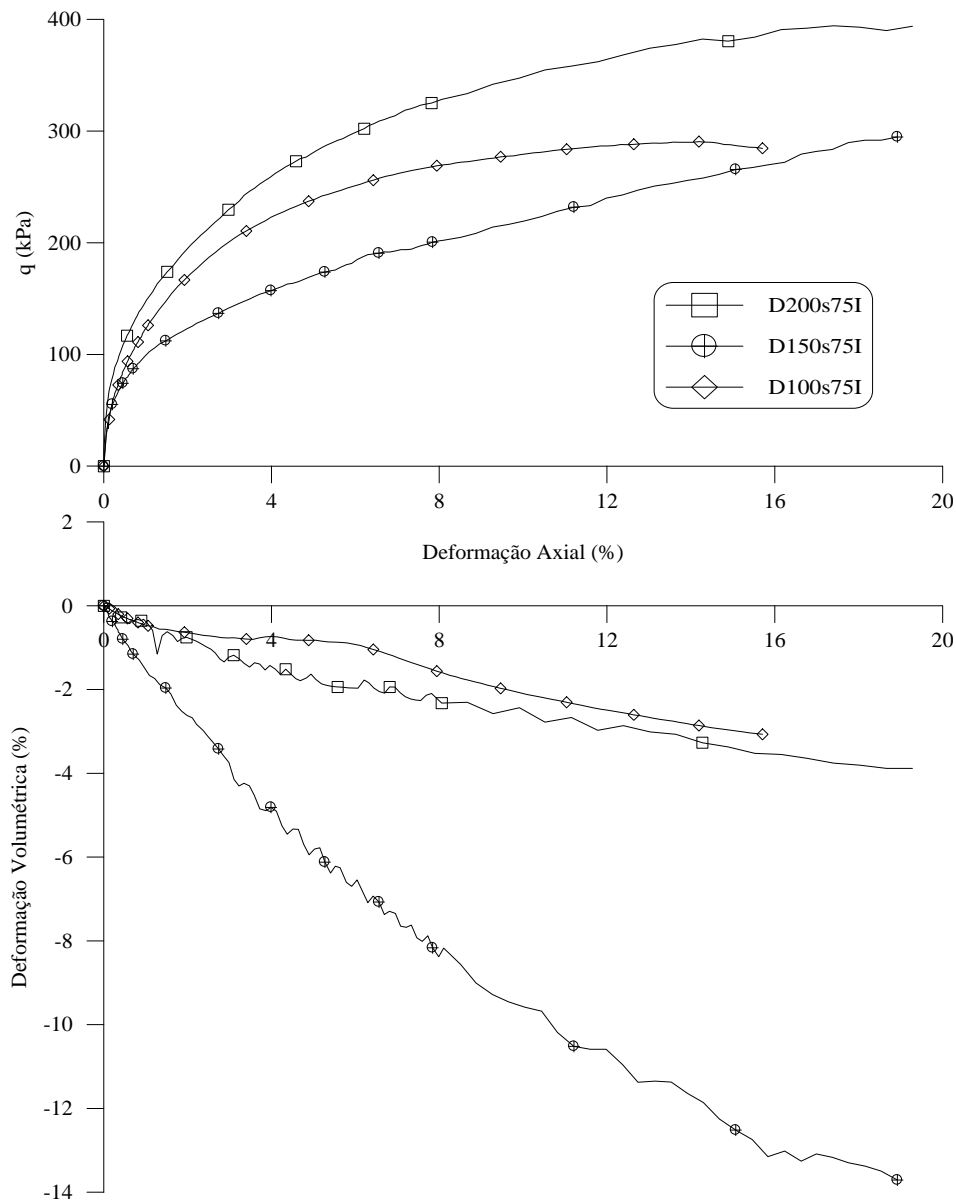
Figura 5.12 – Gráficos q versus \epsilon_a e \epsilon_a versus \epsilon_v , dos ensaios triaxiais com sucção controlada drenados em corpos de prova indeformados do Solo AV, para um nível de sucção de 75 kPa.
