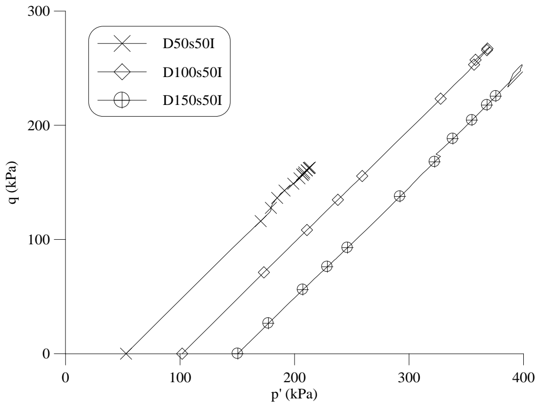
Figura 5.16 – Gráficos p' versus q dos ensaios triaxiais com sucção controlada drenados em corpos de prova indeformados para um nível de sucção de 50 kPa.
