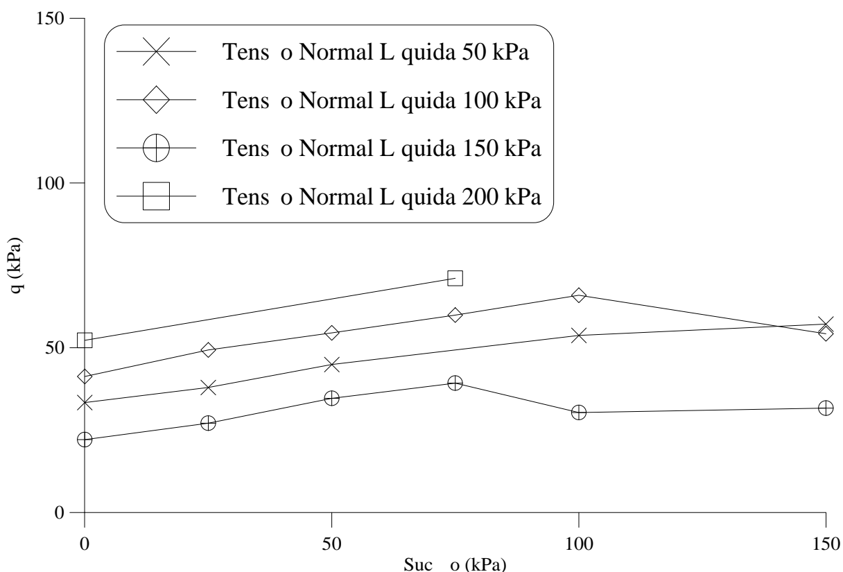
Figura 5.33 – Gráficos q versus sucção dos ensaios triaxiais com sucção controlada drenados em corpos de prova indeformados obtido através do ajuste das curvas tensão versus deformação axial.
