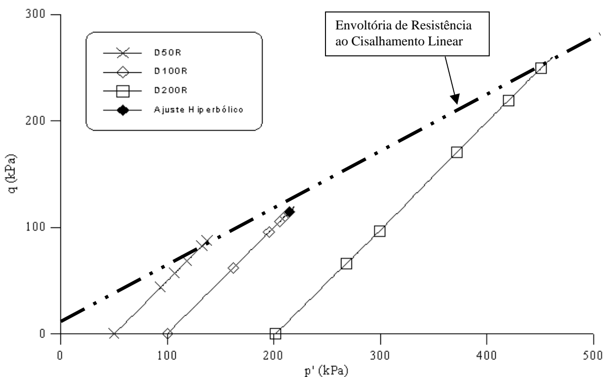
Figura 5.6– Gráfico p' versus q dos ensaios triaxiais convencionais drenados em corpos de prova remoldados do Solo AV .
