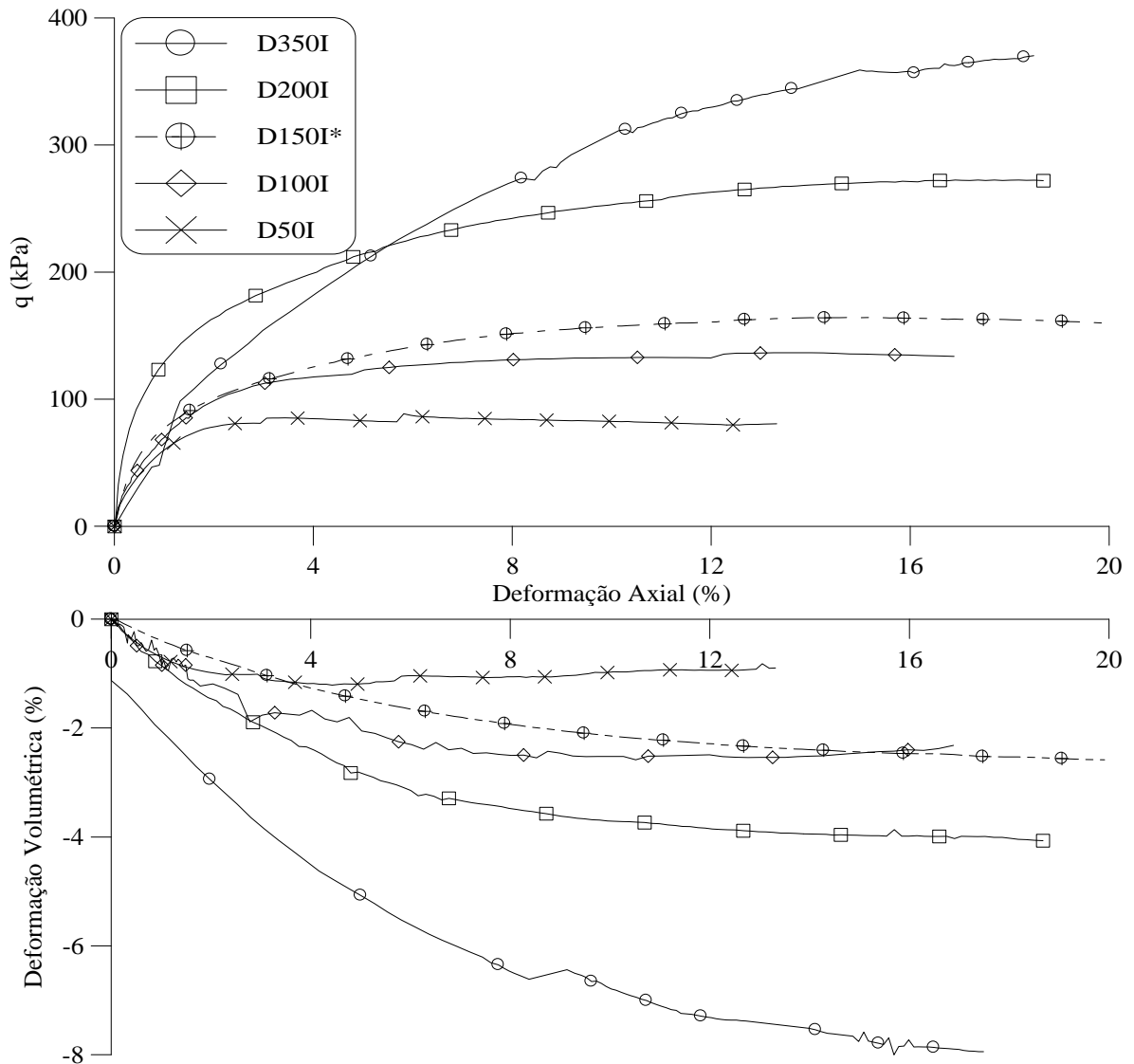
Figura 5.2 – Gráficos q versus \epsilon_a e \epsilon_a versus \epsilon_v do ensaios triaxiais convencionais drenados em corpos de prova indeformados do Solo AV. (*) Ensaio apresentado por Bressani et al. (2005).
