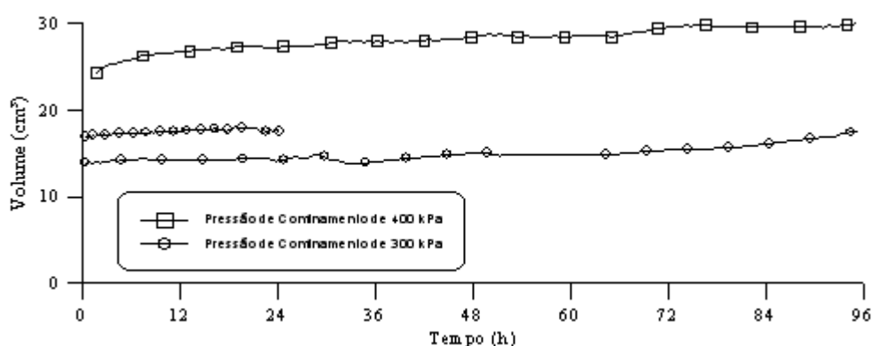
Figura 5.1 – Curvas de calibração para variação volumétrica da câmara triaxial para pressões de confinamento de 300 e 400 kPa.
