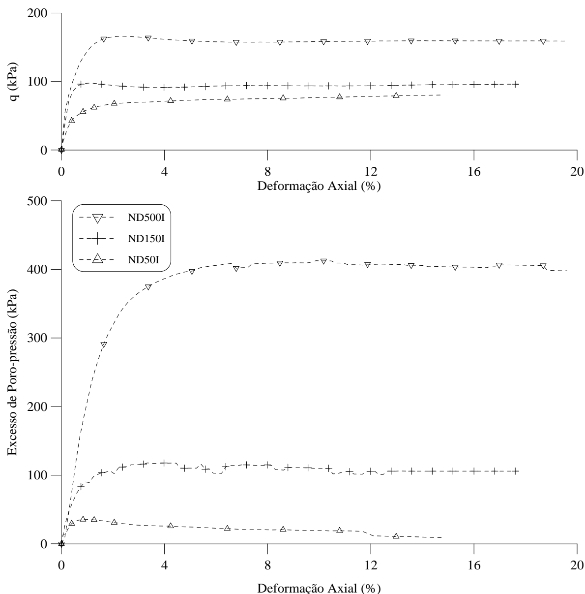
Figura 5.3 – Gráficos q versus \epsilon_a e \epsilon_a versus excesso de poro-pressão dos ensaios triaxiais convencionais não drenados em corpos de prova indeformados do Solo AV
