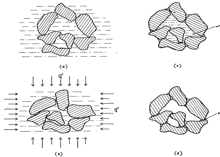
Figura 2.2 – Mudanças estruturais no solo devidas às cargas externas e pressões negativas: (a) partículas em estado natural; (b) partículas sob carga; (c) deslocamentos das partículas devido às forças compreensíveis resultantes do menisco; (d) partículas “unidas” pelas forças do menisco nos contatos dos grãos. (Jennings e Burland, 1962).
