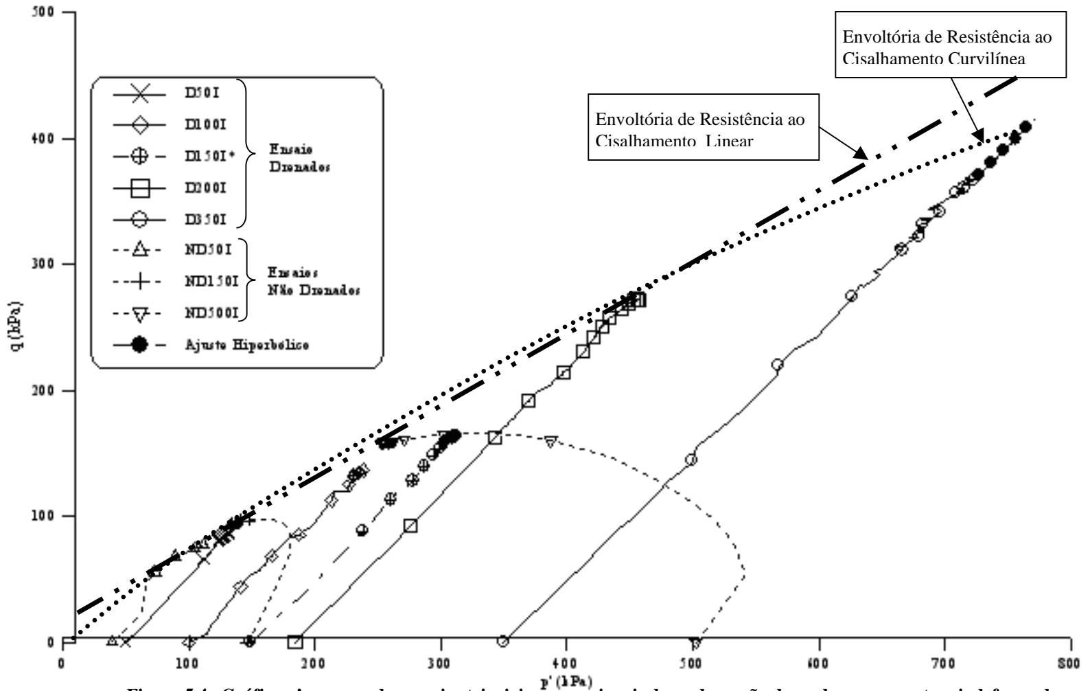
Figura 5.4- Gráfico p' versus q dos ensaios triaxiais convencionais drenados e não drenados em amostras indeformadas do Solo AV. (*) Ensaio realizado por Bressani et al. (2005).
