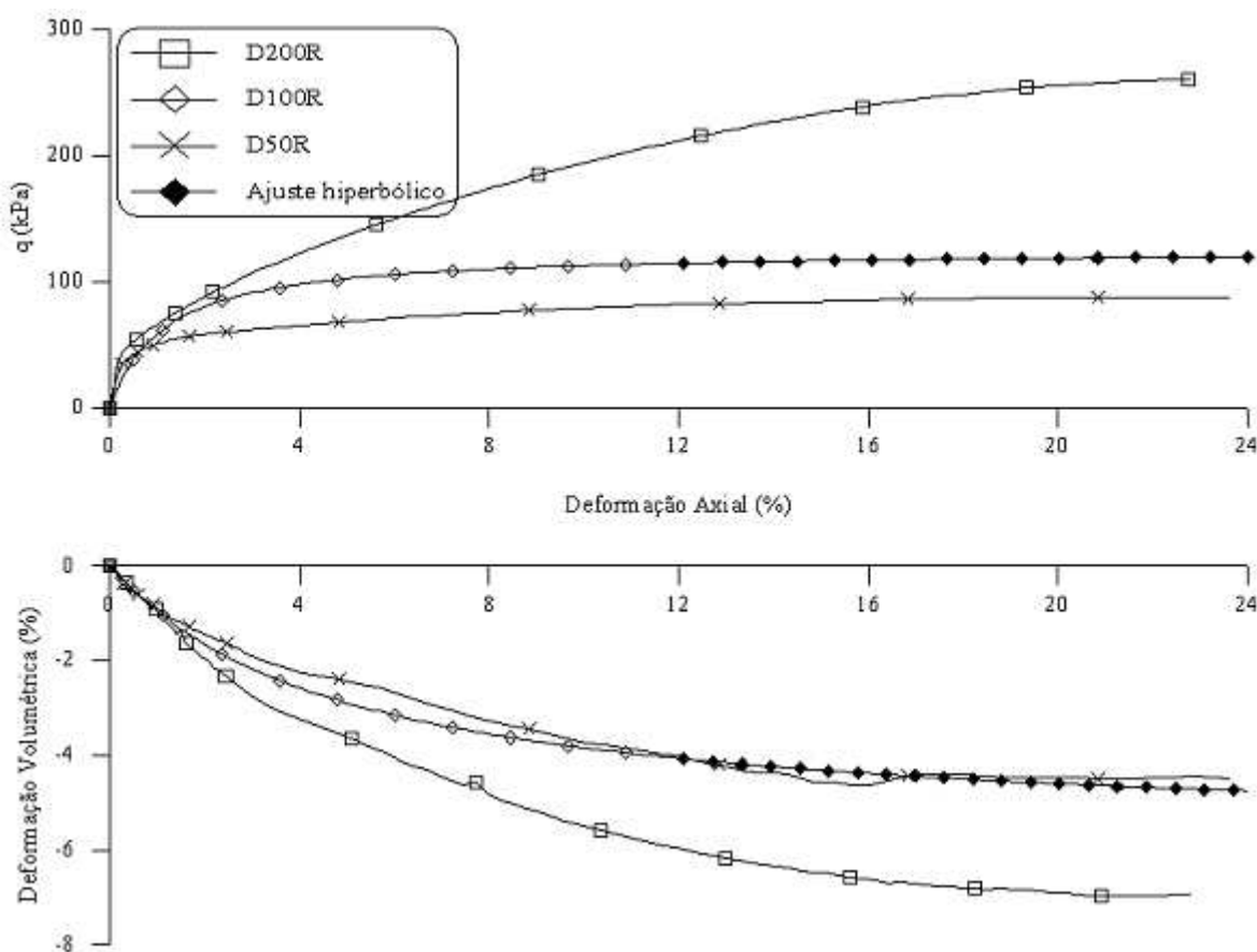
Figura 5.5 – Gráficos q versus \epsilon_a e \epsilon_a versus \epsilon_v do ensaios triaxiais convencionais drenados em corpos de prova remoldados do Solo AV.
