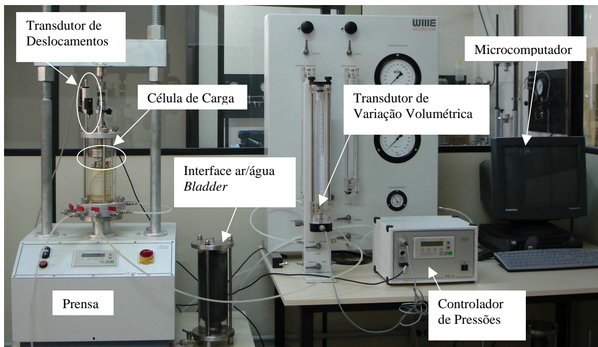
Figura 3.2 – Equipamento de ensaio triaxial para realização de ensaios saturados.
