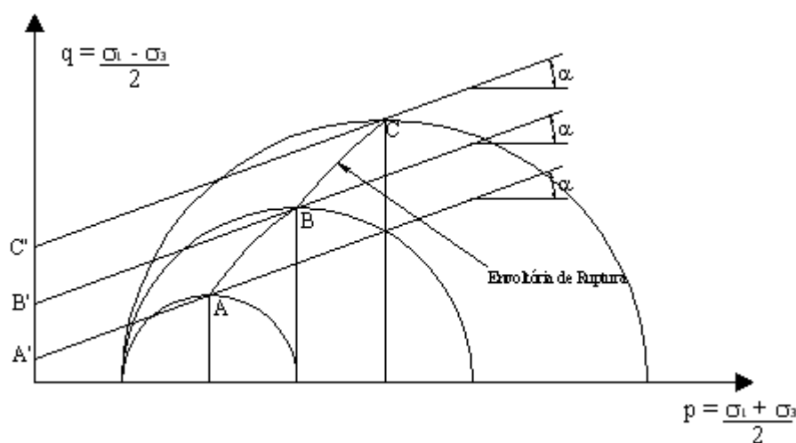
Figura 5.20 – Representação da projeção da envoltória para o plano q versus sucção ( p' igual a zero) dos ensaios triaxiais com sucção controlada (Baseada em Oliveira, 2004).
