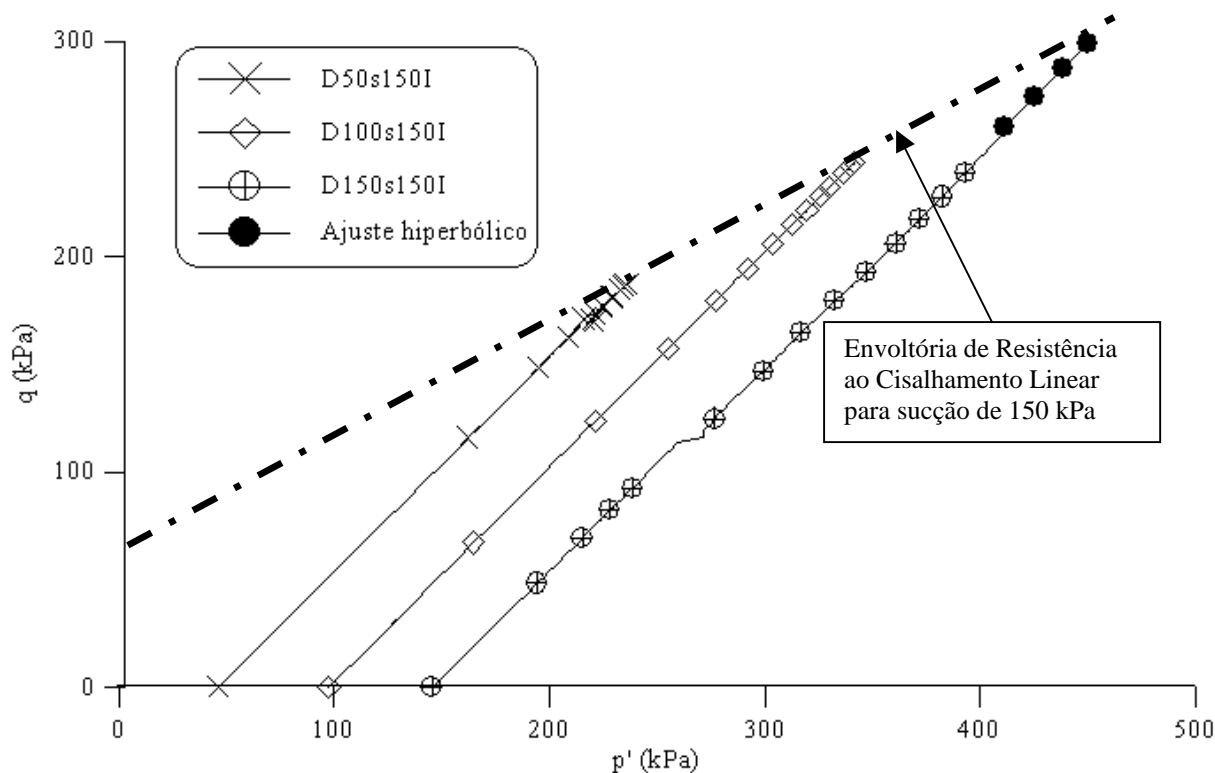
Figura 5.30 – Gráficos p' versus q dos ensaios triaxiais com sucção controlada drenados em corpos de prova indeformados para um nível de sucção de 150 kPa. O ajuste hiperbólico é representado pelo símbolo preenchido.
