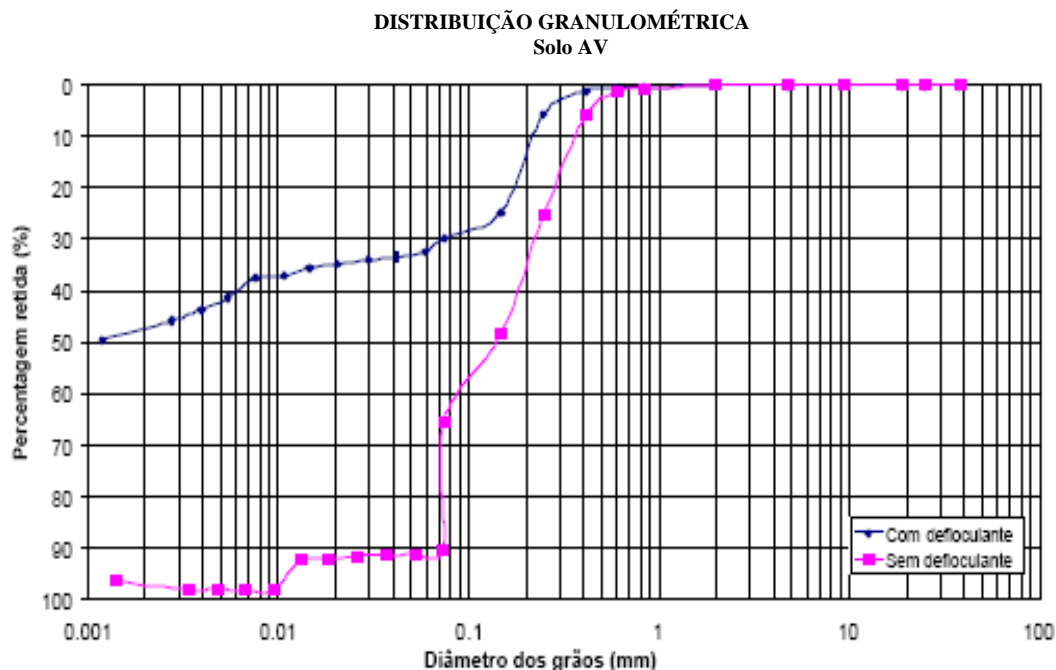
Figura 4.3 – Curva granulométrica do solo coluvionar de arenito, Bloco AV (Feuerharmel, 2003).
