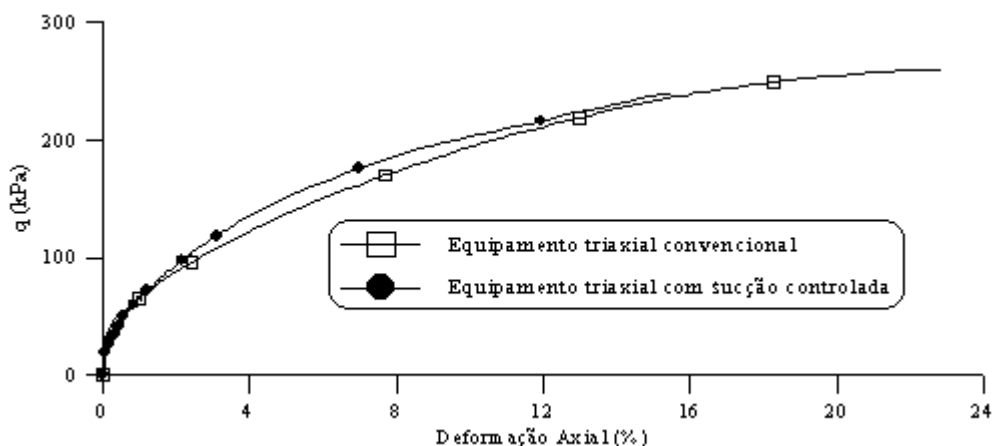
Figura 5.9 – Curvas tensão versus deformação axial para corpos de prova remoldados idênticos, ensaiados na mesma tensão de confinamento efetiva no equipamento triaxial convencional e no equipamento com sucção controlada.
