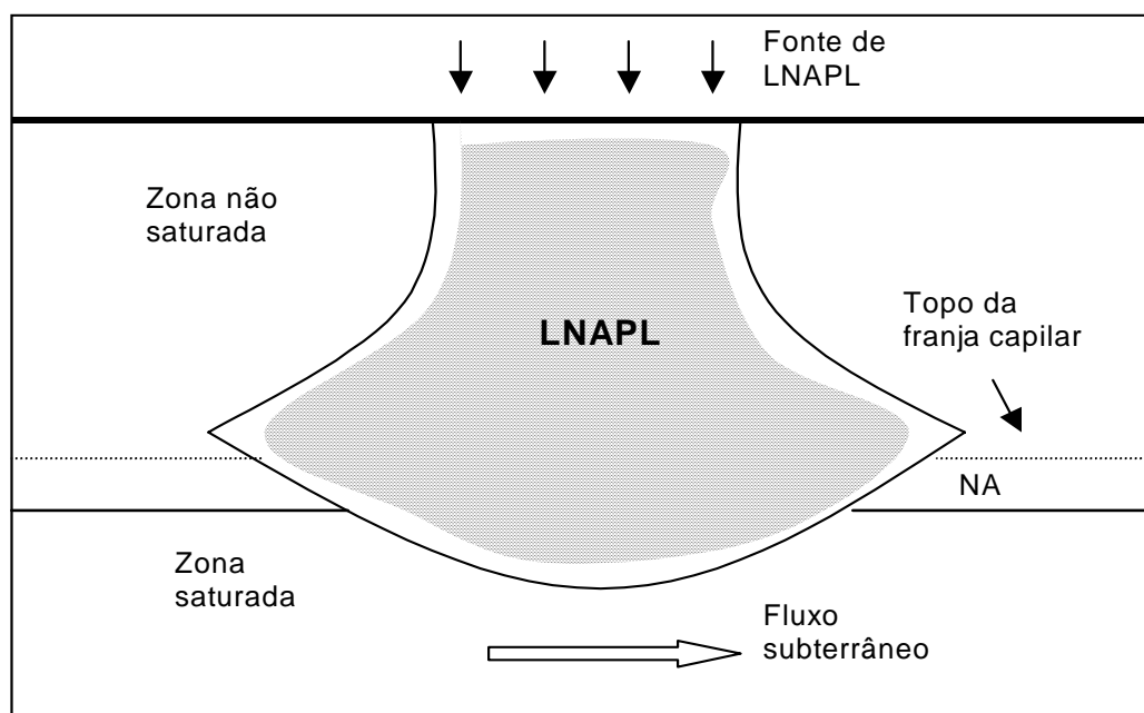
Figura 2.4: deformação da linha do nível d'água resultante de um grande suprimento de LNAPL (fonte: Hasan, 1996)
