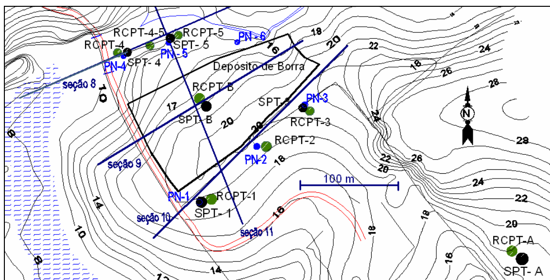
Figura 4.13: posição dos ensaios de cone resistivo na área investigada
