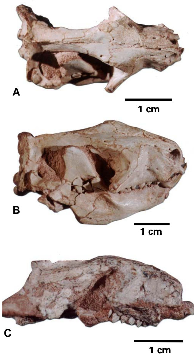
Figura 17 – Exemplos de Riorandia guuibensis , PV0596T, em vista dorsal (A) e lateral (B), e PV0601T, em vista lateral (C).
