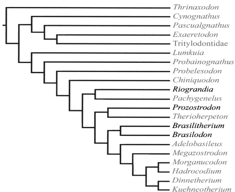
Figura 9 - Cladograma mostrando posição filogenética de Prozostrodon , Riograndia , Brasilodon e Brasilitherium (retirado de Bonaparte et al. , 2005).
