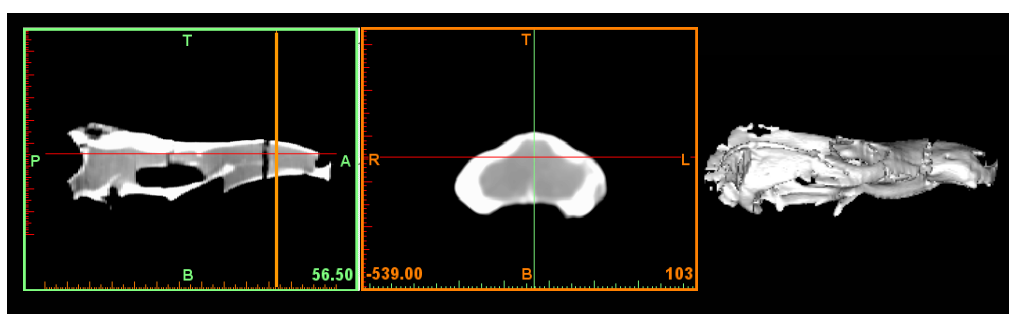
Figura 20 – Imagens bidimensionais de tomografias computadorizadas em plano sagital (à esquerda) e coronal (no centro), e vista lateral da reconstituição 3D (à direita) do crânio de Massetognathus (PV0968T). A linha laranja mostra a posição em vista sagital do plano de corte mostrado ao centro, o qual corresponde à secção transversal da porção respiratória da cavidade nasal. O material rochoso que preenche as cavidades cranianas aparece em cinza. Este exemplar está quebrado na metade do focinho.
