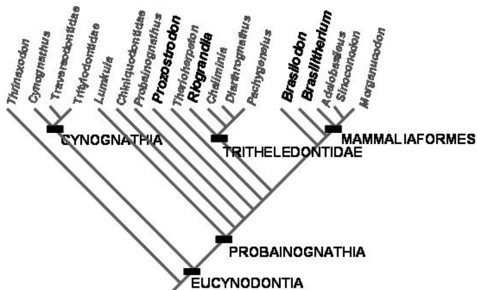
Figura 8 - Cladograma mostrando a posição filogenética de Prozostrodon , Riograndia , Brasilodon e Brasilitherium (retirado de soares, 2004).
