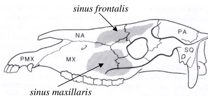
Figura 27 - Representação dos seios paranasais em Equus (modificado de Novacek, 1993)
