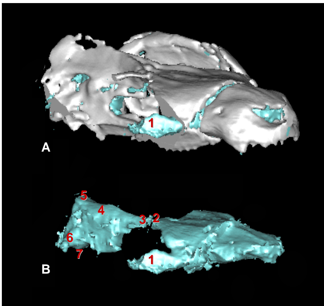
Figura 29 – Reconstituição tridimensional a partir das tomografias do crânio de Massetognathus PV0968T sem o arco zigomático do lado direito (A), e sem os elementos ósseos (representados na cor prata), mostrando um molde interno virtual equivalente à da matriz rochosa (em azul) que preenche as cavidades cranianas (B).
