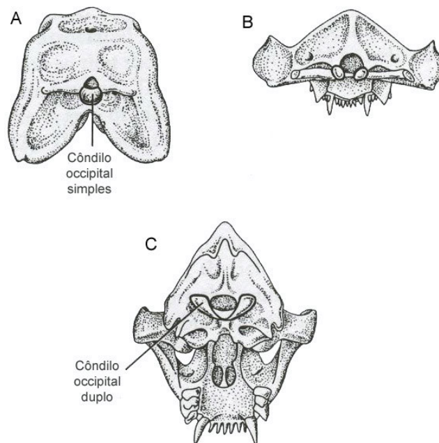
Figura 20: Alterações na articulação crânio/região cervical. A , pelicossauro com cômulo occipital simples. B , cinodonte não-mamaliano com cômulo occipital duplo. C , mamífero com cômulo occipital duplo. Modificado de Carroll (1988).
