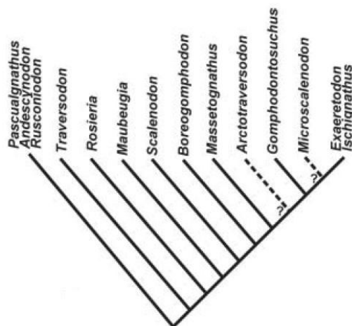
Figura 15: Hipótese filogenética sobre as relações entre os traversodontídeos. Retirado de Godefroit e Battail (1997).
