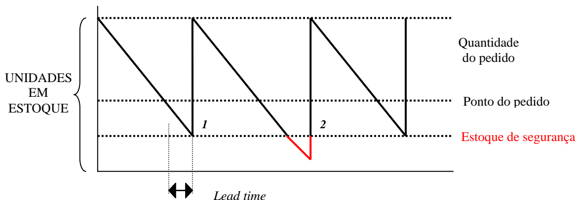
Figura 9- Estoque de segurança
