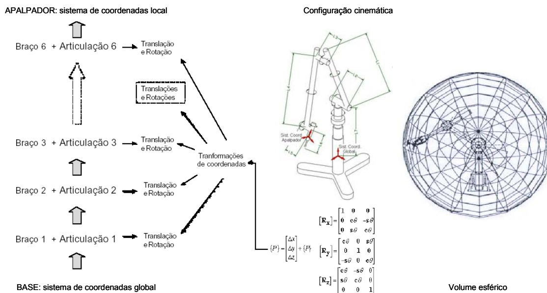
Figura 8 – Transformações de coordenadas e volume de trabalho de um braço articulado de medição [27] .
