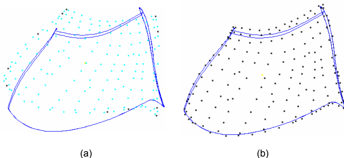
Figura 41 – Pá Francis com a: (a) malha de pontos (cor verde) alinhada de uma maneira incorreta ao modelo em CAD (cor azul) e (b) malha de pontos alinhada corretamente.
