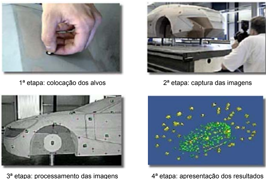
Figura 22 – Fluxo de trabalho do sistema fotogramétrico TRITOP [36] .
