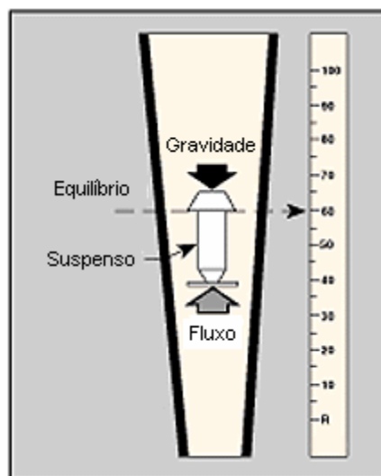
Figura 8 – Rotâmetro
