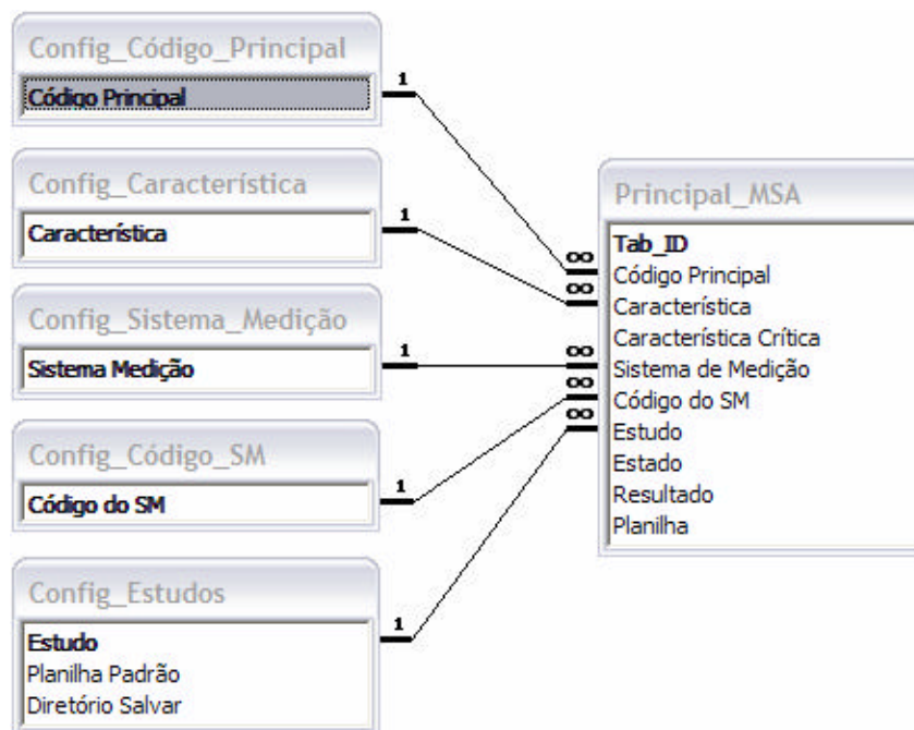
Figura 4.9 – Relacionamento da base de dados do Gerenciador de Documentos – MSA[27]
