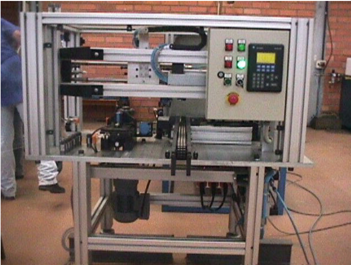
Figura 4.12 – Máquina de Medição de perfil do pinhão
