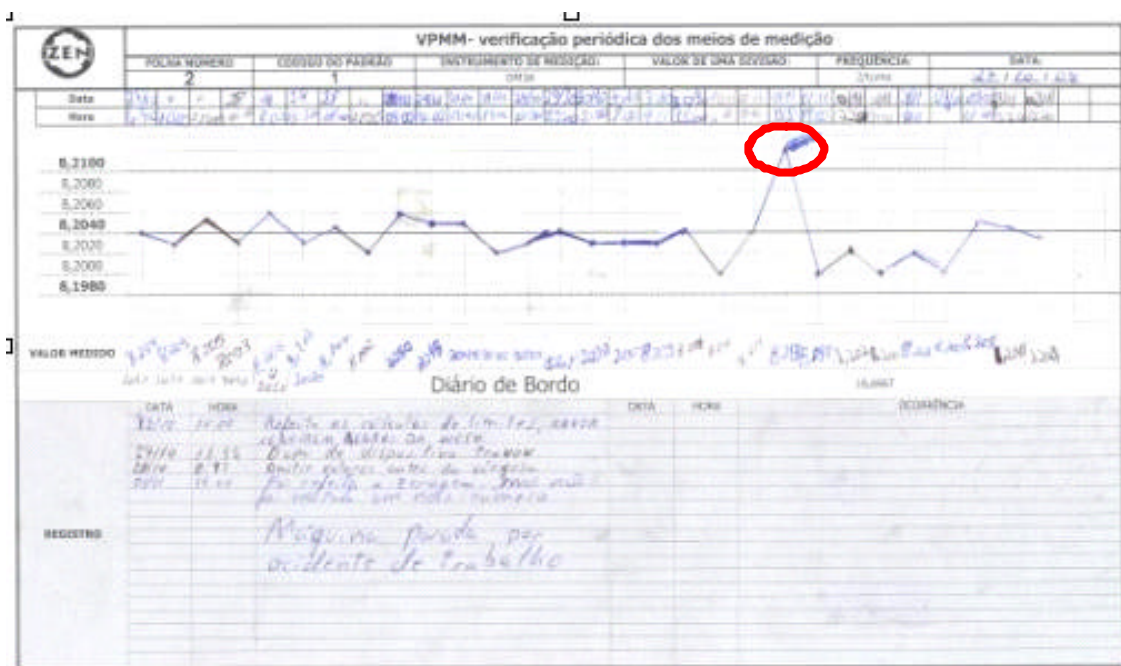
Figura 4.13 – Carta de Controle com ponto fora de controle
