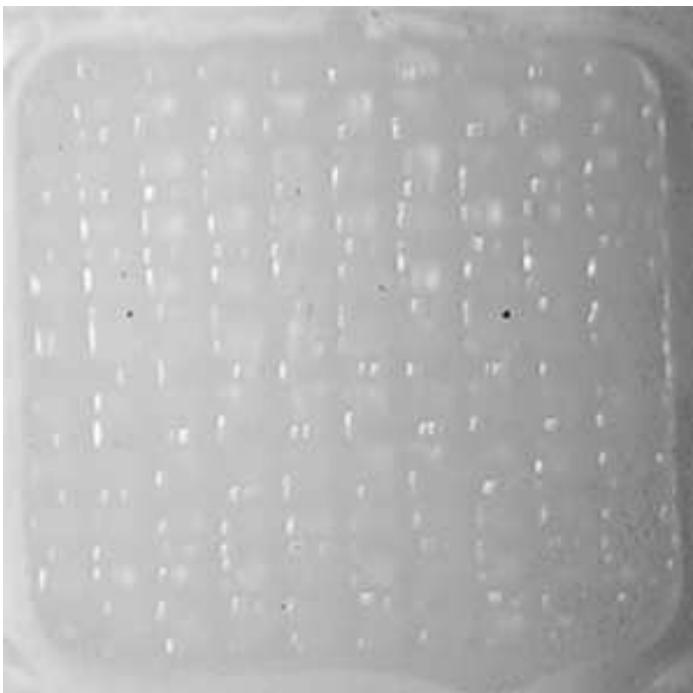
Figura 14 - Fratura coesiva no corpo-de-prova 10 que foi colado com o Sistema adesivo autocondicionante Transbond Plus Self Etching Primer (3M, Unitek) + Resina Z-100 (3M cor B-3
