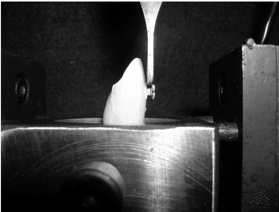
Figura – 10 Detalhe do teste de resistência ao cisalhamento realizado em máquina de ensaio universal (Versat 2000, Pantec, Panambra)
