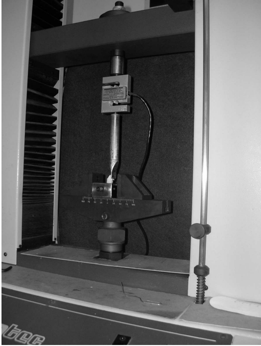
Figura 9 - Corpo-de-prova posicionado na máquina de ensaio universal (Versat 2000, Pantec, Panambra)
