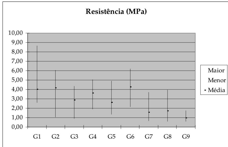
Figura 16 - Gráfico representativo dos valores maiores, menores e das médias da resistência ao cisalhamento (Mpa) de três diferentes adesivos autocondicionantes com e sem contaminação com saliva artificial
