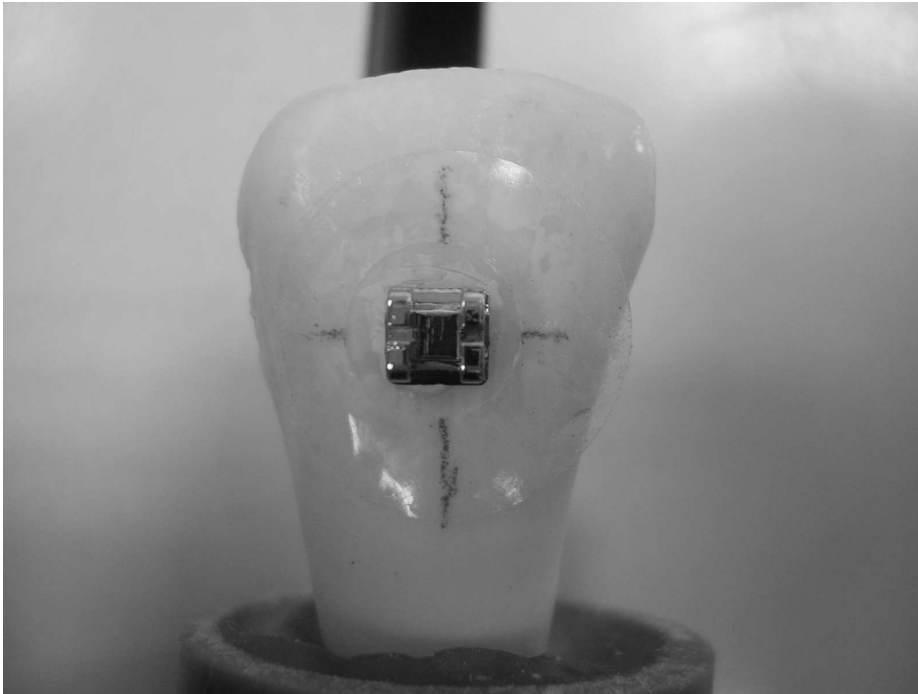
Figura 6 - Corpo-de-prova marcado, com o adesivo plástico e com o braquete colado
