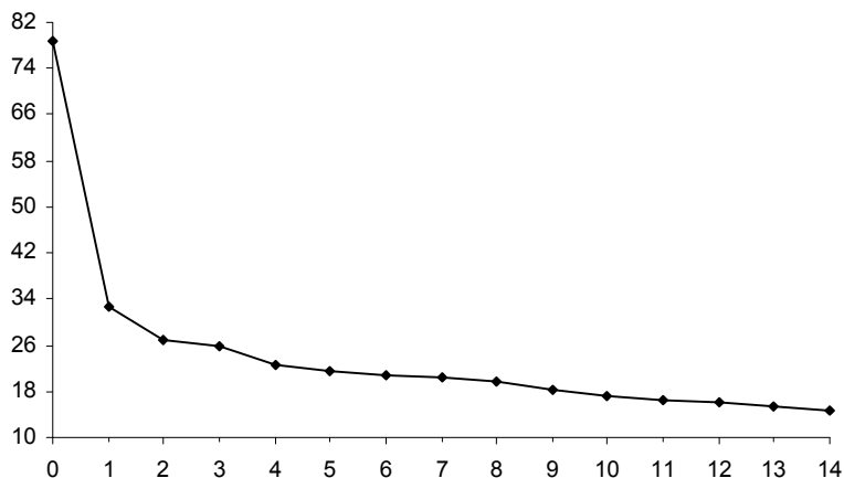
Figura 5. Índice de solubilidade da proteína (%) para os grãos de soja durante o tratamento térmico.
