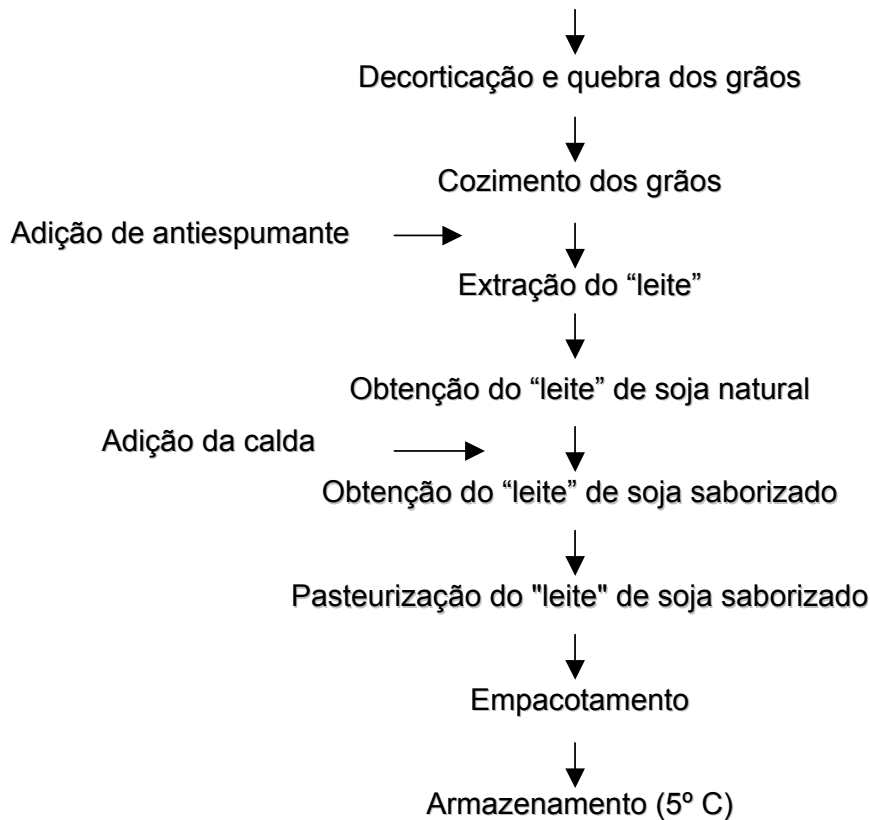
Figura 1. Seqüência tecnológica para a obtenção do "leite" de soja pela Unisoja.
