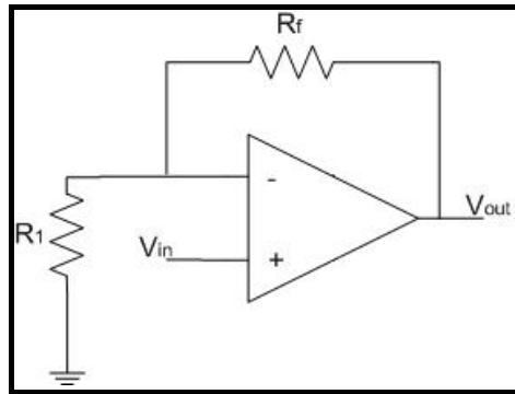
Figura 3.10 - Configuração Amplificador Não-Inversor.
