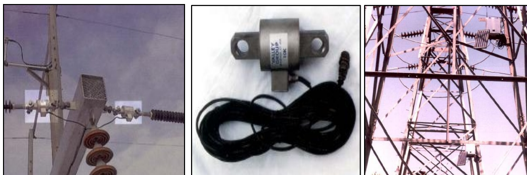
Figura 2.2 – Ilustração da Célula de Carga e Unidade Principal do Sistema CAT-1.
