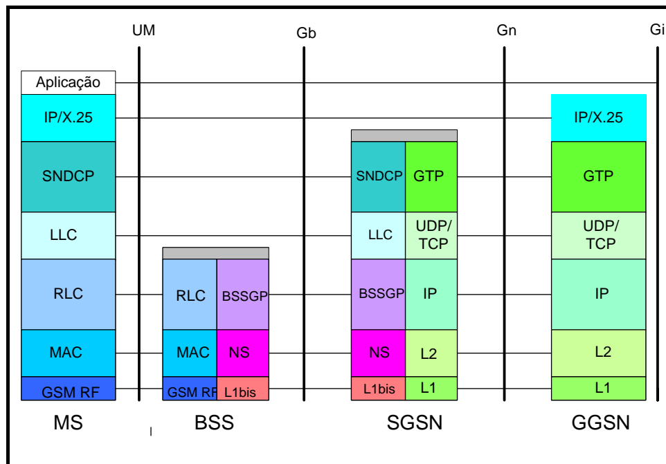
Figura 5.5 - Estrutura e Camadas de Protocolos do GPRS [24]
