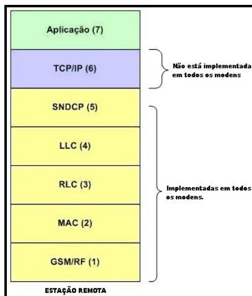
Figura 6.1 - Camadas de Protocolo da Estação Remota.
