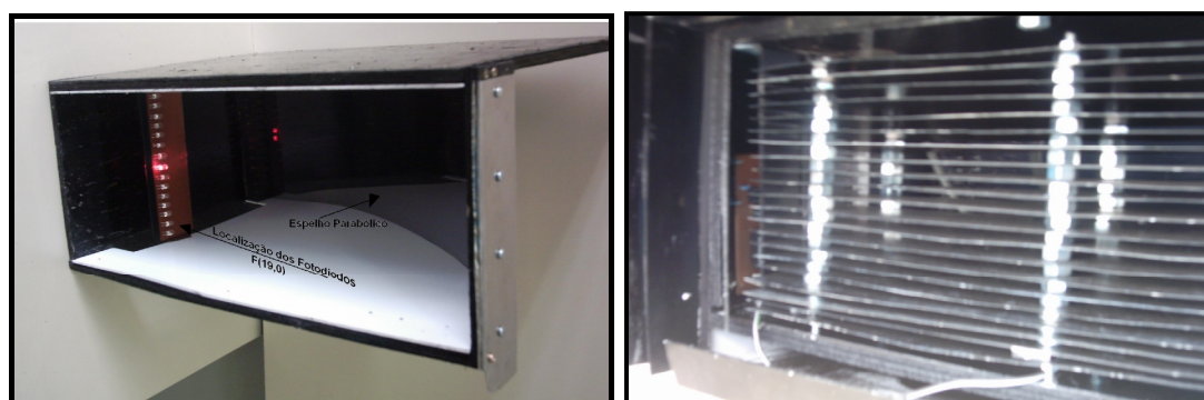
Figura 4.4 - Fotografia da Estrutura Sensora do Protótipo Utilizado no Projeto.
