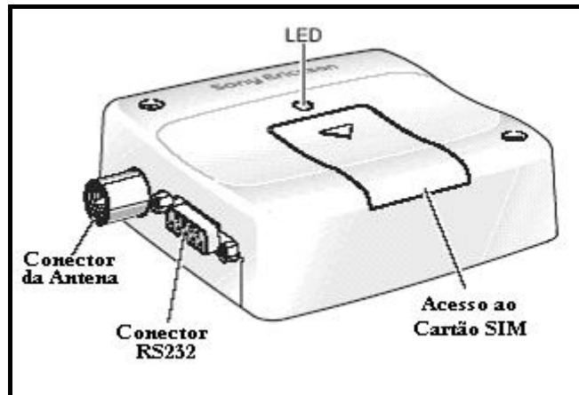
Figura 6.2 – Modem GM29 da Sony-Ericsson.
