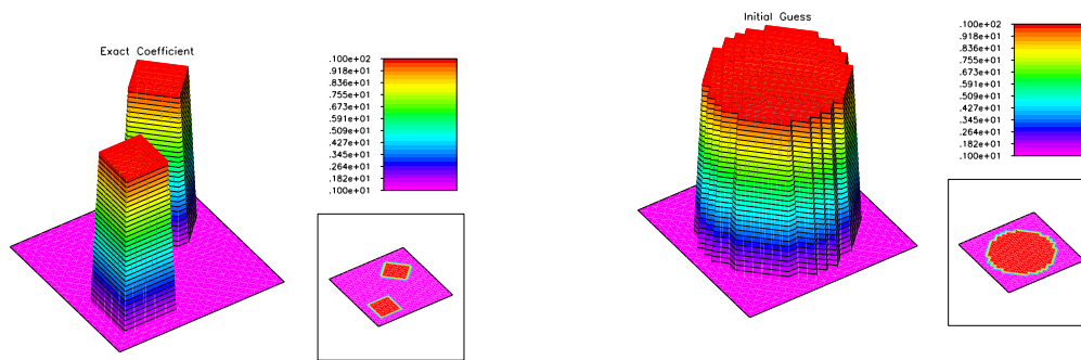
Figura 4.2: Condição inicial para o método de regularização pelo método level set
