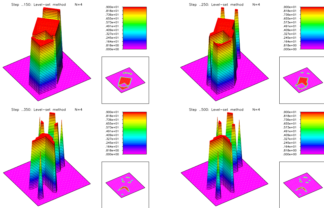
Figura 4.4: Evolução da iteração do erro para dados livres de ruídos
