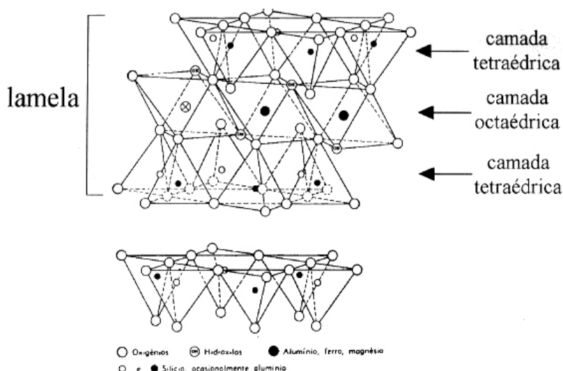
Figura 2.3 - Representação esquemática da estrutura de uma esmectita dioctaédrica que é muito semelhante à estrutura da vermiculita (Aranha et al., 2002).
