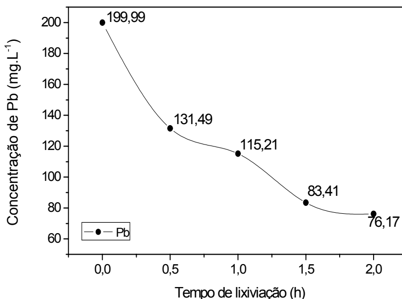
Figura 4.19 – Efeito do tempo de lixiviação sobre a dessorção de \text{Pb}^{2+} , empregando-se vermiculita modificada com NaCl saturada com 200 \text{ mg.L}^{-1} de Pb. Solução lixiviante de acetato de amônio a 1N.
