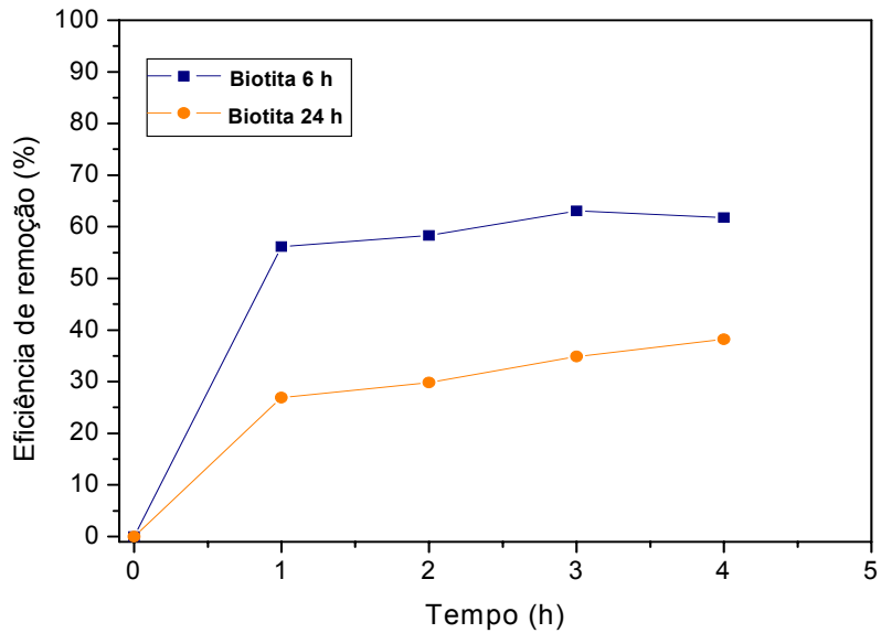
Figura 4.8 – Eficiência de remoção de Pb^{2+} em função do tempo de percolação, empregando-se biotita tratada a 6 e 24 horas. Concentração inicial de Pb = 100 \text{ mg.L}^{-1} ; pH 4,5; granulometria de (-0,2+0,074)\text{mm} .
