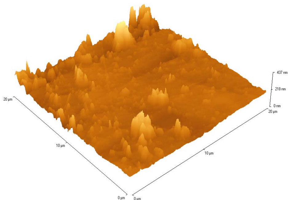
Figura 4.3 – Micrografia, de imagem tridimensional de parte de uma placa de vermiculita no modo de contato, após a adsorção com o metal, obtida em MFA e recursos de análise de imagem.
