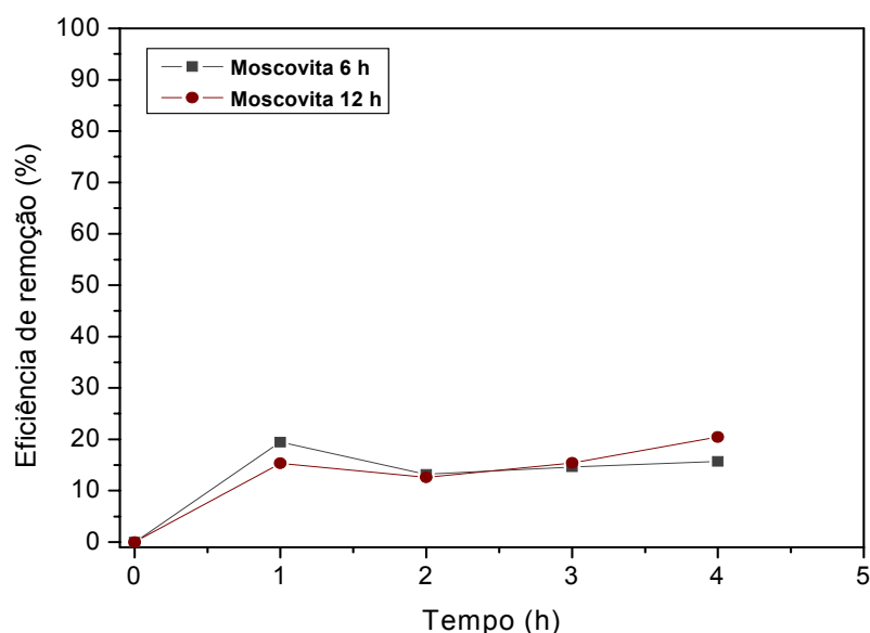
Figura 4.10 - Eficiência de remoção de Pb^{2+} em função do tempo de percolação, empregando-se moscovita tratada a 6 e 24 horas. Concentração inicial de Pb = 100 \text{ mg.L}^{-1} ; pH 4,5; granulometria de (-0,3+0,5)mm.
