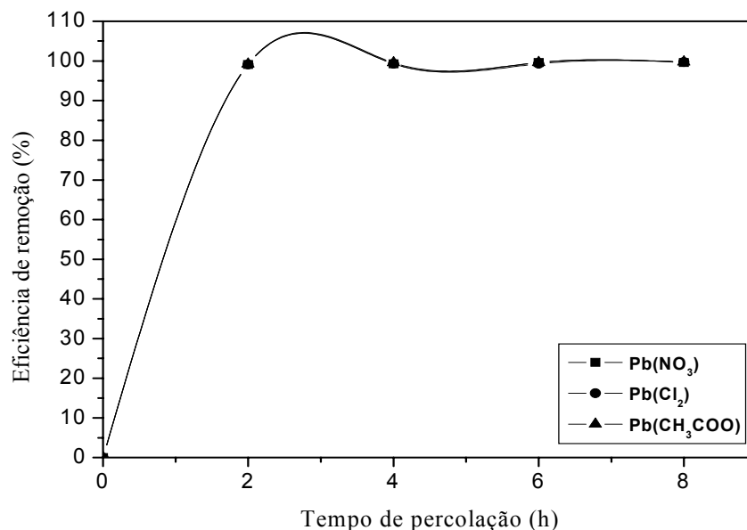
Figura 4.17 – Eficiência de remoção do Pb 2+ em função do tempo de percolação e do tipo de ânion associado ao metal, empregando-se vermiculita modificada com NaCl. Concentração inicial de Pb de 100 mg.L -1 ; pH 4,5.
