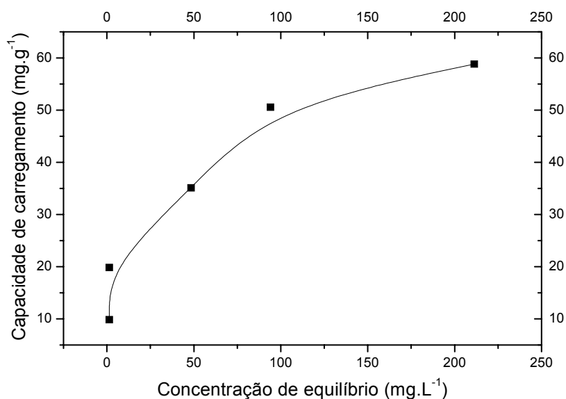
Figura 4.15 – Efeito da concentração de equilíbrio sobre a C_c de Pb empregando-se vermic-NaCl. Tempo de percolação de 2h; pH 4,5 e temperatura de 25 °C.
