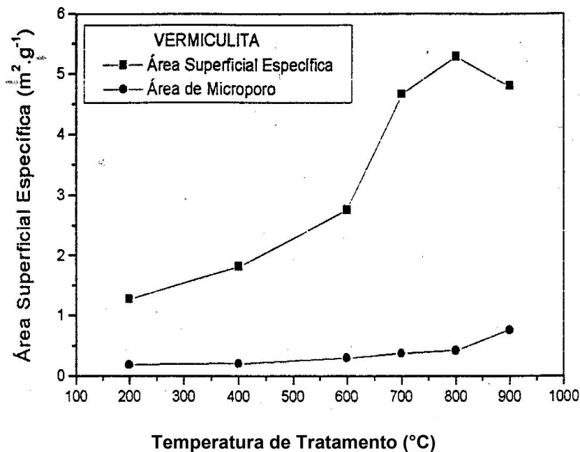
Figura 4.1 – Efeito da temperatura de tratamento térmico sobre a área superficial específica e área de microporos da vermiculita.
