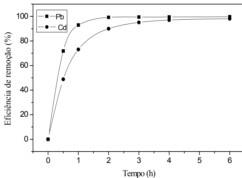
Figura 4.12 – Eficiência de remoção de Pb^{2+} e Cd^{2+} em função do tempo de percolação, empregando-se vermiculita modificada com NaCl. Concentração inicial do metal de 200 \text{ mg.L}^{-1} ; pH 4,5.
