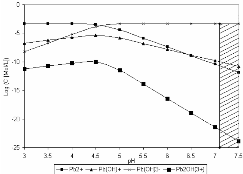
Figura 4.14 – Diagrama de especiação de Pb 2+ , em meio aquoso, 100 mgL -1 . A área listrada representa a formação da espécie neutra Pb(OH) 2 (Montes et al., 2004; Valdiviezo et al., 2004).
