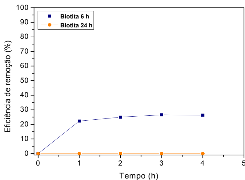
Figura 4.9 - Eficiência de remoção de \text{Cd}^{2+} em função do tempo de percolação, empregando-se biotita tratada a 6 e 24 horas. Concentração inicial de \text{Cd} = 100 \text{ mg.L}^{-1} ; pH 4,5; granulometria de (-0,2+0,074)\text{mm} .
