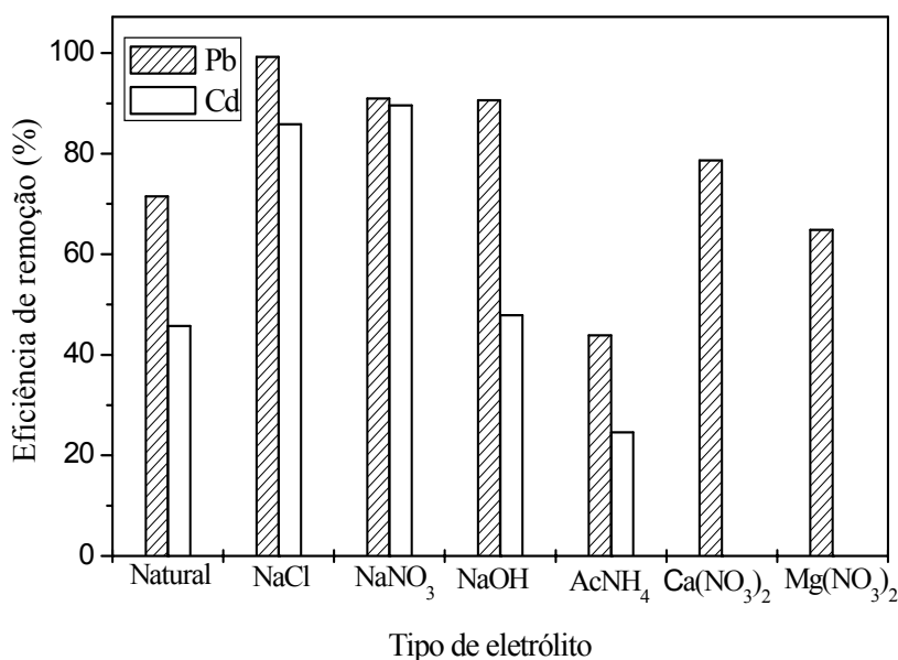
Figura 4.11 – Eficiência de remoção de \text{Pb}^{2+} e \text{Cd}^{2+} em função do tipo de sal intercalado com a vermiculita. Concentração inicial do metal de 200 \text{ mg.L}^{-1} ; pH 4,5; tempo de percolação de 2 horas.
