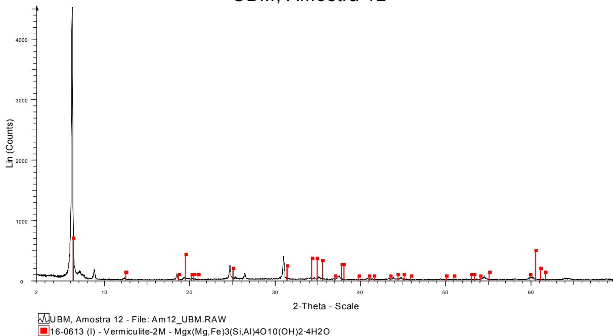
Figura 4.4 - Difratoograma de raios-x de uma amostra de vermiculita de Santa Luzia - PB, com intervalo de varredura de 2° a 70°. O nome UBM, amostra 12, foi usado para identificação.
