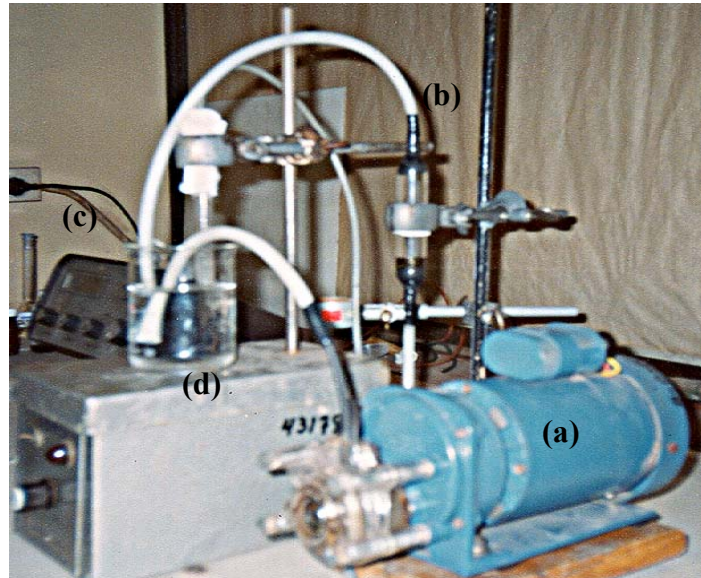
Figura 3.2 - Esquema do arranjo da coluna de percolação com seus acessórios usados nos ensaios de adsorção. (a) bomba peristáltica; (b) coluna de percolação; (c) pH-metro e (d) reator de vidro contendo o efluente líquido.
