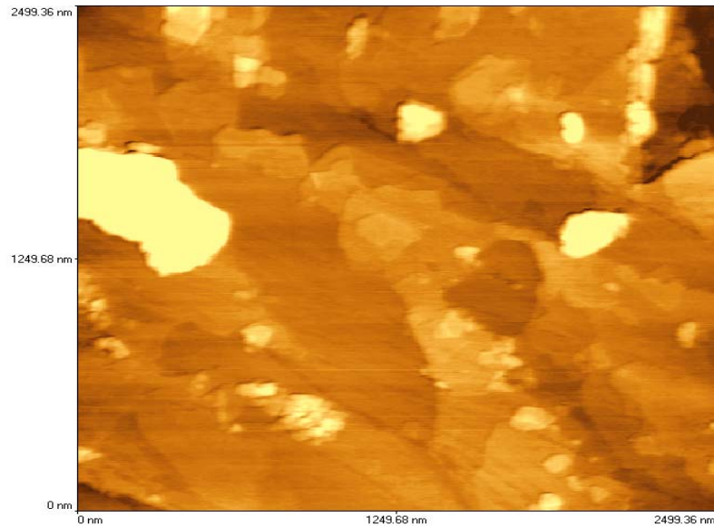
Figura 4.2 – Micrografia, com imagem tridimensional de parte de uma placa de vermiculita no modo de contato, depois da adsorção com o metal, obtida no MFA.
