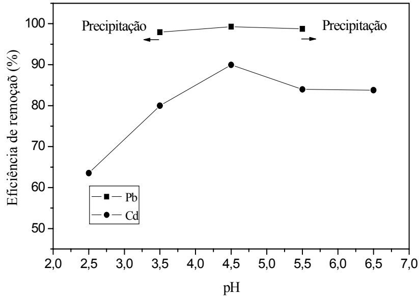
Figura 4.13 - Eficiência de remoção de Pb 2+ e Cd 2+ em função do pH, empregando-se vermiculita modificada com NaCl. Concentração inicial do metal de 200 mg.L -1 , tempo de percolação de 2 horas.
