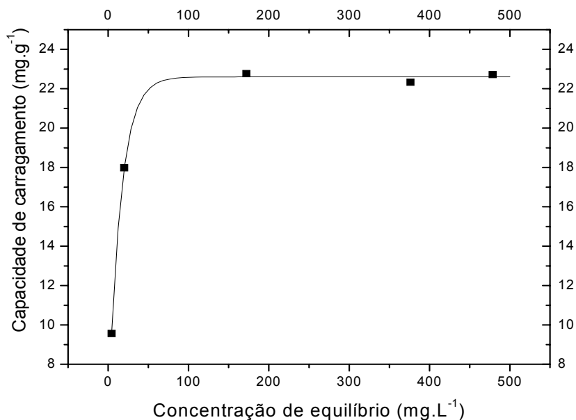
Figura 4.16 – Efeito da concentração de equilíbrio sobre a C_c de Cd empregando-se vermiculita. Tempo de percolação de 2h; pH 4,5 e temperatura de 25 °C.
