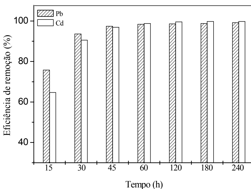
Figura 4.18 – Efeito competitivo de \text{Pb}^{2+} e \text{Cd}^{2+} sobre a eficiência de remoção, empregando-se vermiculita modificada com NaCl. Concentração inicial de Pb de 50 \text{ mg.L}^{-1} ; concentração inicial de Cd de 50 \text{ mg.L}^{-1} ; pH 4,5.
