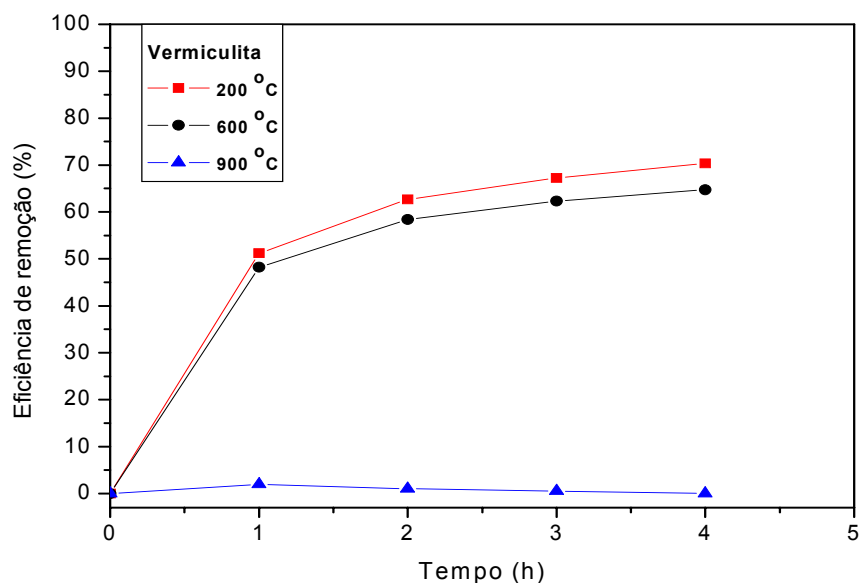
Figura 4.7 – Eficiência de remoção de \text{Cd}^{2+} em função do tempo de percolação, empregando-se vermiculita tratada a diferentes temperaturas. Concentração inicial de \text{Cd} = 100 \text{ mg.L}^{-1} ; pH 4,5; granulometria de (-0,5+0,3)\text{mm} .
