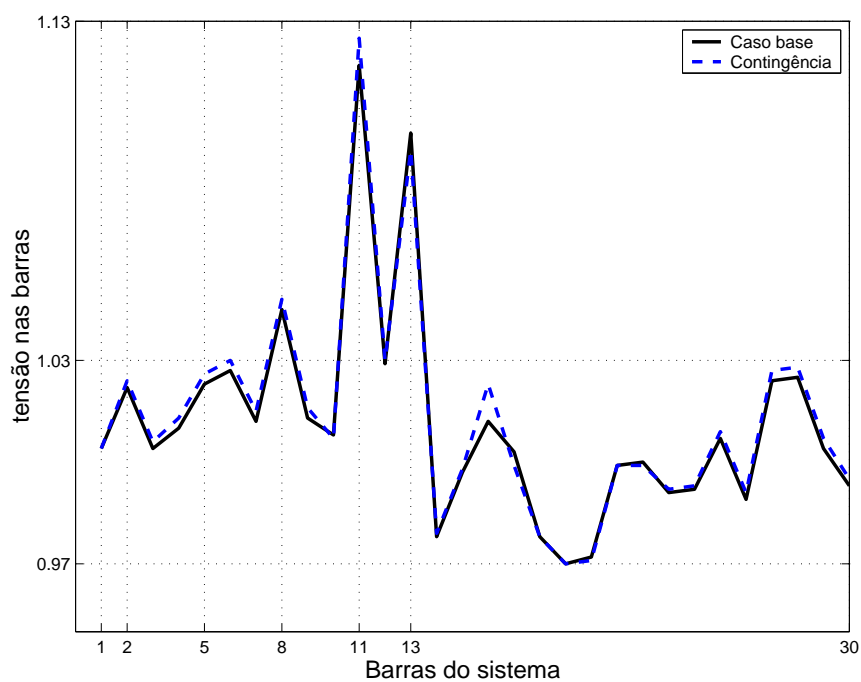
Figura 4.11: Tensão das barras no cenário S1 - sistema IEEE 30-barras
