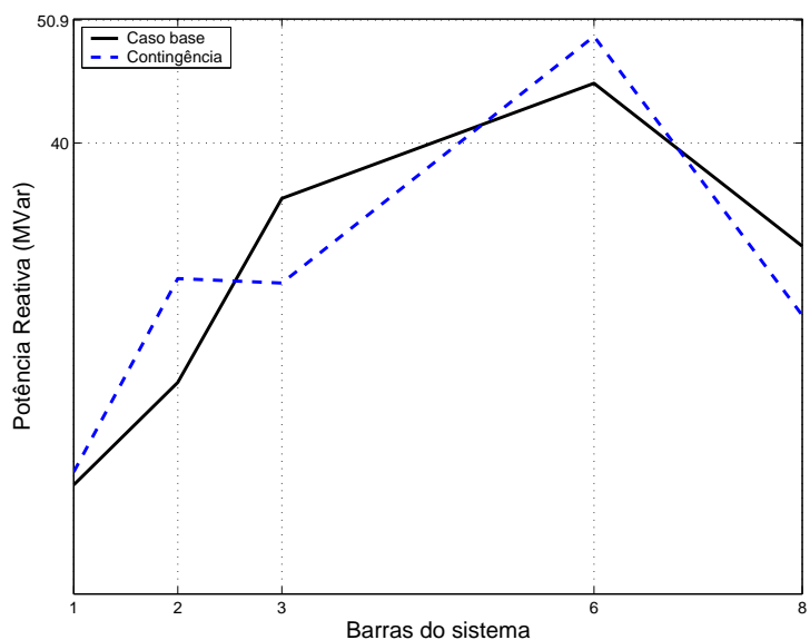
Figura 4.6: Reativos dos geradores no cenário S1 sistema IEEE 14-barras: caso base e contingência
