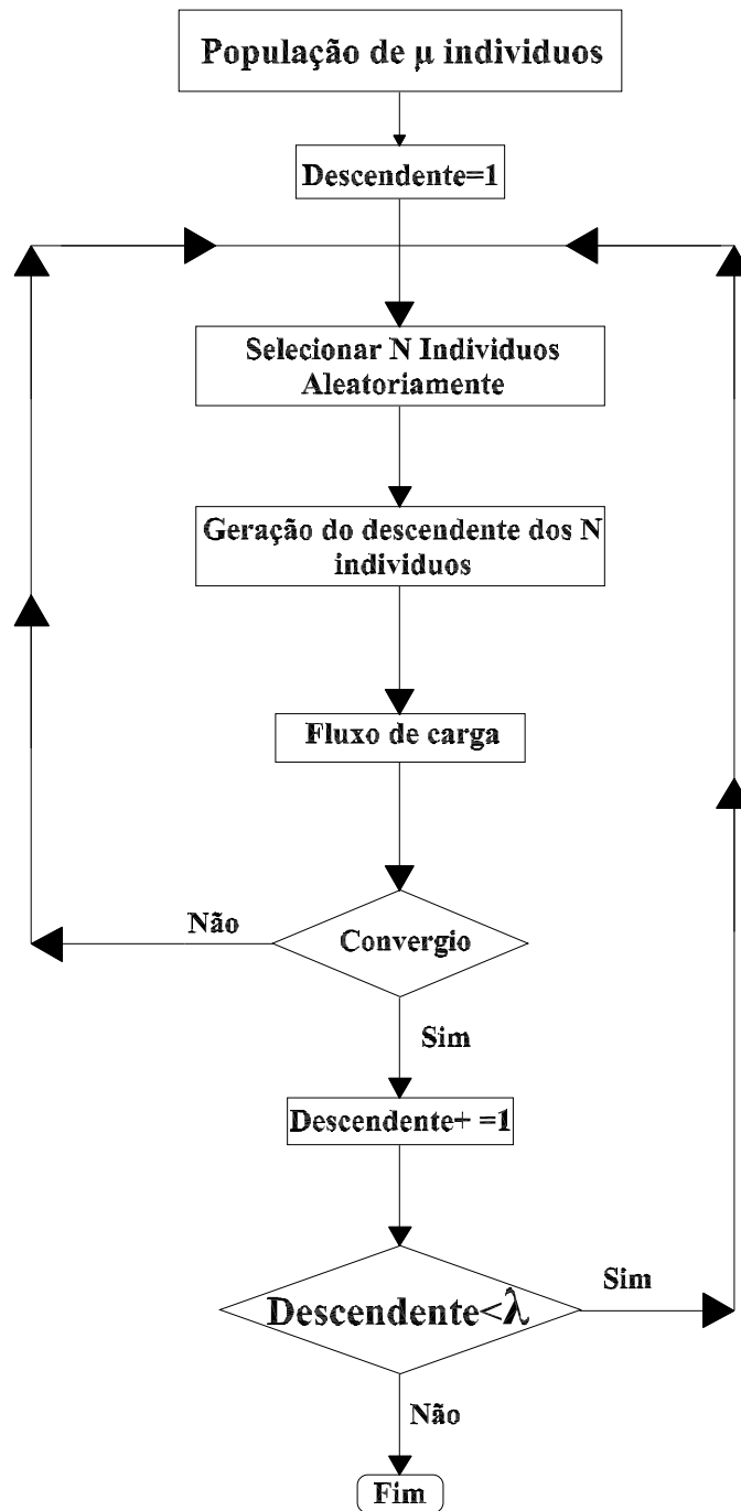
Figura 3.7: Fluxograma da recombinação
