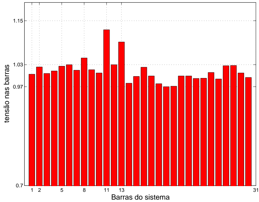
Figura 4.10: Tensão das barras no cenário S1 sistema IEEE 30-barras: caso contingência
