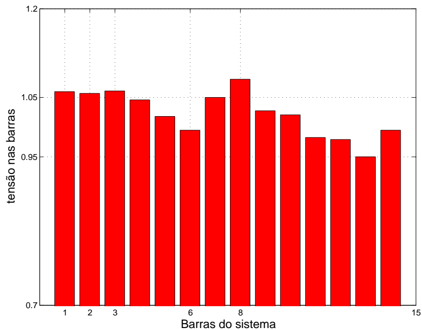
Figura 4.4: Tensão das barras no cenário S1 sistema IEEE 14-barras: caso contingência
