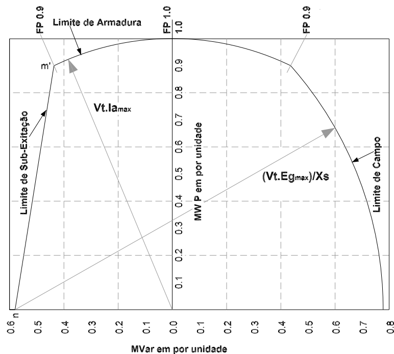
Figura 2.1: Diagrama de Capacidade de um Gerador de 635 MVA
