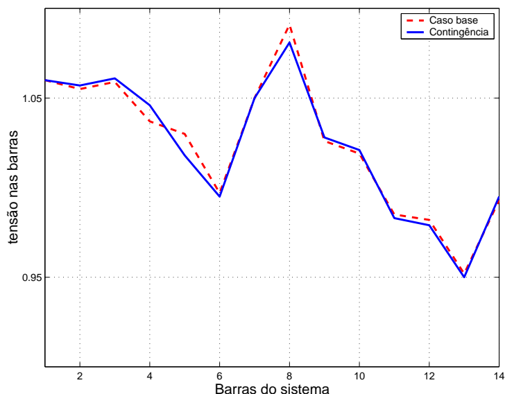
Figura 4.5: Tensão das barras no cenário S1 sistema IEEE 14-barras: caso base e contingência
