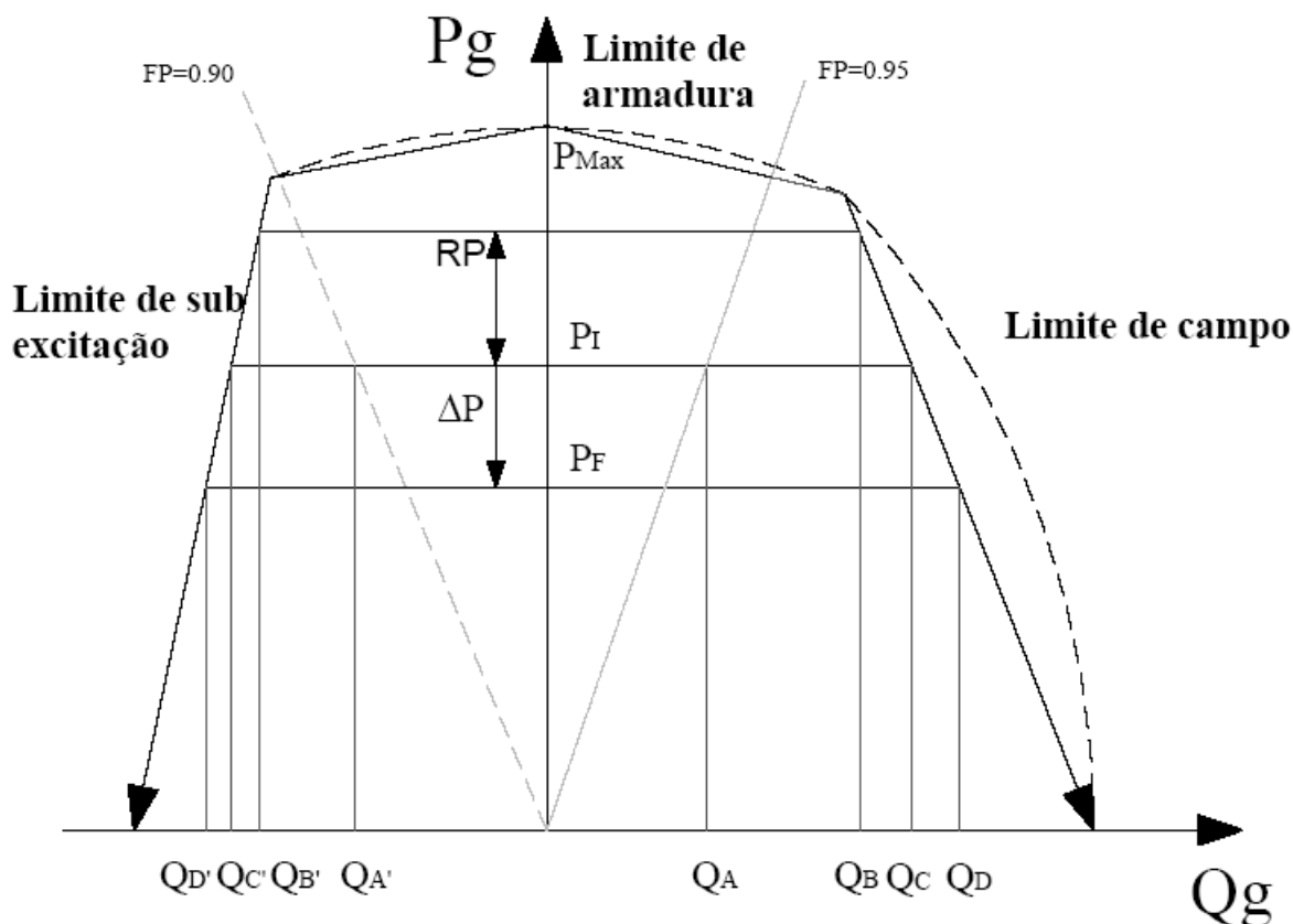
Figura 3.2: Curva de Capacidade do Gerador
