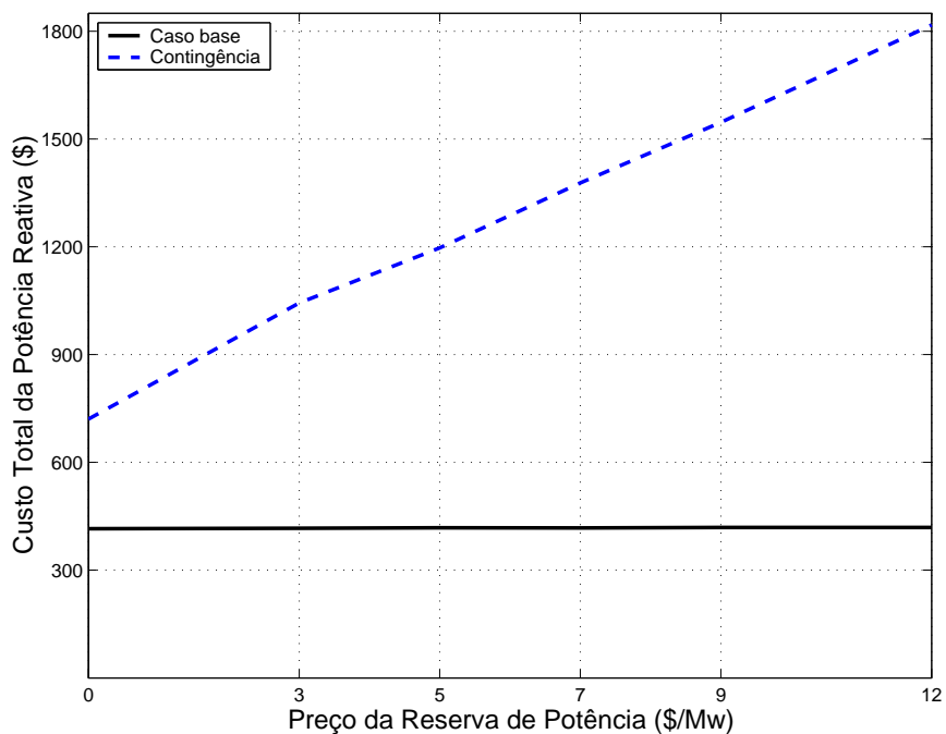
Figura 4.12: Custo total de Potência Reativa no sistema IEEE 30-barras: caso base e contingência
