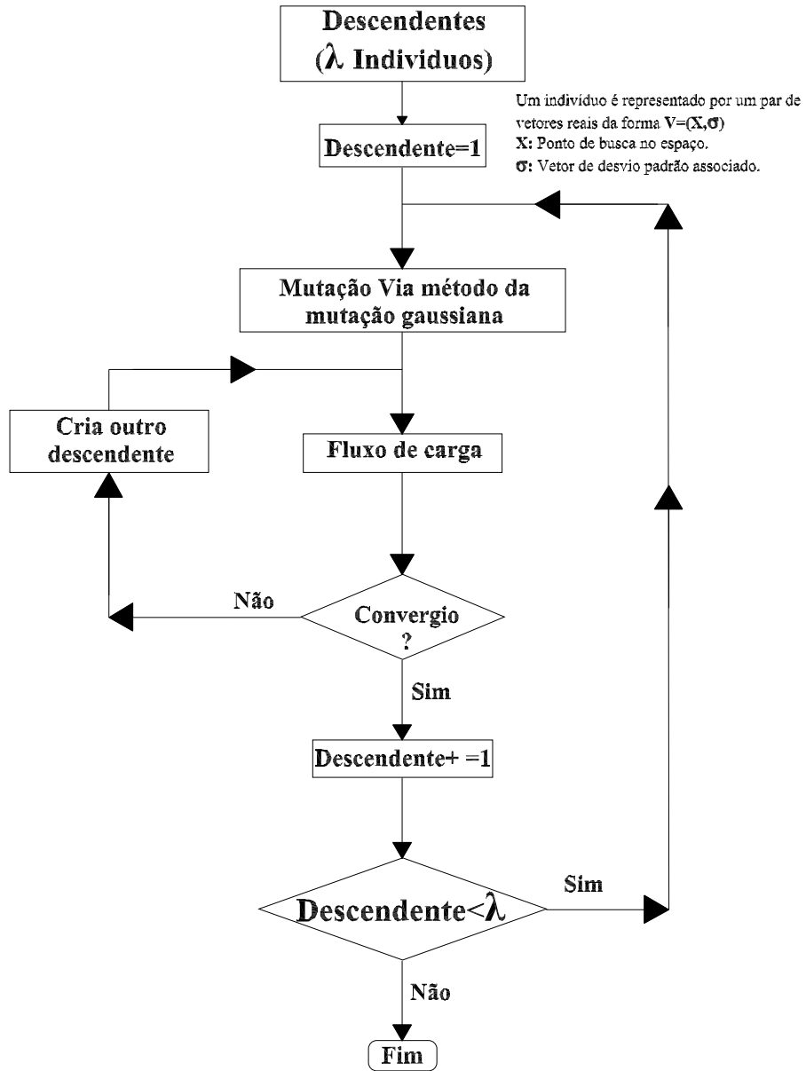
Figura 3.8: Fluxograma da mutaçao
