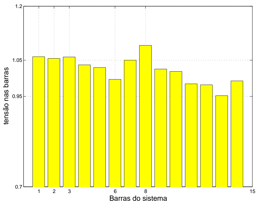
Figura 4.3: Tensão nas barras no cenário S1 - sistema IEEE 14-barras: caso base
