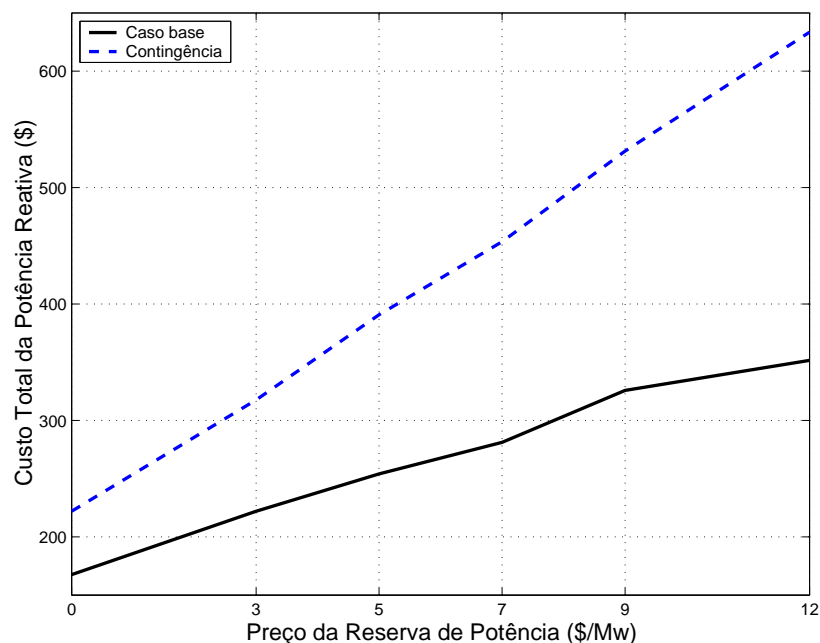
Figura 4.7: Custo total de Potência Reativa no sistema IEEE 14-barras: caso base e contingência
