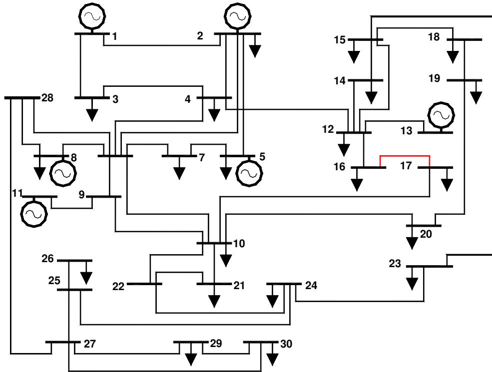
Figura 4.8: Sistema IEEE 30-barras
