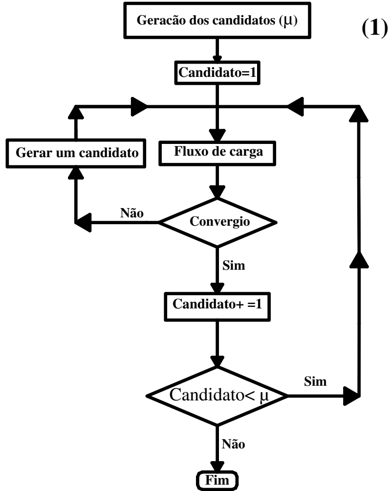
Figura 3.6: Fluxograma para inicializar a população
