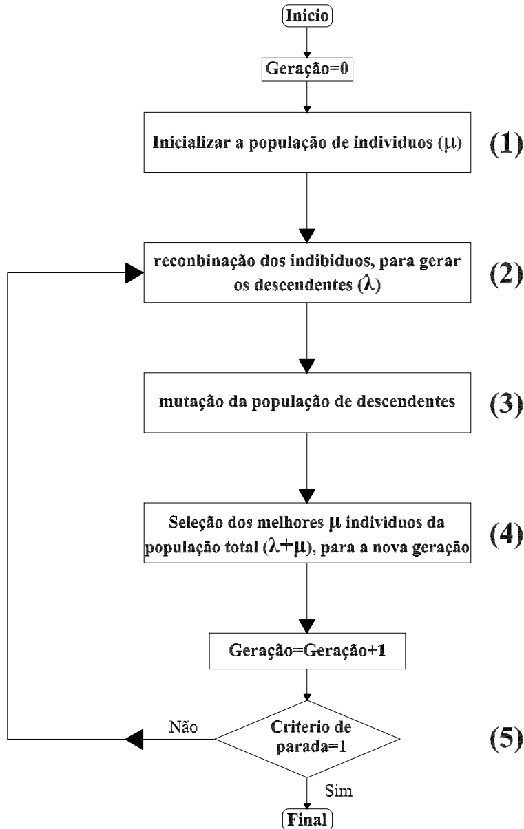
Figura 3.5: Fluxograma do algoritmo proposto
