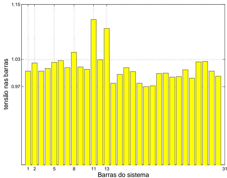
Figura 4.9: Tensão das barras no cenário S1 sistema IEEE 30-barras: caso base
