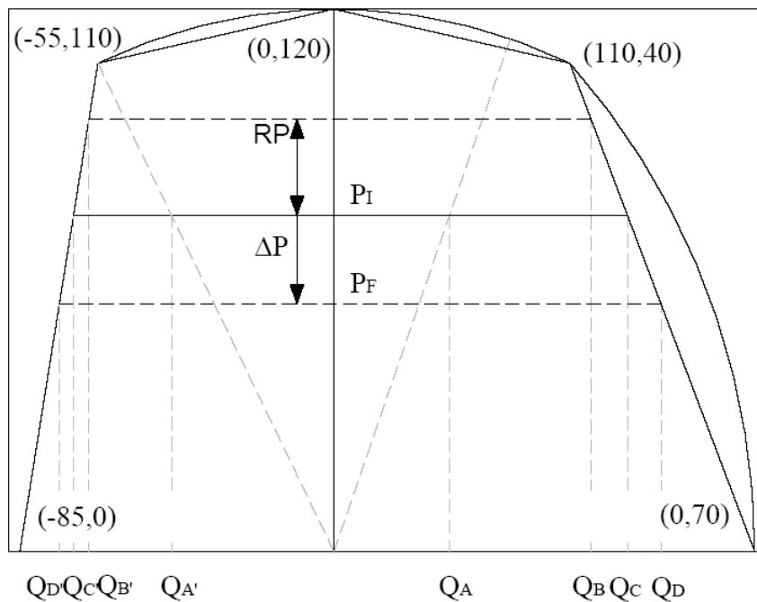
Figura 4.2: Pontos que representam os geradores do sistema IEEE 14-Barras
