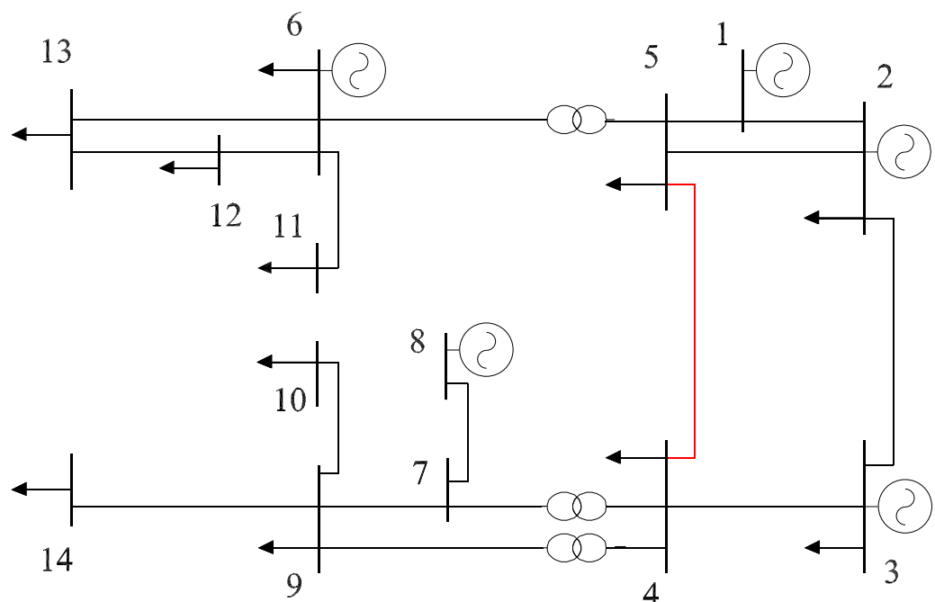
Figura 4.1: Sistema IEEE 14-barras
