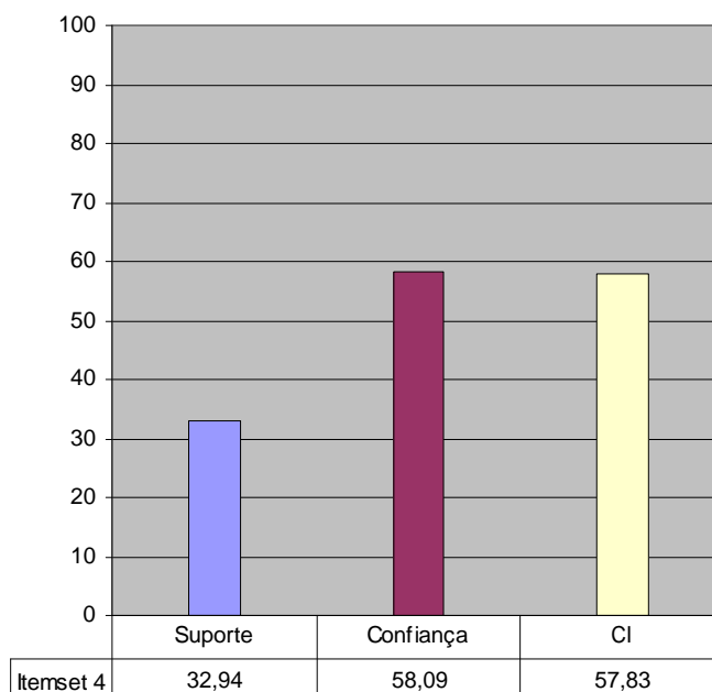
Gráfico 04. Valores de Suporte , Confiança e CI para o itemset 4 .
