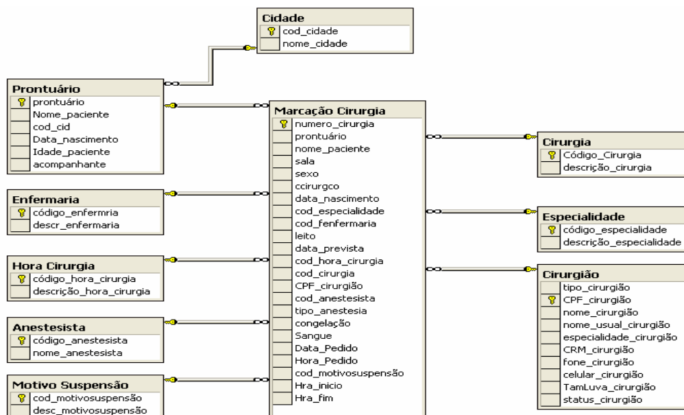
Figura 13. Modelo lógico de dados do centro cirúrgico do HUUFMA.
