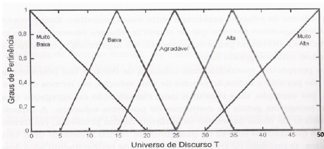
Figura 3. Partição fuzzy de uma variável linguística representando a temperatura.
