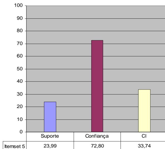
Gráfico 05. Valores de Suporte , Confiança e CI para o itemset 5 .
