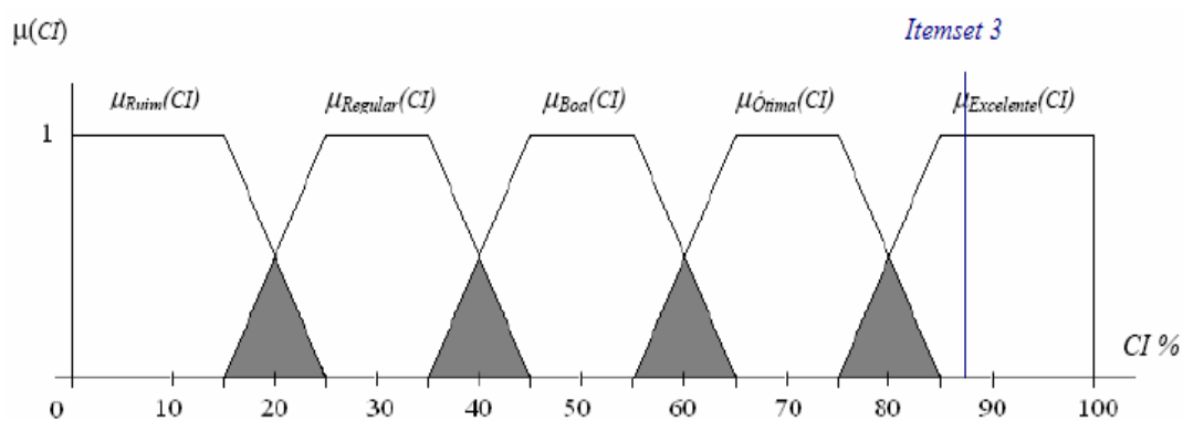
Figura 16. Valor da CI do itemset 3 no conjunto nebuloso da classificação.
