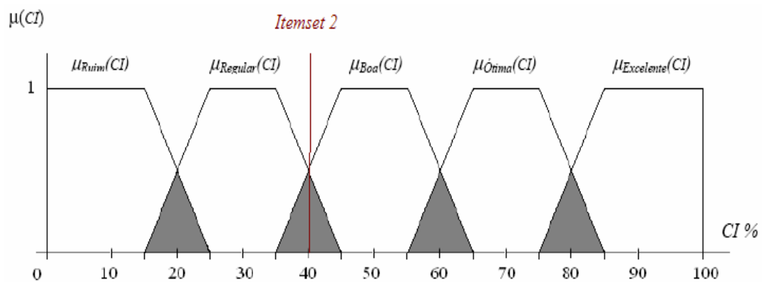
Figura 15. Valor da CI do itemset 2 no conjunto nebuloso da classificação.
