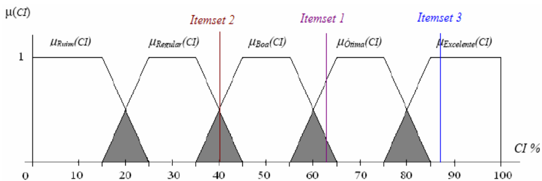
Figura 17. Itemsets 1, 2 e 3 no conjunto nebuloso da classificação.
