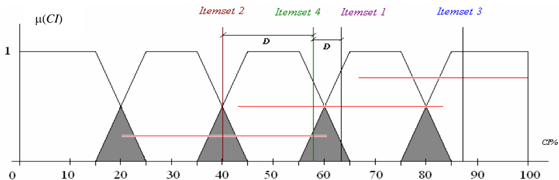
Figura 19. Comparação do itemset 4 com os itemsets 1, 2 e 3 .
