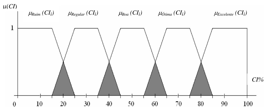
Figura 6. Representação gráfica dos conjuntos nebulosos \mu_{Ruim}(CI_i) , \mu_{Regular}(CI_i) , \mu_{Boa}(CI_i) , \mu_{Ótima}(CI_i) e \mu_{Excelente}(CI_i) .
