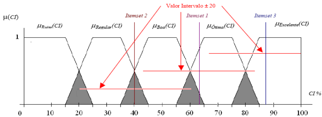
Figura 18. Itemsets 1, 2 e 3 no conjunto nebuloso da classificação e os respectivos intervalos de similaridade.
