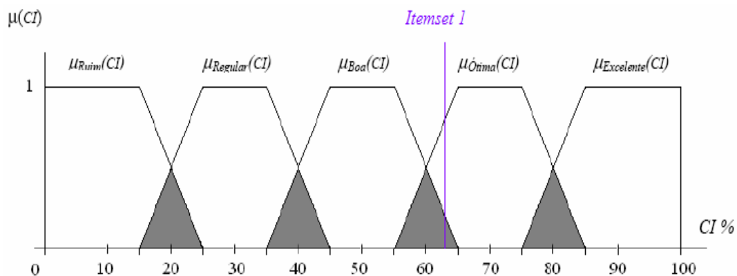
Gráfico 01. Valores de Suporte , Confiança e CI para o itemset 1 .
