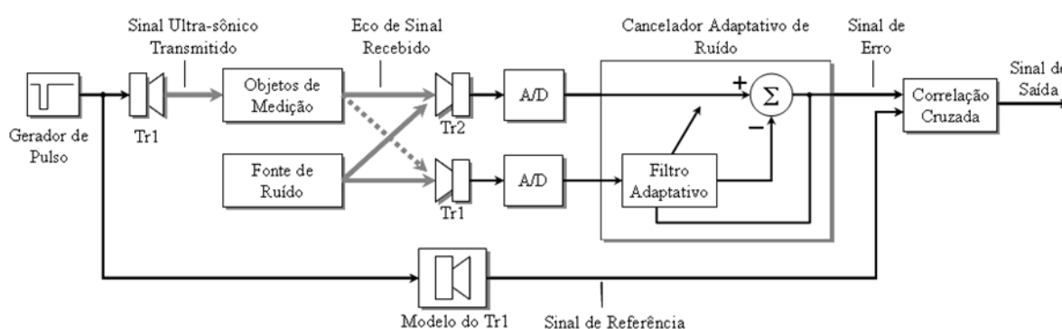
Figura 20 – Sistema de Medição com o uso de Cancelador Adaptativo de Ruído.
