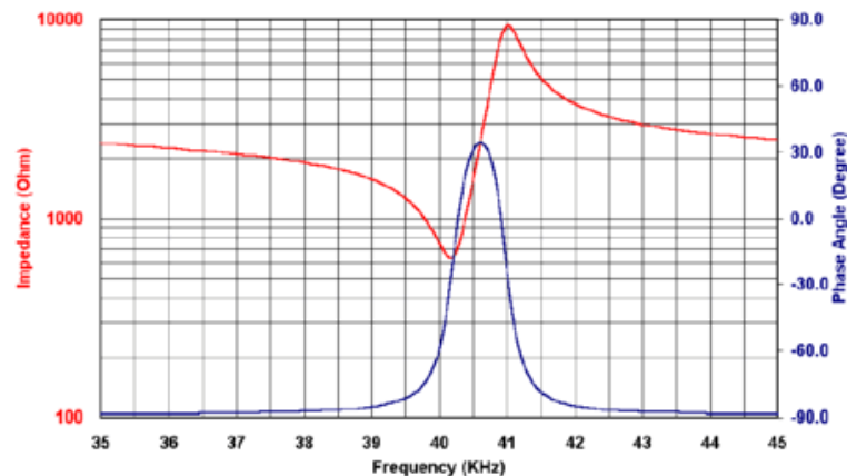
Figura 3 – Comportamento típico da magnitude e da fase de um transdutor ultra-sônico.
