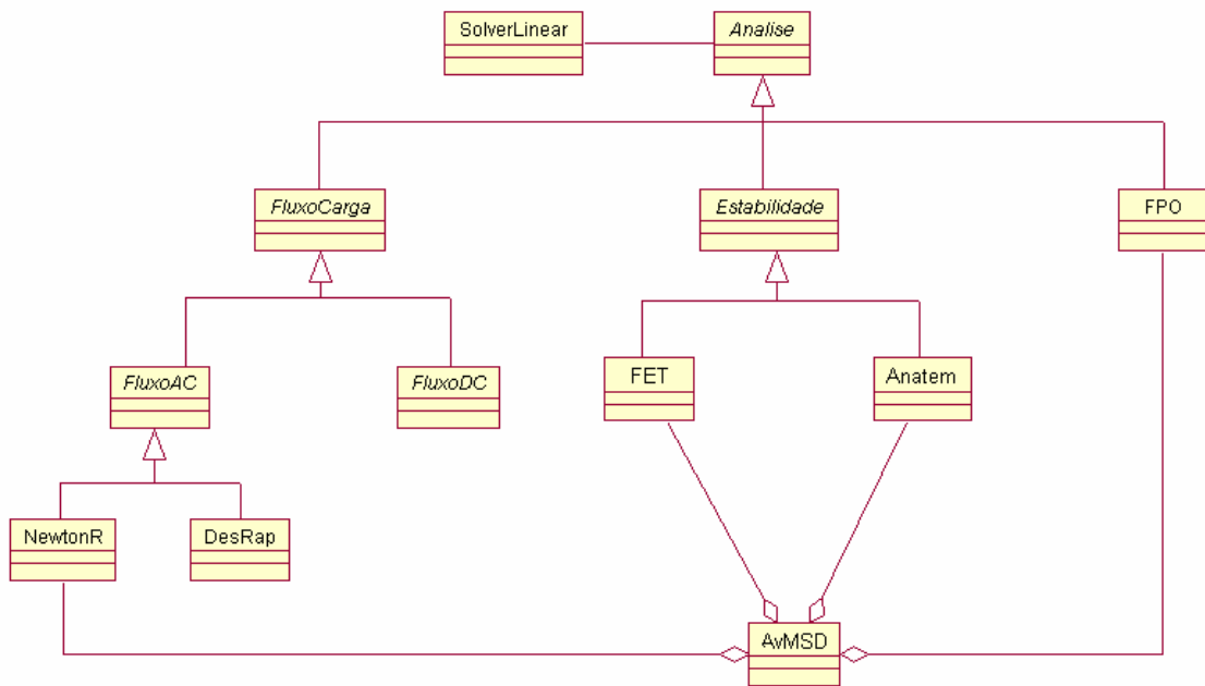
Figura 3.9: Diagrama de classes do componente AnalisesEletricas
