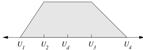
Figura 3.2: Número trapezoidal
