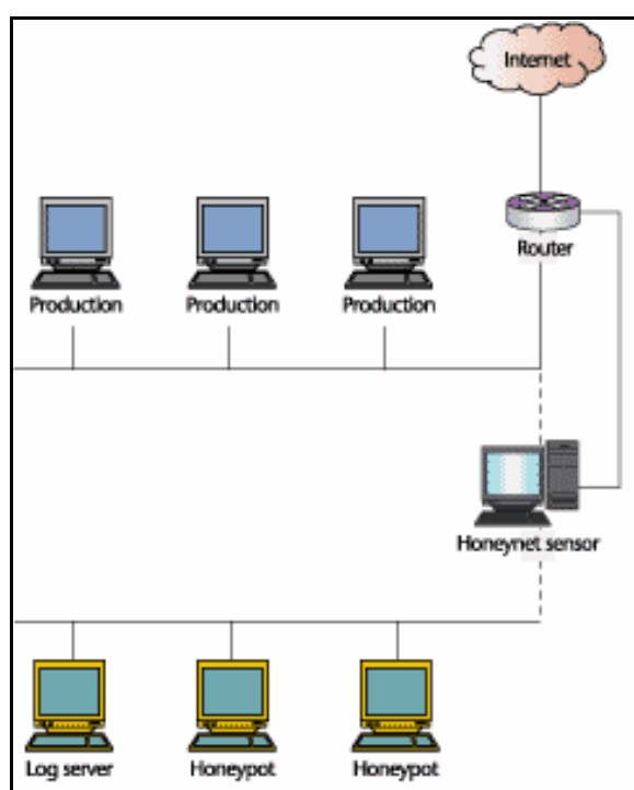
Figura 2.10 – Honeynet Gen II
