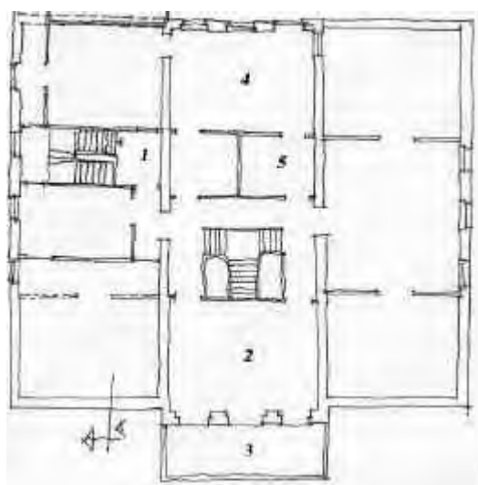
Fig. 76 – SOLAR RODRIGUES MENDES, RECIFE – PE, PLANTA-BAIXA DO PAVIMENTO SUPERIOR.
