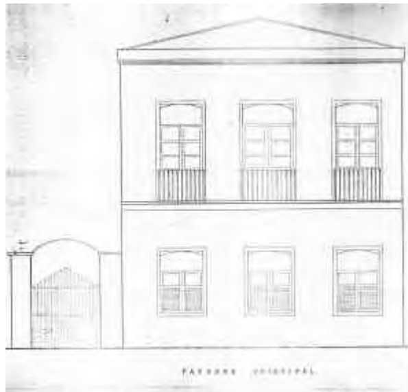
Fig. 104 – CASA 813, RUA OLIVEIRA LIMA, RECIFE – PE, FACHADA FRONTAL. Fachada que dá a frente para o logradouro, de composição simétrica, classicista, onde percebemos o frontão triangular. Os acessos, pela lateral do terreno, para onde se volta a residência, é uma implantação típica da segunda metade do século XIX. (Crédito da Ilustração: cópia de planta encontrada na mapoteca do IPHAN – 5ª. Superintendência Regional).
