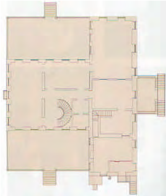
Fig. 122– CASA 1893, AV. 17 de AGOSTO, RECIFE – PE, PLANTA BAIXA DO PAVIMENTO TÉRREO.
