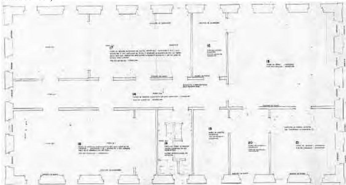
Fig.114–CASA 150,RUA BENFICA, RECIFE-PE, PLANTA-BAIXA PAVIMENTO SUPERIOR. Planta-baixa do pavimento superior da residência, onde vemos a circulação central de distribuição dos cômodos e grande sala frontal, provavelmente o salão de visitas da residência. Os banheiros, tanto deste pavimento quanto do pavimento térreo, são de construção recente. (Crédito da Ilustração: Foto da Autora, datada de 2002).
