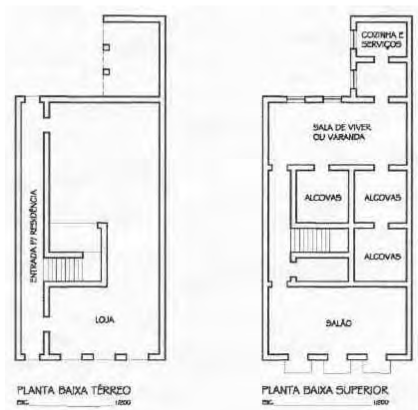
Fig. 1 – PLANTAS DO SOBRADO TÍPICO COLONIAL BRASILEIRO.
